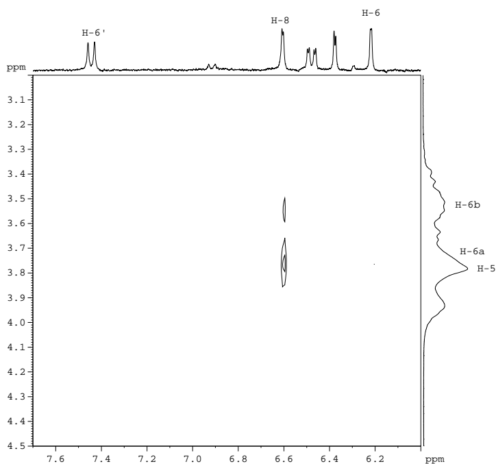
Figura 3.2.14 Sección del espectro ROESY del complejo M-HP \beta CD.
