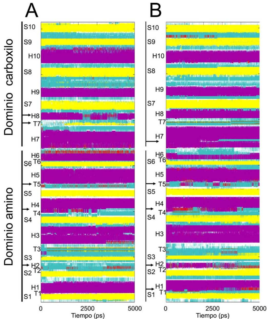
Figura 5. Comportamiento temporal de la estructura secundaria de simulaciones a 300 K. Panel A. PaFtsZ, Panel B. MjFtsZ. Los colores representan distintos elementos de estructura secundaria, calculados con STRIDE: morado: hélices \alpha ; amarillo: hebras \beta ; verde: vueltas \beta ; rojo: hélices \pi .
