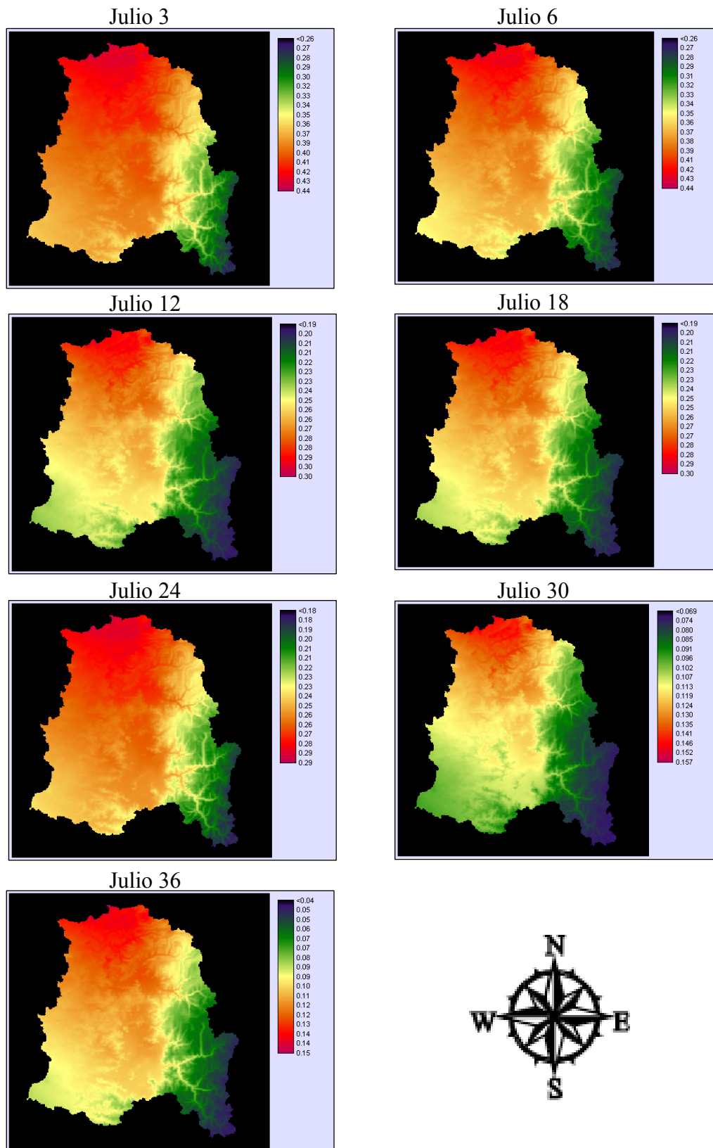
Figura 13. Imágenes de la sequía meteorológica. Probabilidades de no excedencia asociada a precipitación igual o menor al 70% de la media. Mes de inicio Julio.
