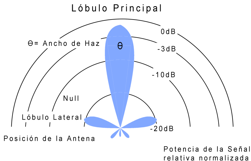
Figura 2.1: Patrón de radiación de una antena estándar.
