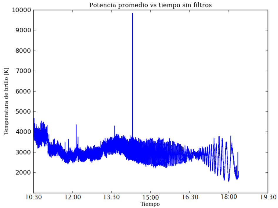
Figura 4.19: Evolución temporal de la potencia promedio del espectro medido. Medición obtenida por el interferómetro en un seguimiento al sol.
