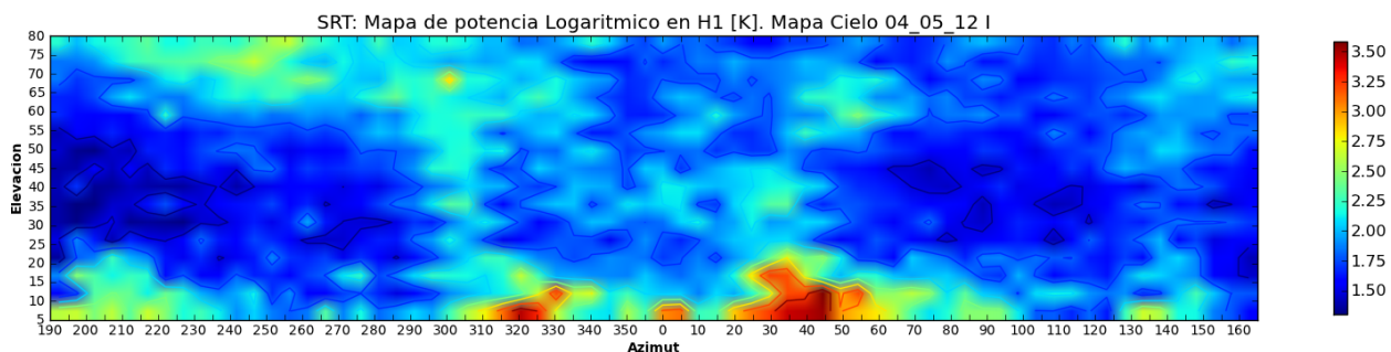
Figura 6.1: Mapa de potencia logarítmico antena poniente.
