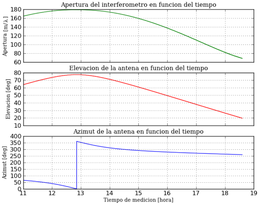
Figura 4.21: Evolución de la apertura, azimut y elevación del interferómetro en función del tiempo [UTC-4].
