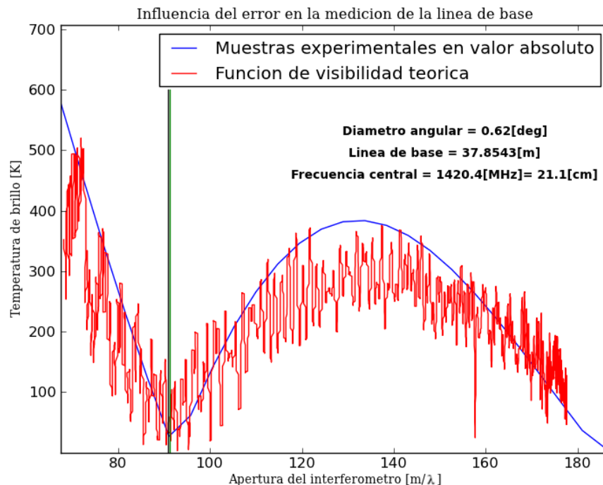
Figura 4.25: Rango de error en la determinación del punto de inflexión para muestras experimentales.
