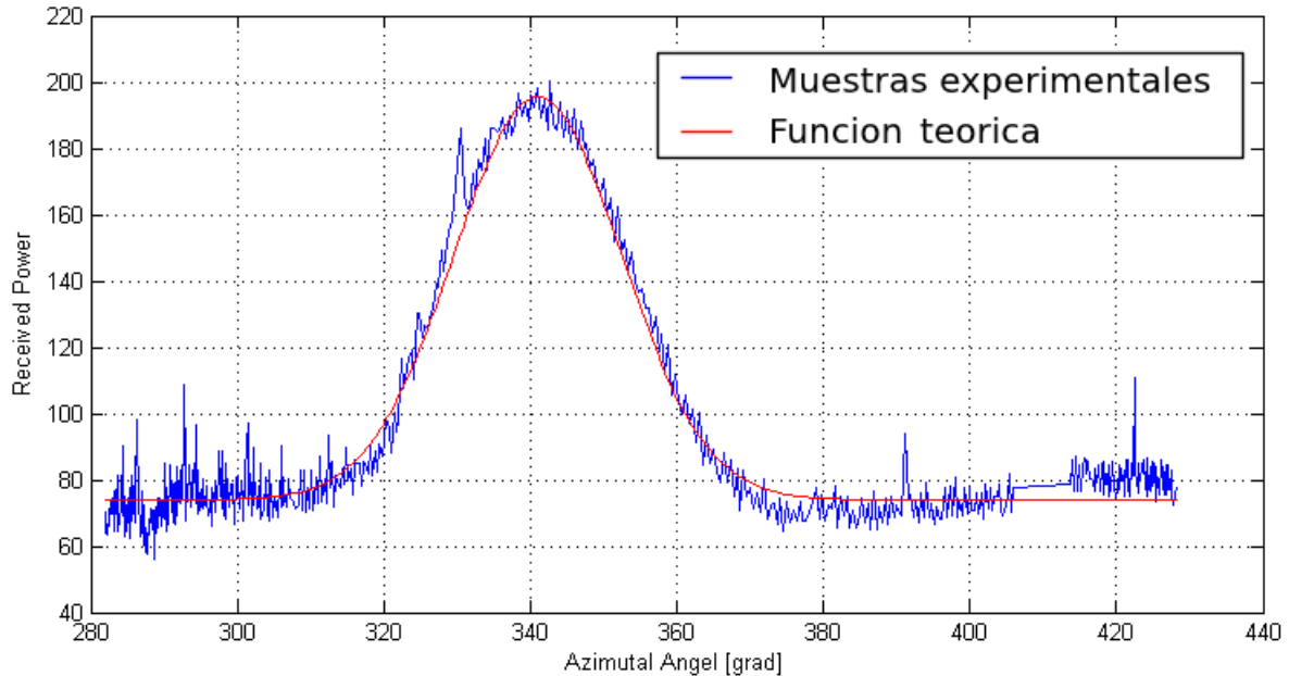
Figura 6.2: Potencia promedio en función del ángulo azimutal [12].
