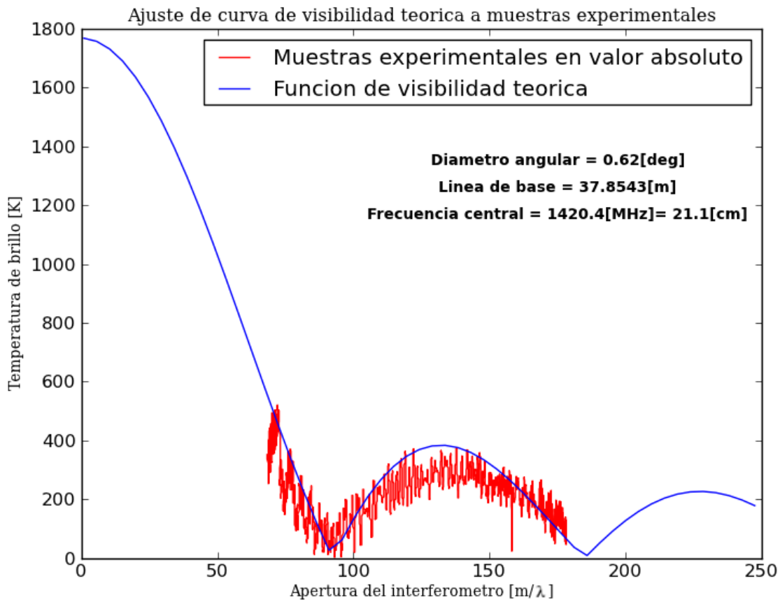
Figura 6.6: Ajuste de función de visibilidad V con los datos de potencia promedio en valor absoluto, en función de la apertura del interferómetro.
