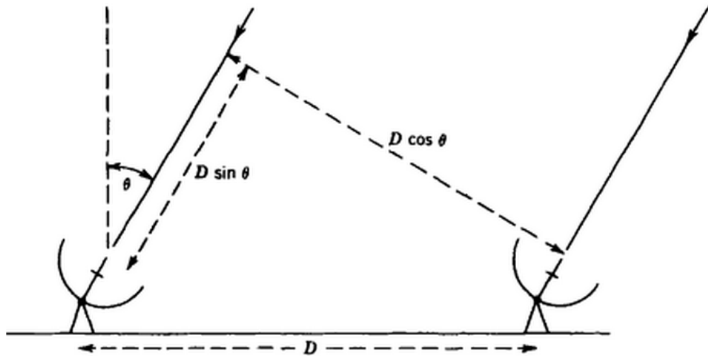
Figura 4.18: Geometría de un interferómetro elemental [8].
