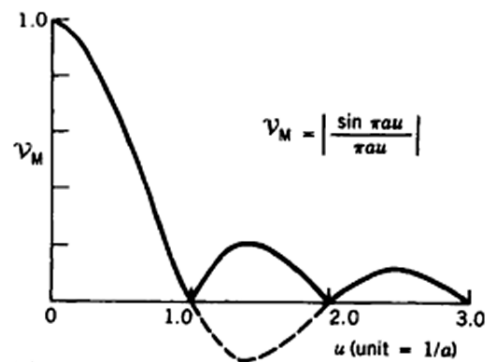
Figura 4.17: Gráfico de la función de visibilidad [8].
