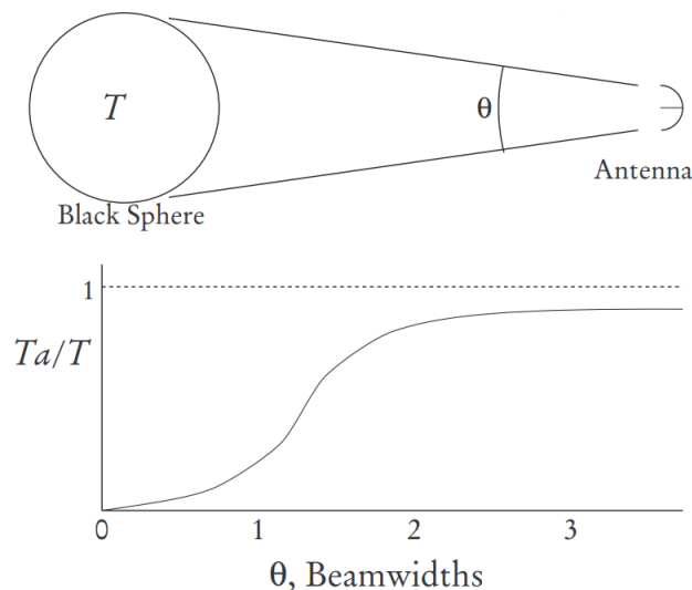
Figura 2.2: Factor de dilución de haz. Corresponde a la razón entre la temperatura recibida T_a sobre la temperatura de la fuente T , en función del diámetro angular de una fuente circular. Este diámetro está medido en anchos de haz de la antena [5].
