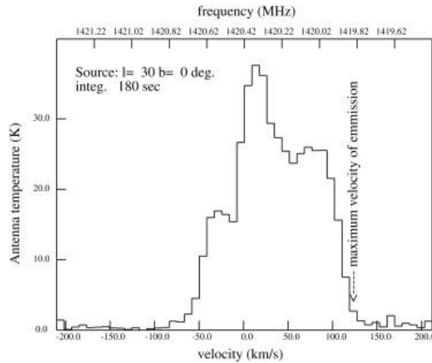
Figura 5.3: Espectro acumulado ejemplo para longitud l = 30 [16].
