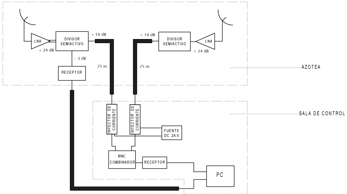
Figura 4.14: Diagrama de bloques de la interconexión para la obtención de las primeras franjas interferométricas.
