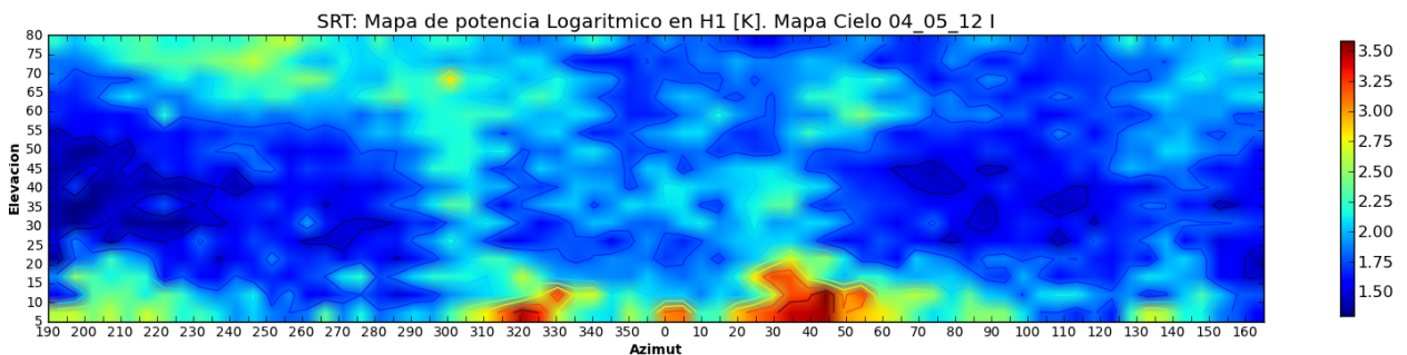
Figura 3.2: Mapa de potencia logarítmico antena poniente.
