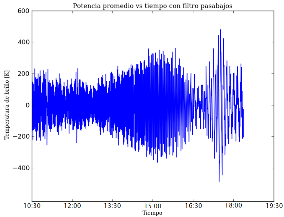
Figura 4.20: Evolución temporal de la potencia promedio del espectro medido, después de aplicar un filtro pasabanda. Medición obtenida por el interferómetro en un seguimiento al sol.
