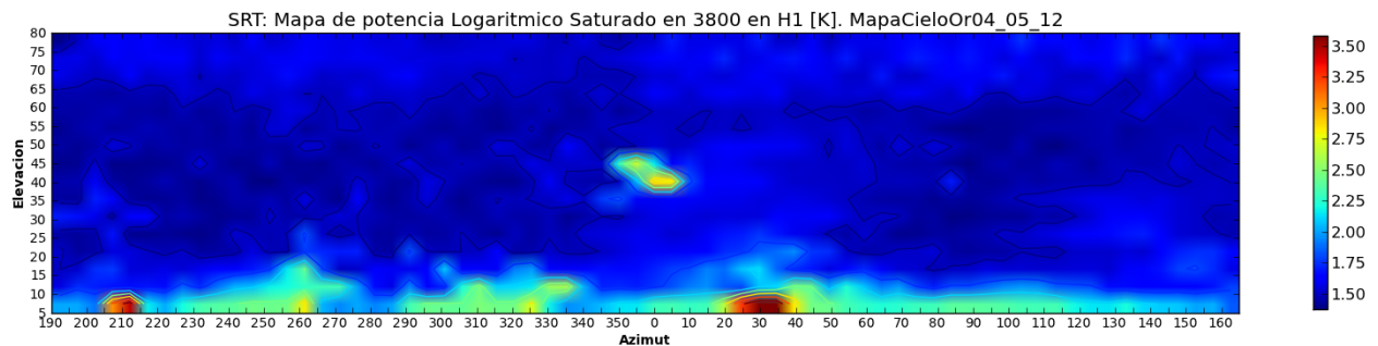
Figura 3.1: Mapa de potencia logarítmico saturado antena oriente.
