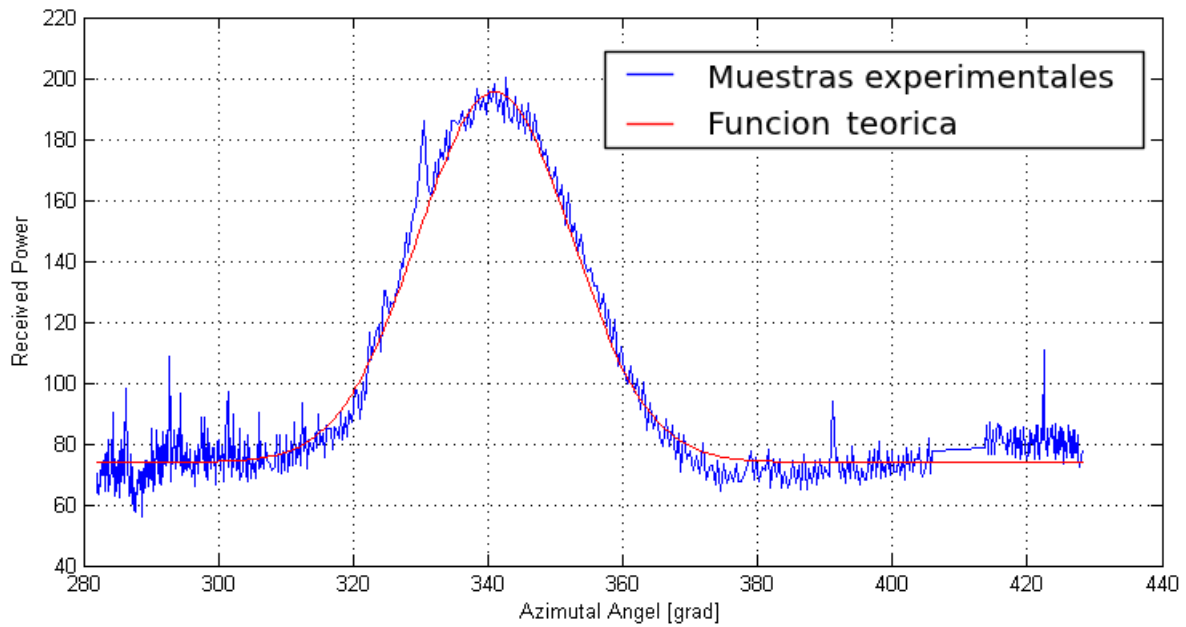
Figura 3.5: Potencia promedio en función del ángulo azimutal [12].
