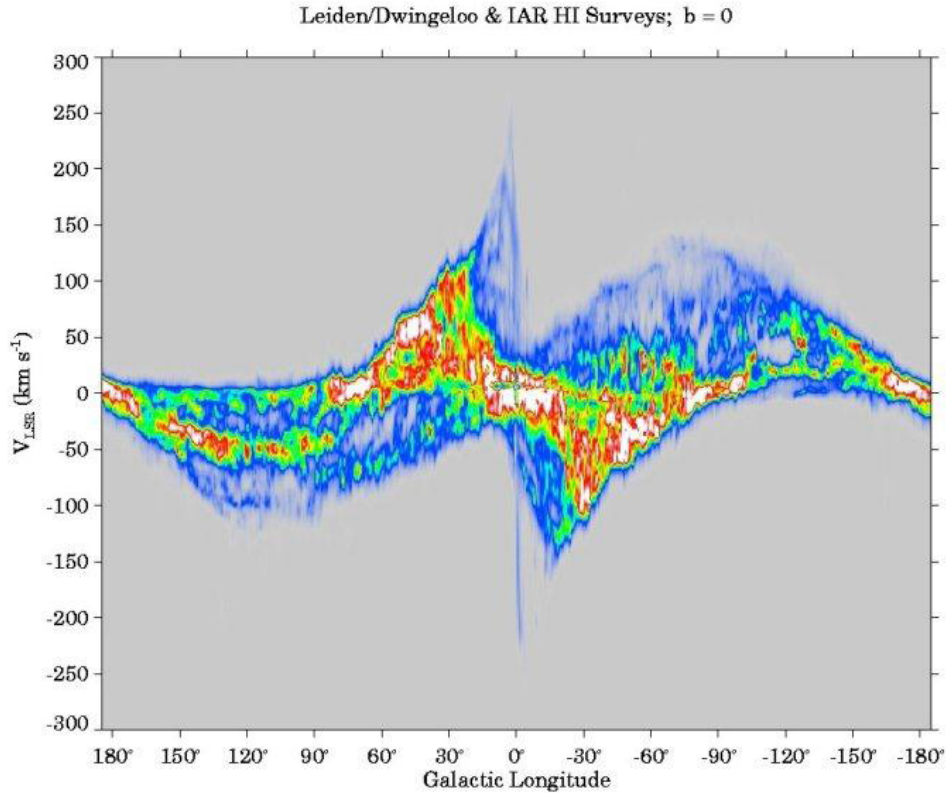
Figura 5.4: Hidrógeno neutro a través del plano galáctico [13].
