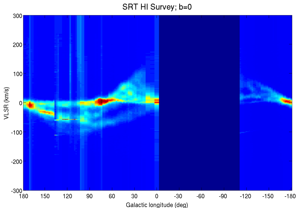
Figura 5.5: Hidrógeno neutro a través del plano galáctico medido desde un SRT [13].
