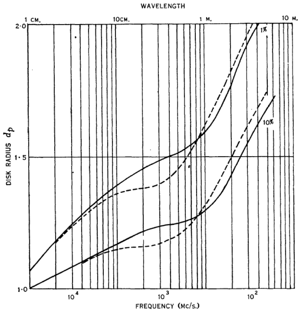
Figura 4.26: Variación del radio del disco solar respecto de la frecuencia. El radio, d_p (en unidades de R_0 ), del disco está especificado por la razón de la temperatura efectiva en el extremo y: (a) la temperatura aparente (línea continua), (b) temperatura máxima efectiva (línea punteada) [21].
