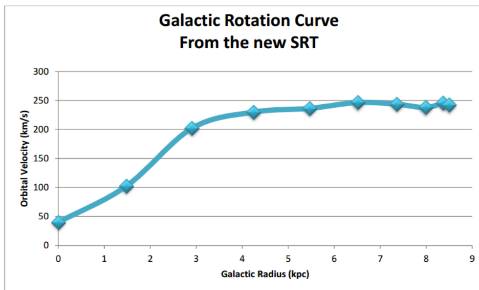
Figura 5.1: Curva de rotación galáctica tomada con el nuevo SRT en el MIT [13].
