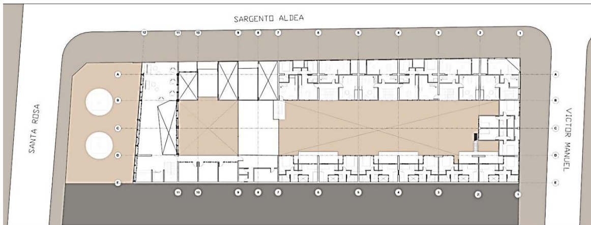
Planta tercer nivel
