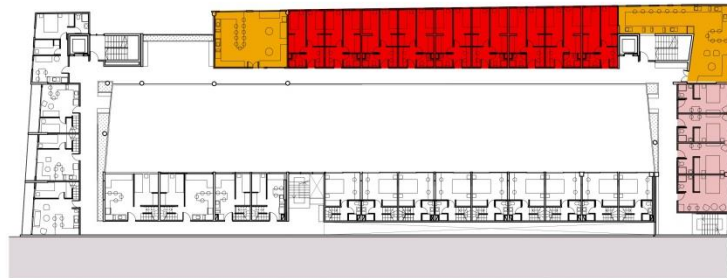
PLANTA 3 PISO
