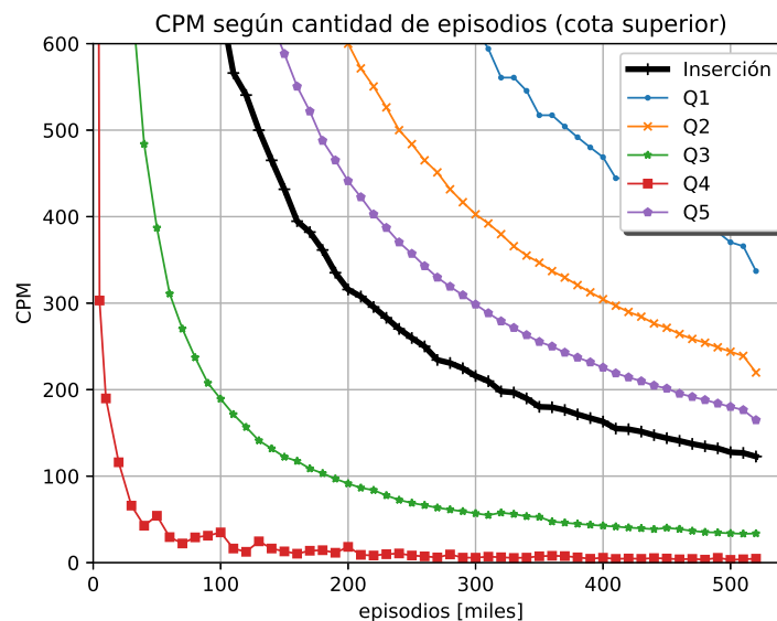
Figura 6.3: El gráfico muestra la cota superior para las CPM posibles para cada operación según la cantidad de episodios almacenados en la base de datos.
