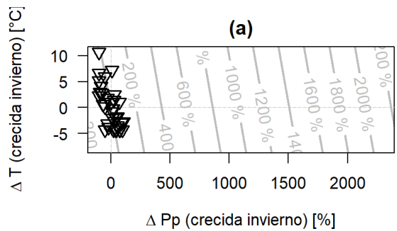
Figura-D 16: variaciones de caudal máximo [-] para temporada de invierno (a) y temporada de invierno (b). Cuenca 5710001
