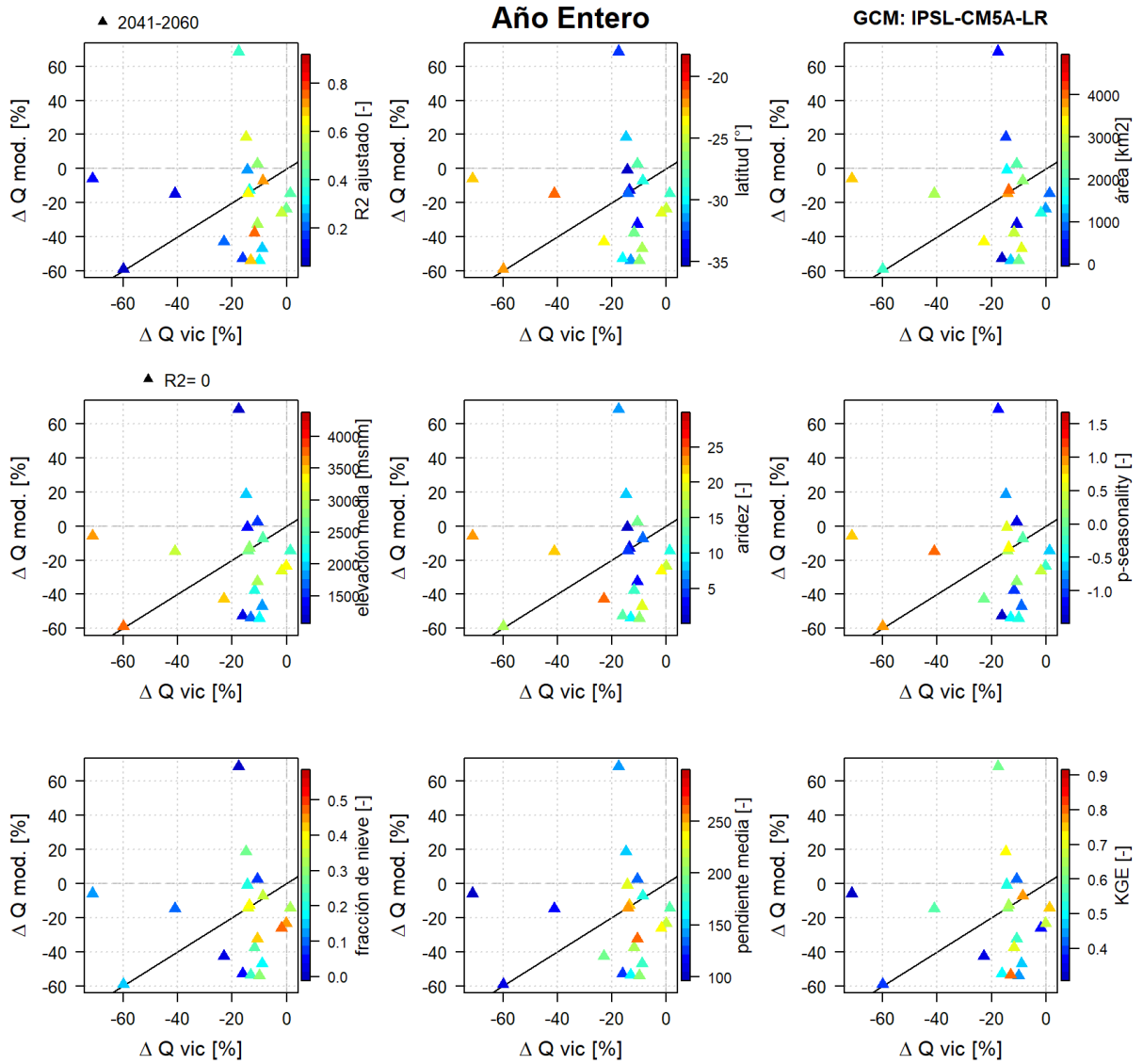
Figura C- 16: Comparación de variaciones de caudales VIC y caudales MOD en Año Entero junto a estadísticos y características de las cuencas para IPSL-CM5A-LR. Periodo 2040-2059.
