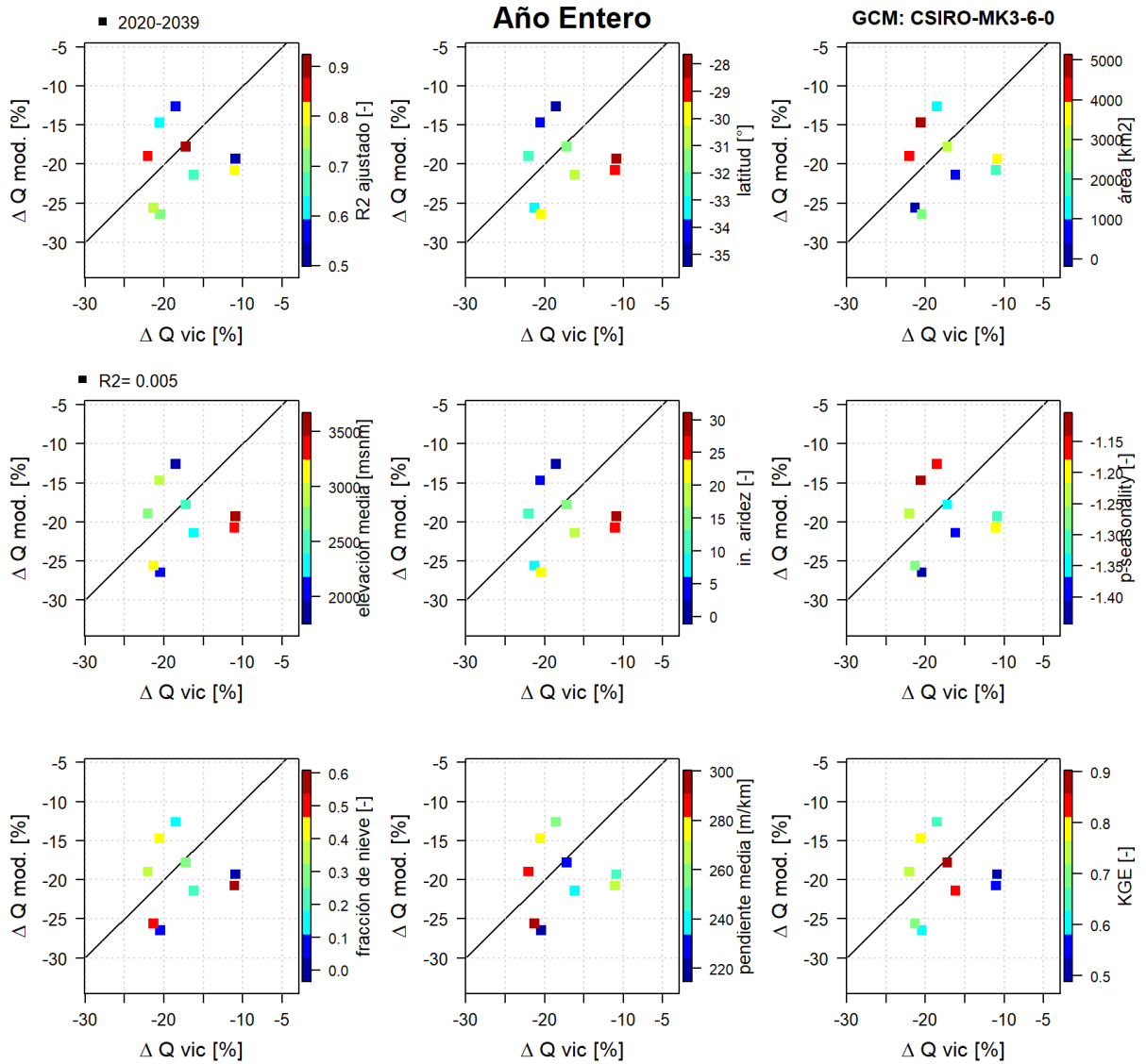
Figura C- 27: Comparación de variaciones de caudales VIC y caudales MOD en Año Entero junto a estadísticos característicos de las cuencas para GCM CSIRO-MK3-6-0 para error absoluto menor a 10%. Período 2020-2039.
