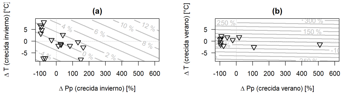
Figura-D 6: variaciones de caudal máximo [-] para temporada de invierno (a) y temporada de invierno (b). Cuenca 4313001
