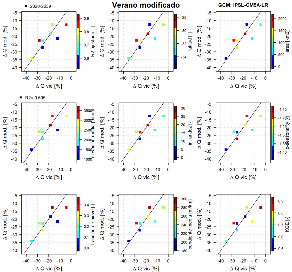
Figura C- 37: Comparación de variaciones de caudales VIC y caudales MOD en Verano Modificad junto a estadísticos y características de las cuencas para GCM IPSL-CM5A-LR para error absoluto menor a 10%. Período 2020-2039.
