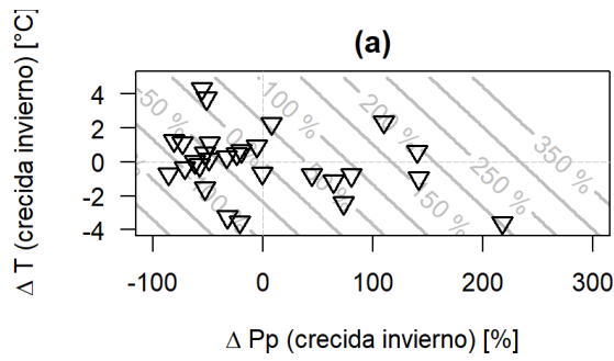
Figura-D 13: variaciones de caudal máximo [-] para temporada de invierno (a) y temporada de invierno (b). Cuenca 5101001
