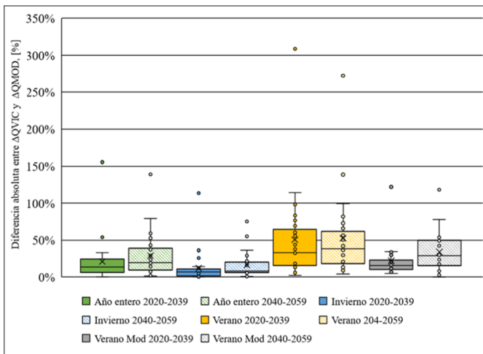
Figura 5. 17: Distribuciones de diferencias absolutas entre variaciones \Delta QVIC y \Delta QMOD para distintas temporadas para dos periodos futuros para GCM MIROC-ESM.
