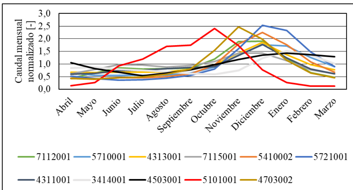
Figura 3. 5: Caudales medios mensuales normalizados de cuencas con en régimen Nival entre los años 1985 y 2015.
