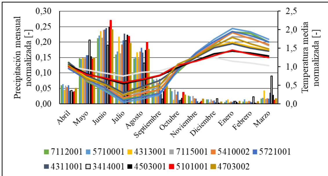
Figura 3. 4: Climogramas de cuencas con régimen Nival entre los años 1985 y 2015.
