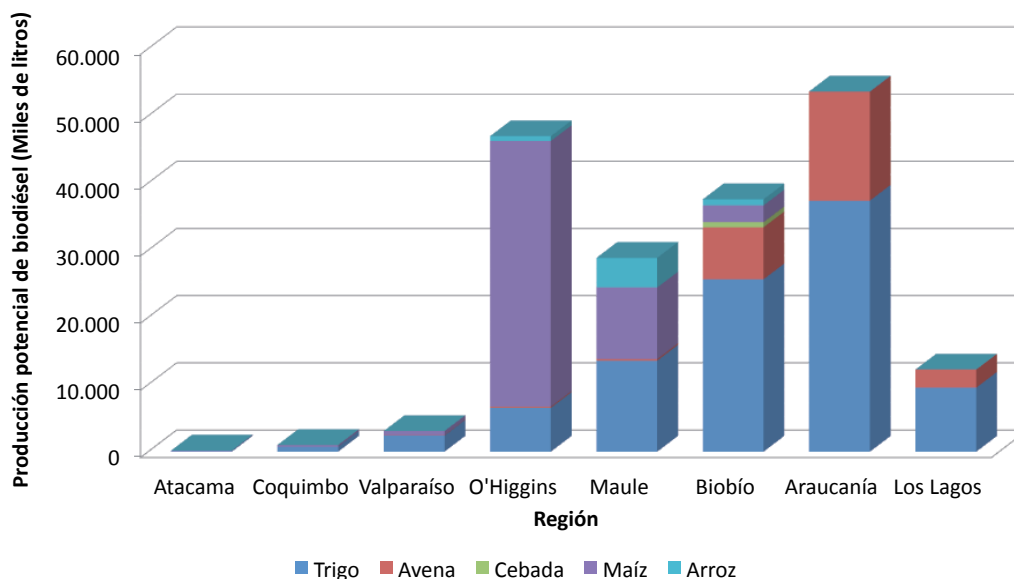
Figura 15. Producción de biodiésel (miles de litros) entre las regiones de Atacama y Los Lagos empleando los residuos agrícolas de trigo, avena, cebada, maíz y arroz.
