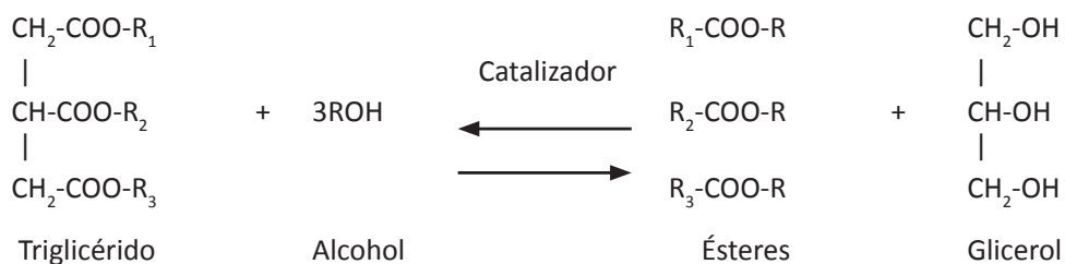
Figura 8. Transesterificación de triglicéridos (Srivastava y Prasad, 2000; Demirbas, 2008; Demirbas, 2009b).
