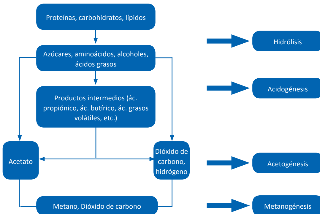
Figura 12. Proceso de conversión anaeróbica de la materia orgánica (Demirbas, 2009a).
