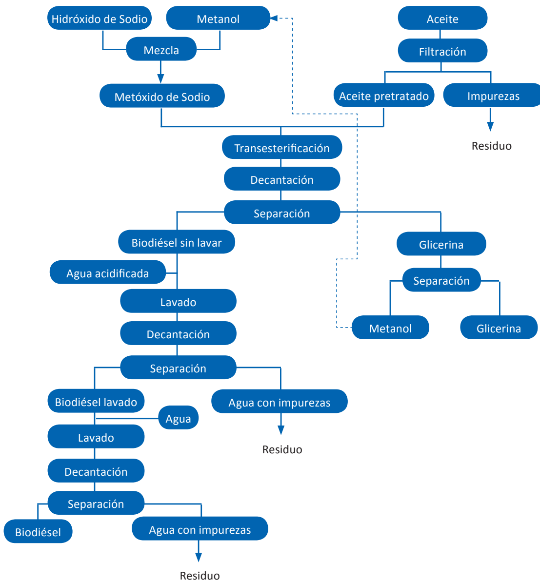
Figura 10. Esquema general para la obtención de biodiésel (Fuenzalida, 2008).
