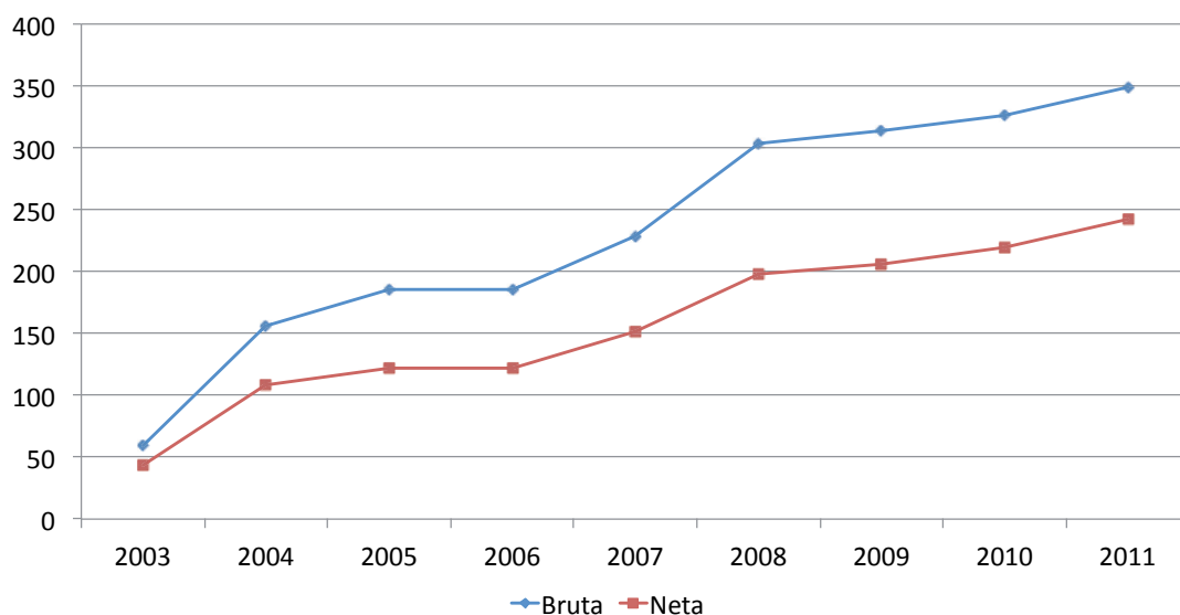
Figura 16. Potencia Bruta y Neta (MW) de Unidades generadoras Sistema Interconectado Central de Chile, en base a Biomasa o biomasa-petróleo acumulada años 2003 a 2011 (CNE, 2011b).
