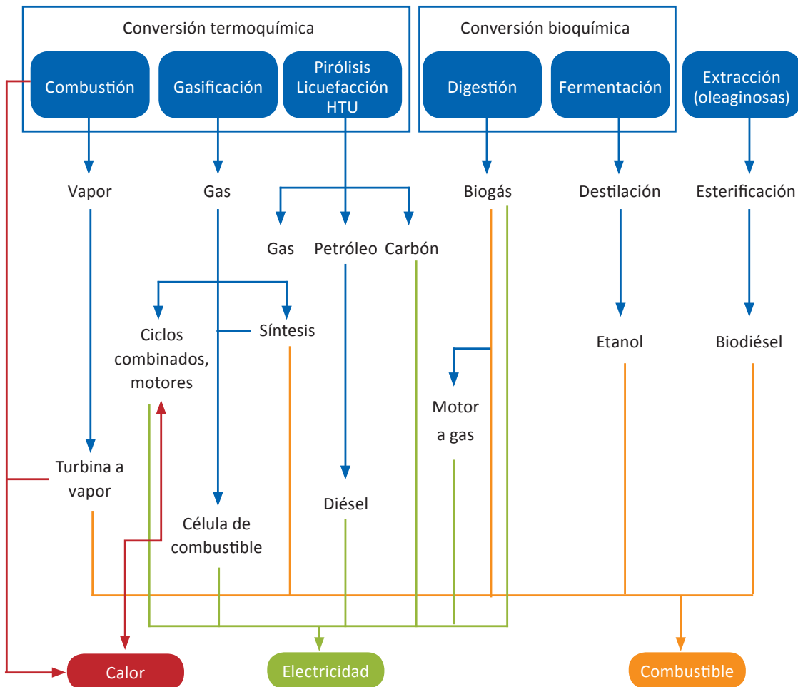
Figura 1. Vías tecnológicas para la producción de bioenergía (Turkenburg et al., 1998; BNDES y CGEE, 2008).
