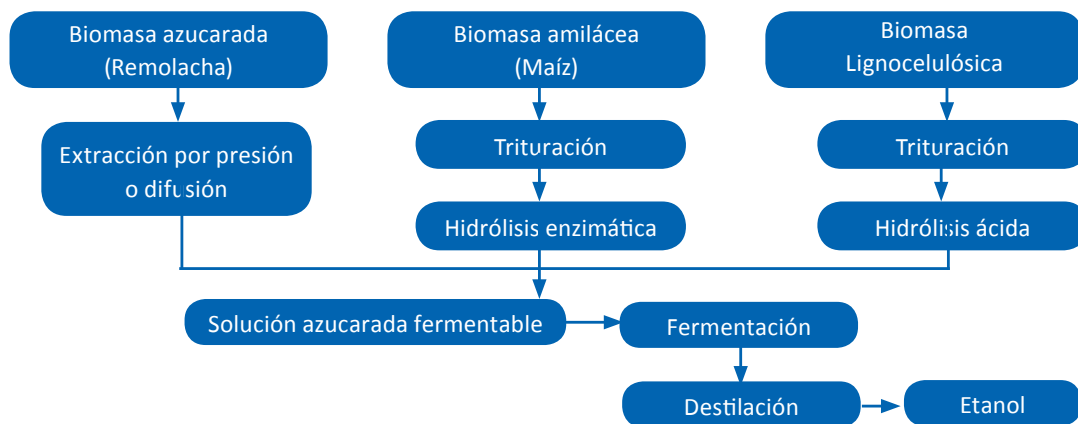
Figura 6. Rutas tecnológicas para la producción de bioetanol (BNDES y CGEE, 2008).
