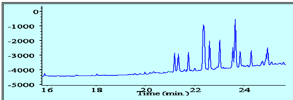
Figura 4.1-Cromatograma del estándar de LAS-butilado 2000 [mg L -1 ].
