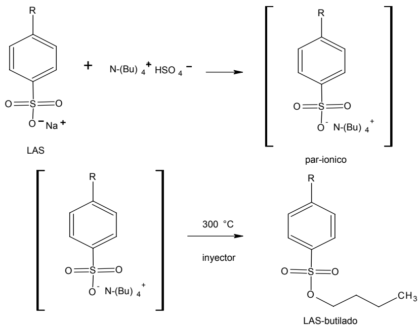
Figura 1.3-Reacción de derivatización, pirólisis del tetraalquilamonio (TAA).
