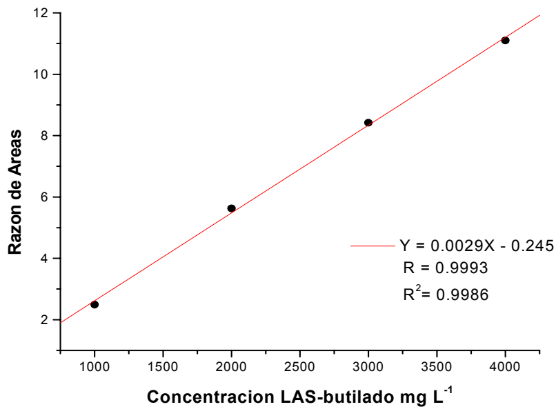
Figura 4.16-Curva de calibración rango 1000-4000 [mg L -1 ]
