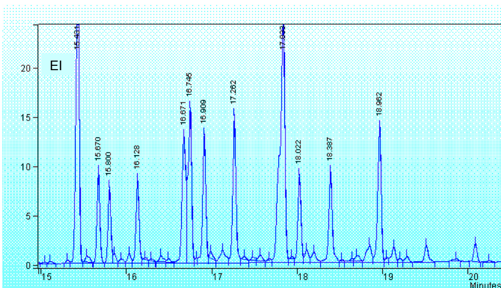
Figura 4.17-Cromatograma del estándar de LAS-butilado 2000 [ \text{mg L}^{-1} ], utilizando metodología y condiciones cromatográficas optimizadas GC-FID.
