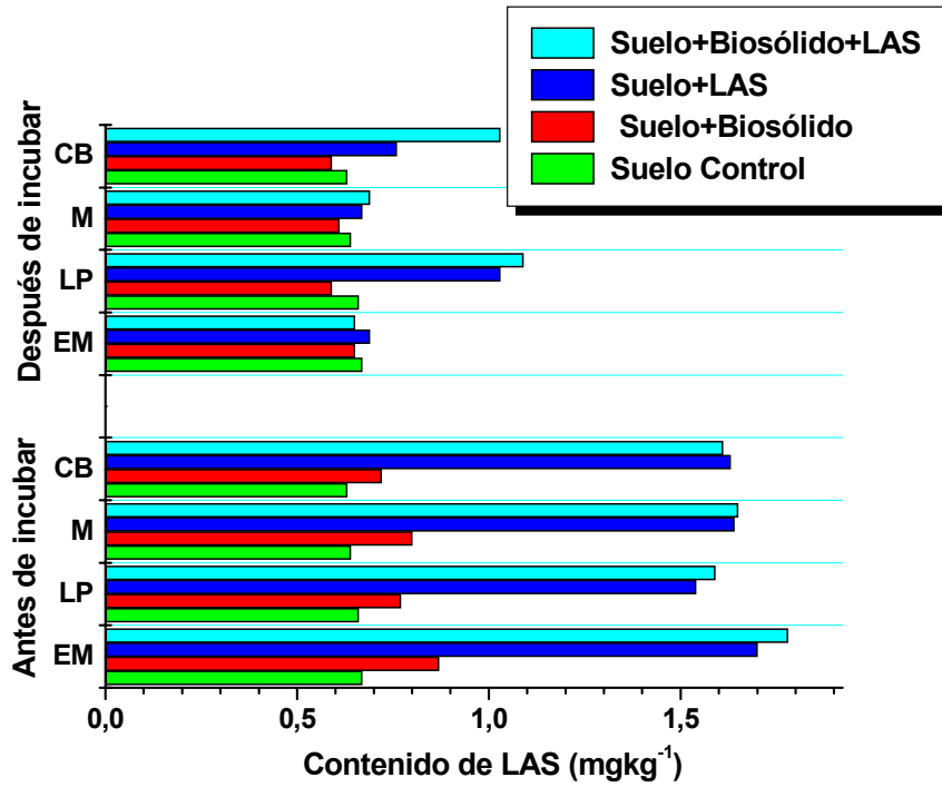
Figura 4.19-Contenido de LAS en los suelos Control, tratados con BET2005 y LAS, antes y después del tratamiento de incubación por 30 días en condiciones controladas de temperatura y capacidad de campo.
