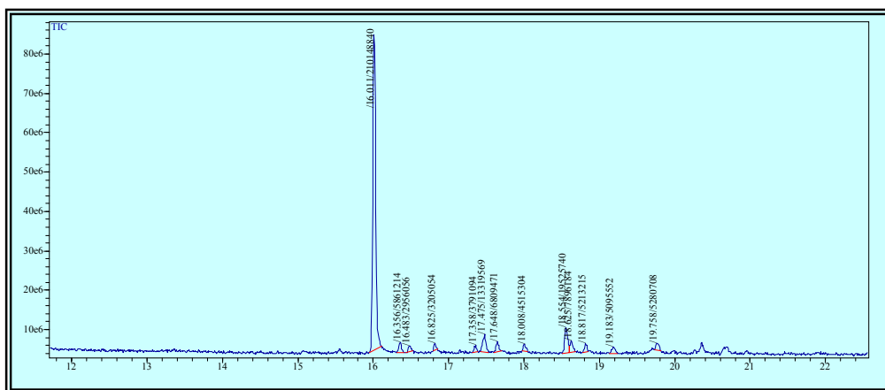
Figura 4.2-Cromatograma de una muestra de biosólido BET2005, empleando extracción acuosa y derivatización, mediante GC-MS.
