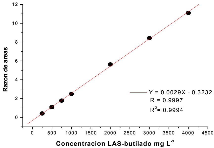
Figura 4.14-Curva de calibración rango 250-4000 [mg L -1 ]
