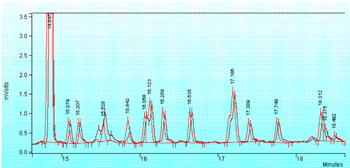
Figura 4.21-Cromatograma del suelo, La Paloma (LP), enriquecido con 1,0 \text{ g kg}^{-1} de LAS ; — 0 días ; — 30 días.
