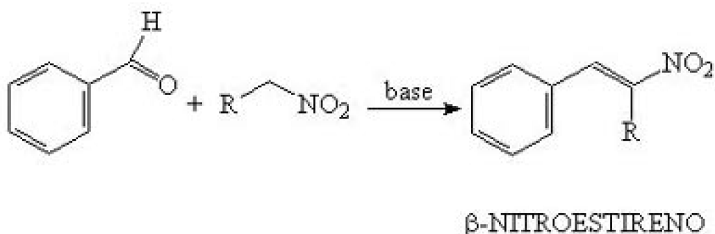
Figura 6: Reacción para la obtención de \beta -nitroestirenos
