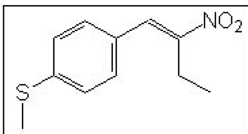
( Z )-1-(4-metiltiofenil)-2-nitrobuteno (20)
