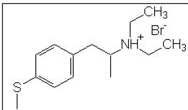
(±)-1-(4-Metiltiofenil)-2-( N -alilamino)-propano (NAMTA) (15)
