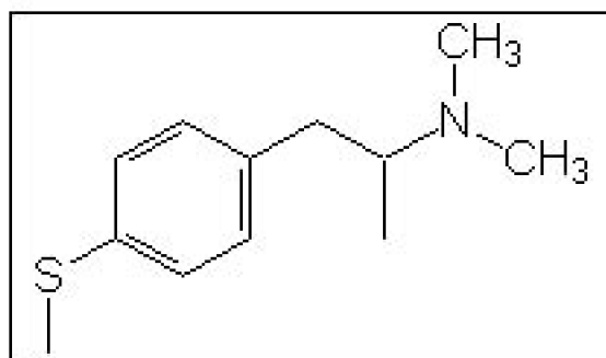
(±)-1-(4-Metiltiofenil)-2-(N,N-dimetilamino)-propano(clorhidrato) (DMMTA · HCl)
