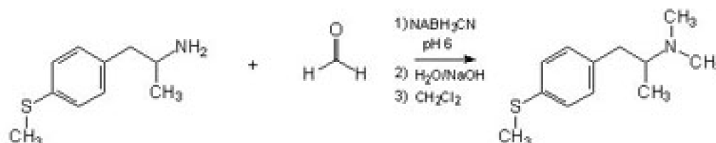
Figura 12: Ruta sintética para la obtención de DMMTA
