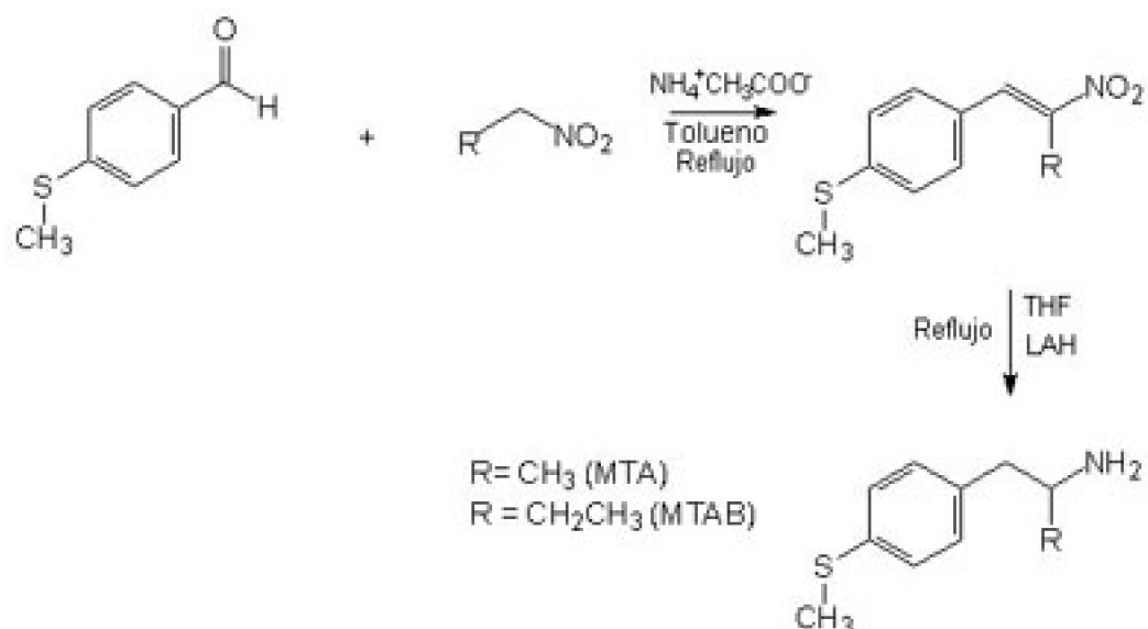
Figura 7: Ruta sintética para la obtención de MTA y MTAB
