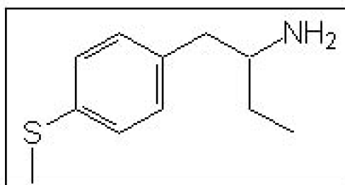
(±)-1-(4-Metiltiofenil)-2-aminobutano (clorhidrato) (MTAB + HCl) (22)
