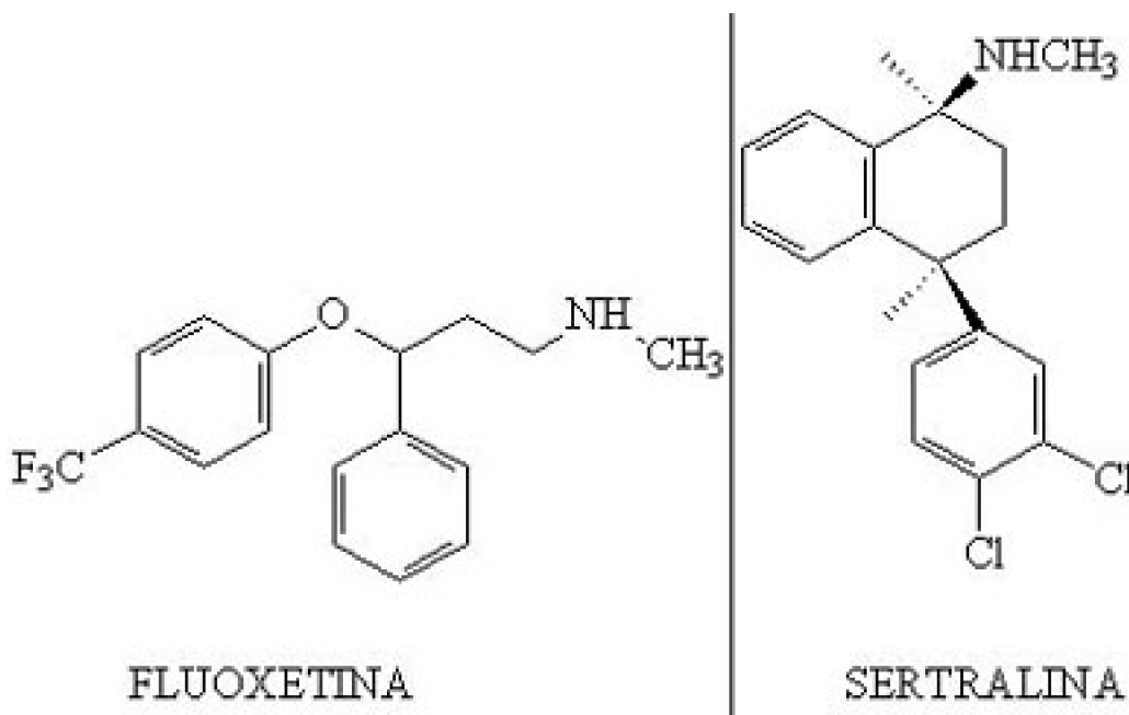
Figura 4: Estructuras químicas de fluoxetina y sertralina
