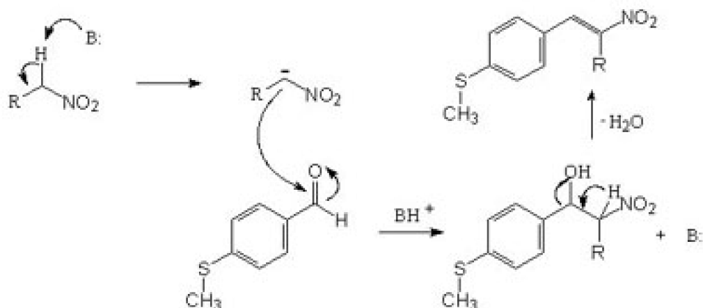
Figura 8: Mecanismo de la reacción de síntesis de \alpha -nitroestirenos
