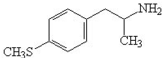
4-metiltioanfetamina (MTA)
