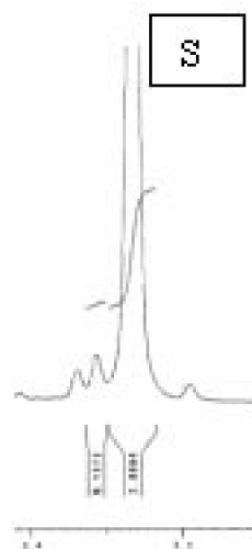
Figura 16.- Señales de ^1\text{H} -RMN correspondientes a los metoxilos en las amidas de Mosher y configuración absoluta de las aminas.
