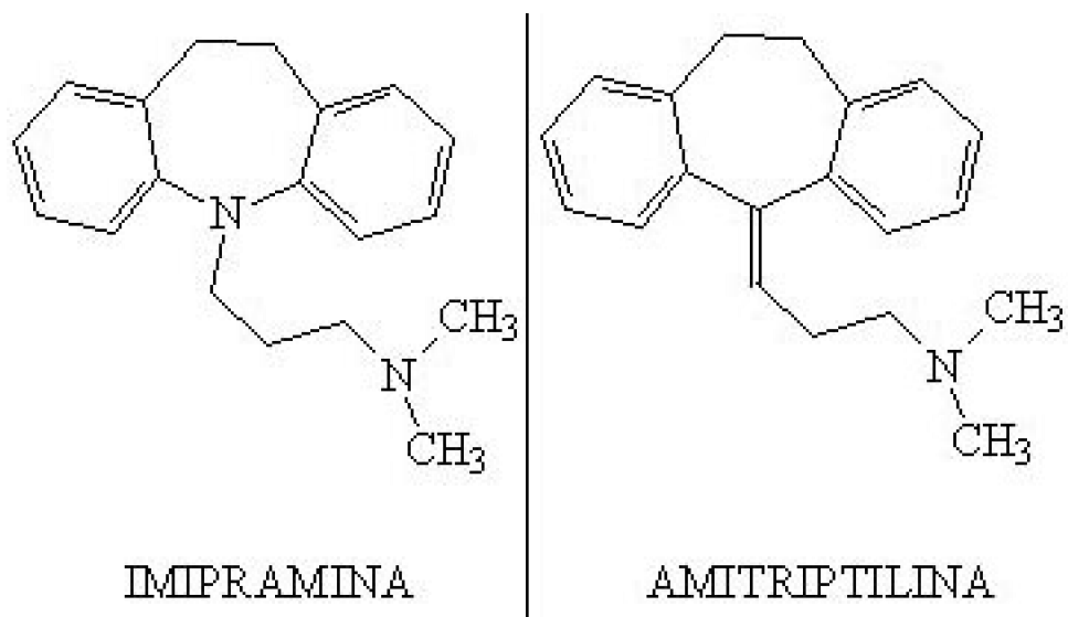
Figura 2: Estructuras químicas de imipramina y amitriptilina
