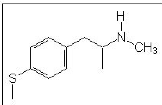
(±)-1-(4-Metiltiofenil)-2-(N-metilamino)-propano (clorhidrato) (NMMTA · HCl) (7)
