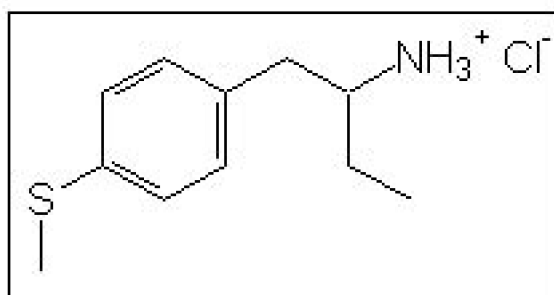
(±)-1-(4-Metiltiofenil)-2-aminobutano (clorhidrato) (MTAB + HCl) (22)
