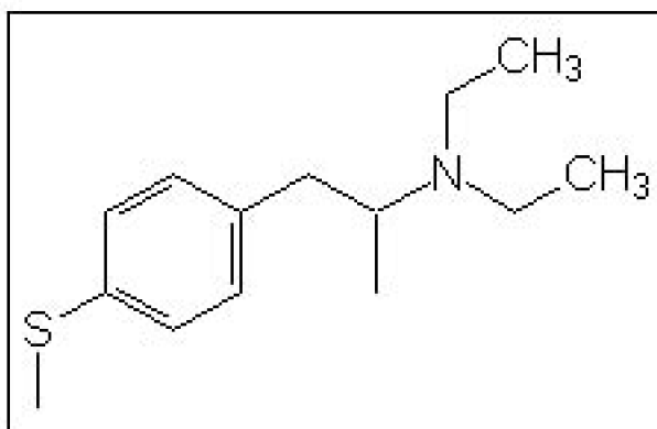
(±)-1-(4-Metiltiofenil)- 2-( N,N -dietilamino)-propano (bromhidrato) (DEMTA · HBr) (14)
