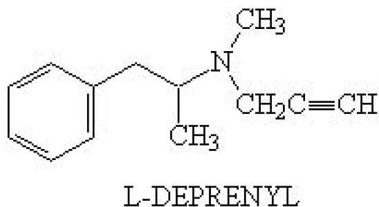
Figura 5: Estructura química de L-deprenyl
