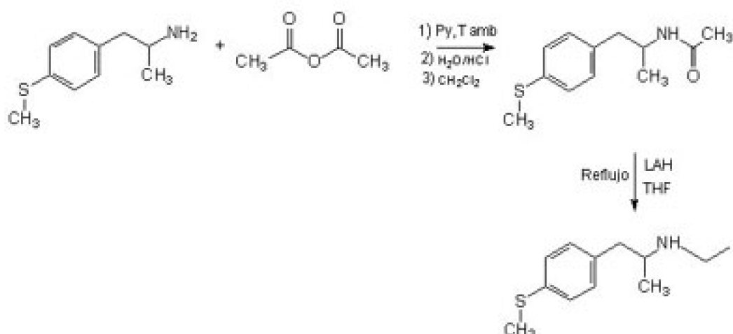
Figura 13: Ruta sintética para la obtención de NEMTA
