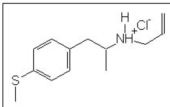
(±)-1-(4-Metiltiofenil)-2-( N,N -dialilamino)-propano (clorhidrato) (DAMTA · HCl) (18)
