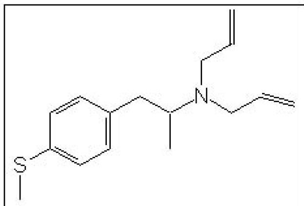
(±)-1-(4-Metiltiofenil)-2-( N -alilamino)-propano (clorhidrato) (NAMTA · HCl) (17)
