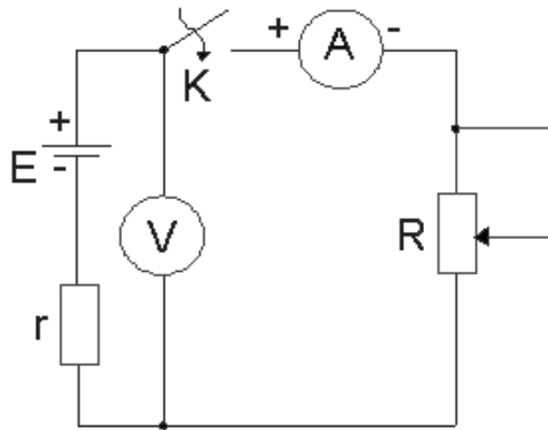
Fig. 7. Circuito Eléctrico. http://www.uib.es/depart/gte/edutec-e/revelec16/leon.htm [Consulta: 10/10/2010]
