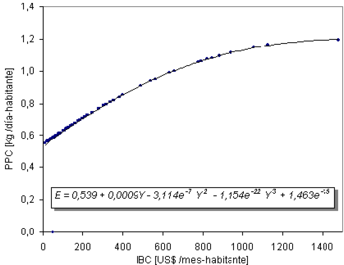
Figura N° : Curva polinómica de Kuznets Ambiental
