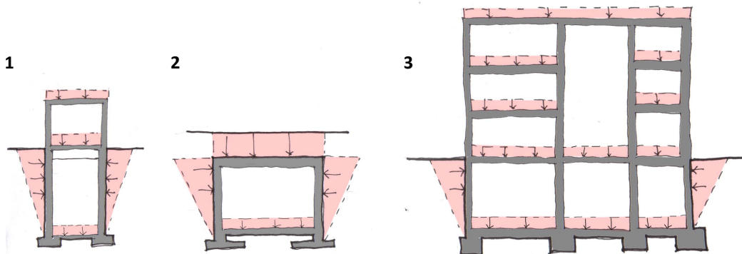
Cargas estructurales en Cortes tipo: 1. Acceso, 2. Salas, 3. Investigación. Fuente: Elaboración propia
