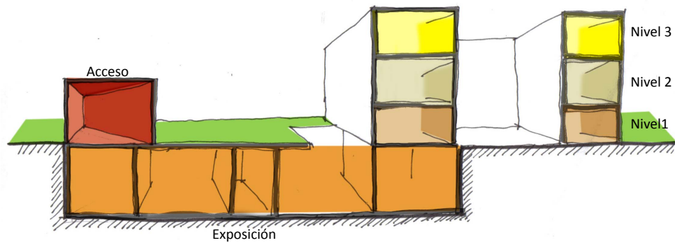
Corte esquemático
