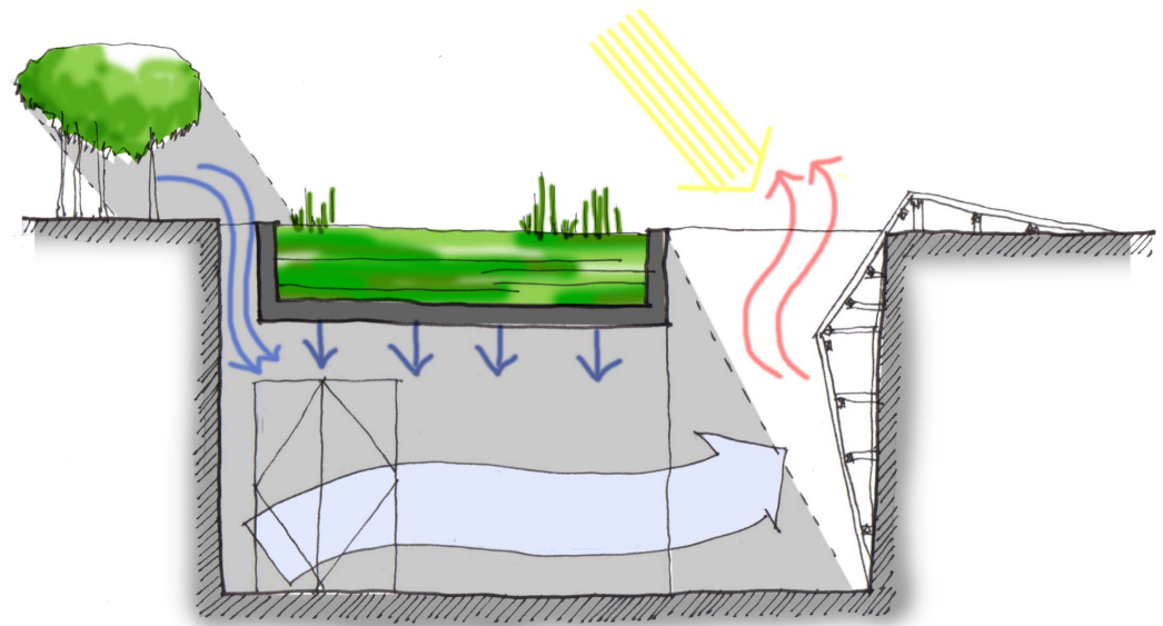
Esquema circulación de aire y enfriamiento por métodos pasivos en recintos subterráneos. Fuente: Elaboración propia.
