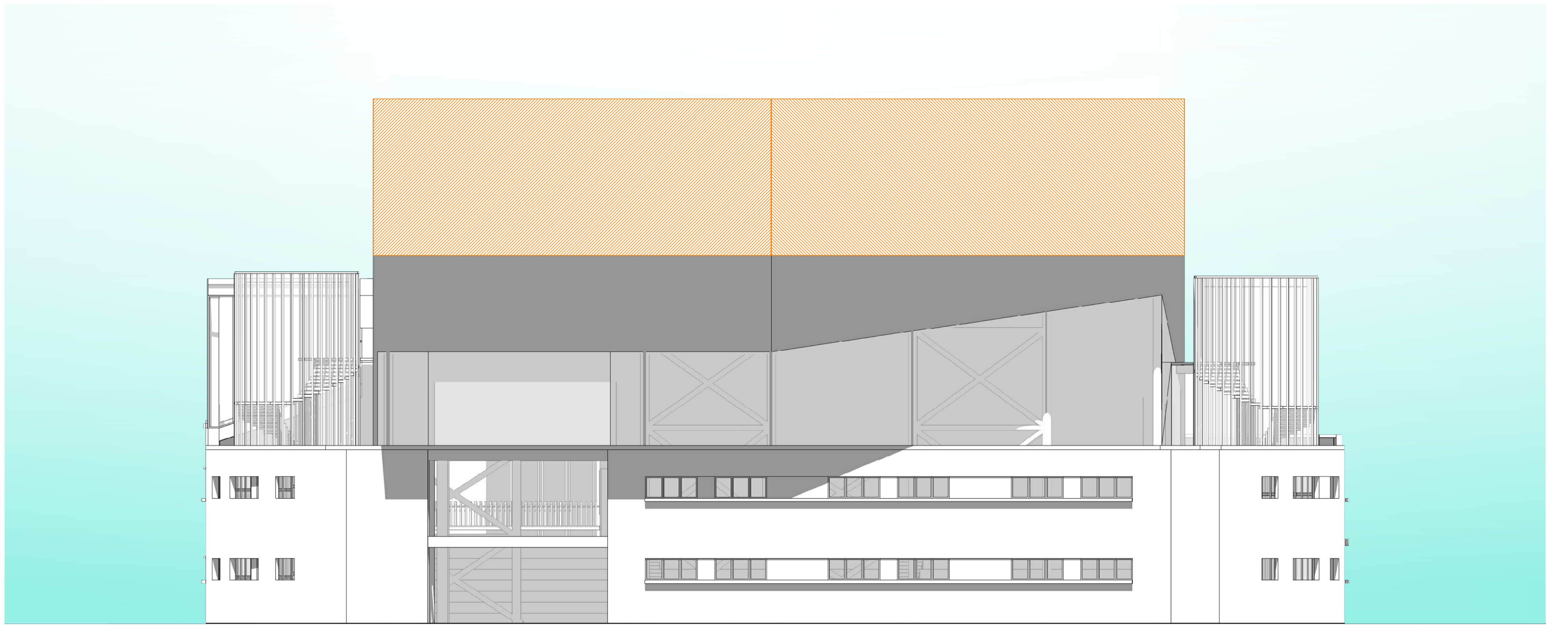
Elevación Norte Escala 1:125
