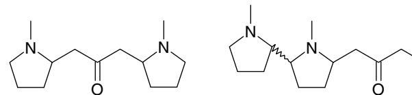
Cuscohygrine
