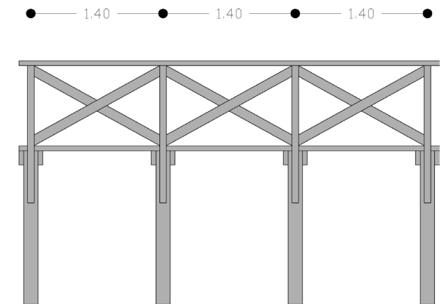
Elevaciones modelo de pasarela Esquema de Maria Paz Hargreaves intervenido por el autor
