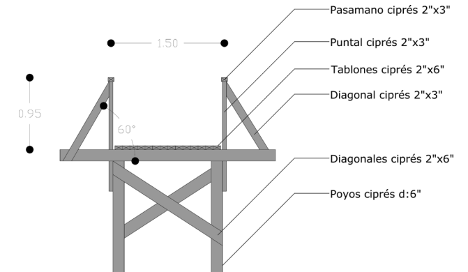
Escantillón Envaralado Esquema de Maria Paz Hargreaves intervenido por el autor
