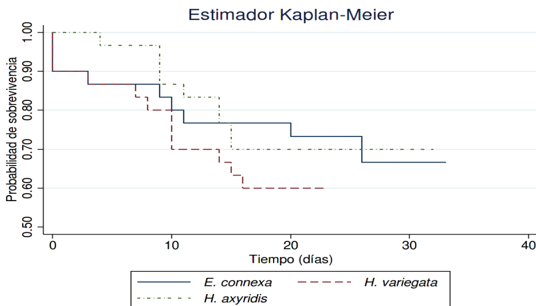
Fig. 2 Curvas de sobrevivencia de las tres especies E. connexa , H. variegata y H. axyridis . Se muestra la probabilidad de sobrevivencia acumulada.
