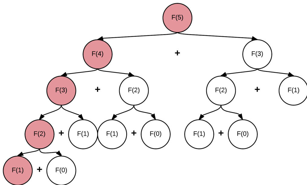
Figura 2.5: Cálculos hechos en serie de Fibonacci siguiendo perspectiva top-down. En rojo se puede observar los cálculos necesarios si se siguiera una perspectiva bottom-up.
