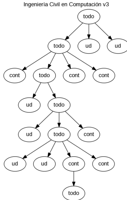
Figura 4.1: Árbol de planes con sus respectivas reglas como etiqueta de los nodos.
