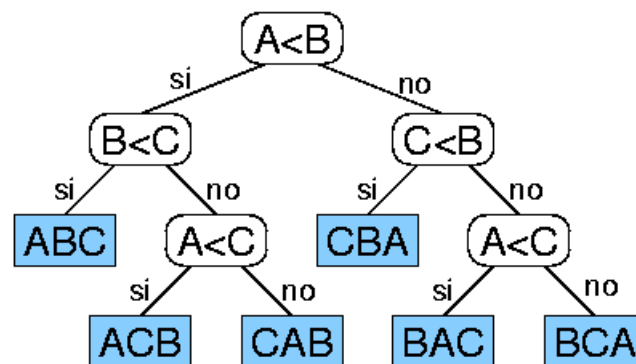
Figura 2.4: Árbol de decisión para ordenar tres elementos A, B y C.
