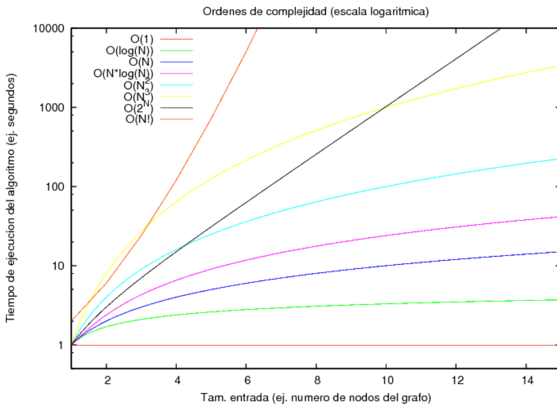
Figura 2.1: Gráfico con las curvas de órdenes de complejidad en una escala logarítmica
