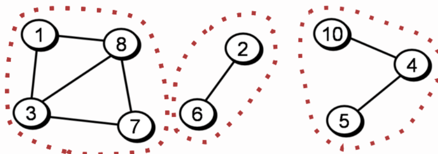
Figura 2.3: Ejemplo de componentes conexas.
