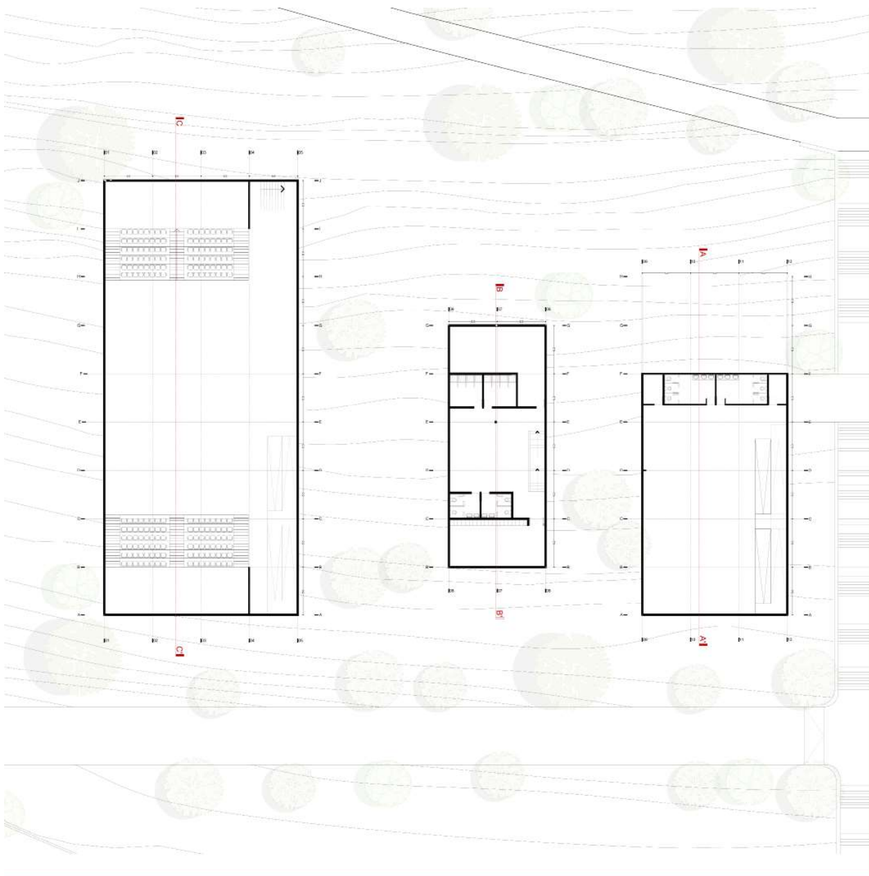
FIGURA 34 Proyecto Planta Nivel -1 Fuente: Elaboración propia
