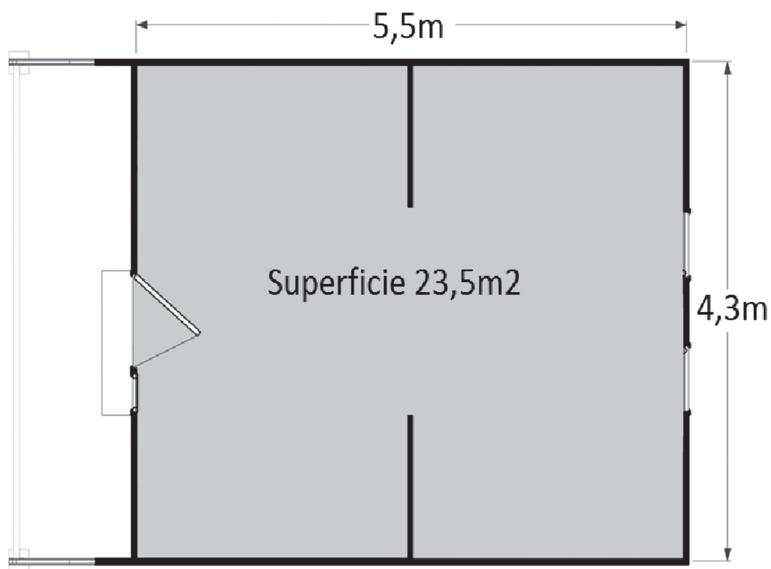
Figura 1. Planta de la vivienda de emergencia
