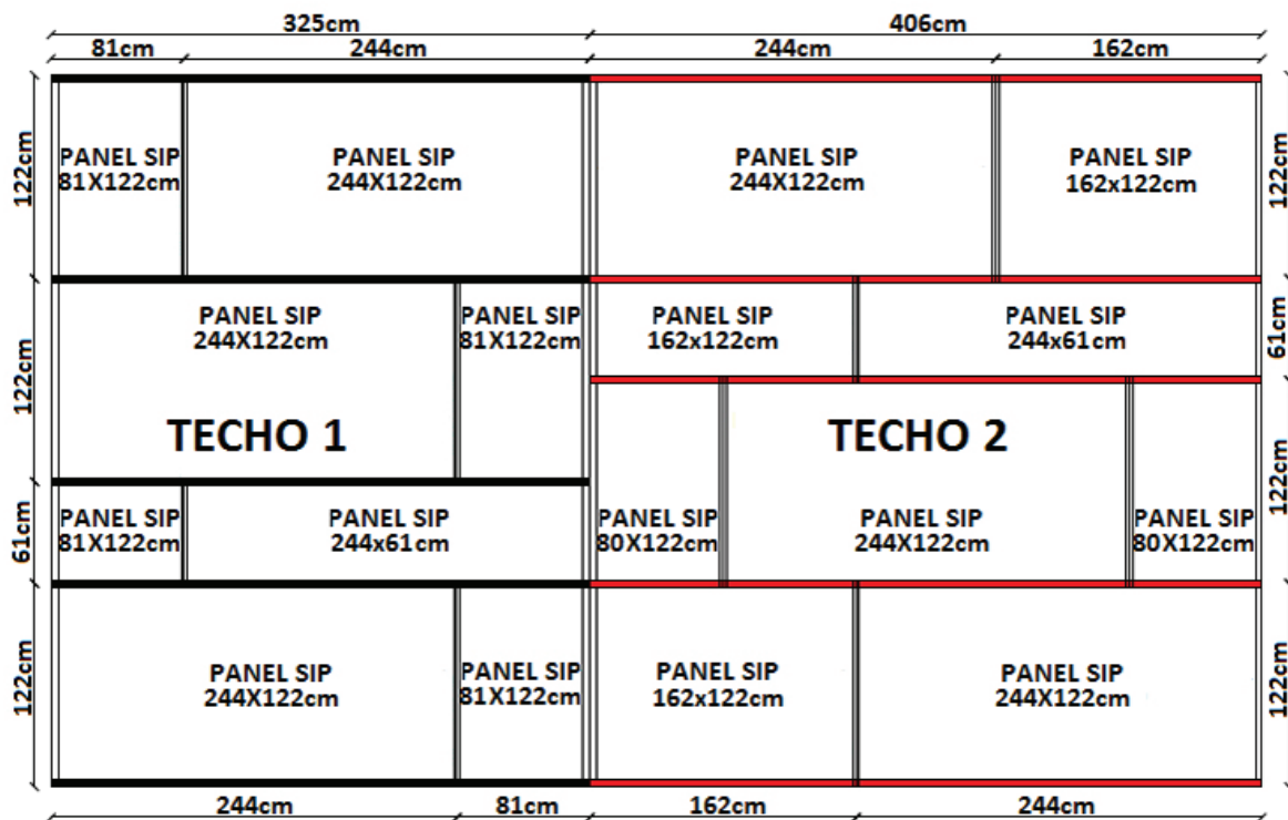
Figura 3 Vista en planta de la estructura de techo
