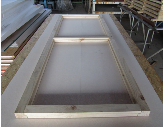
Figura 8a Preparación Ventanas
