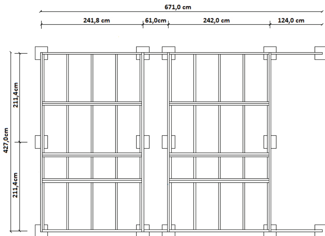
Figura 4. Vista en planta vigas de piso (Vigas periféricas en 2x6" y Vigas interiores en 2x4")
