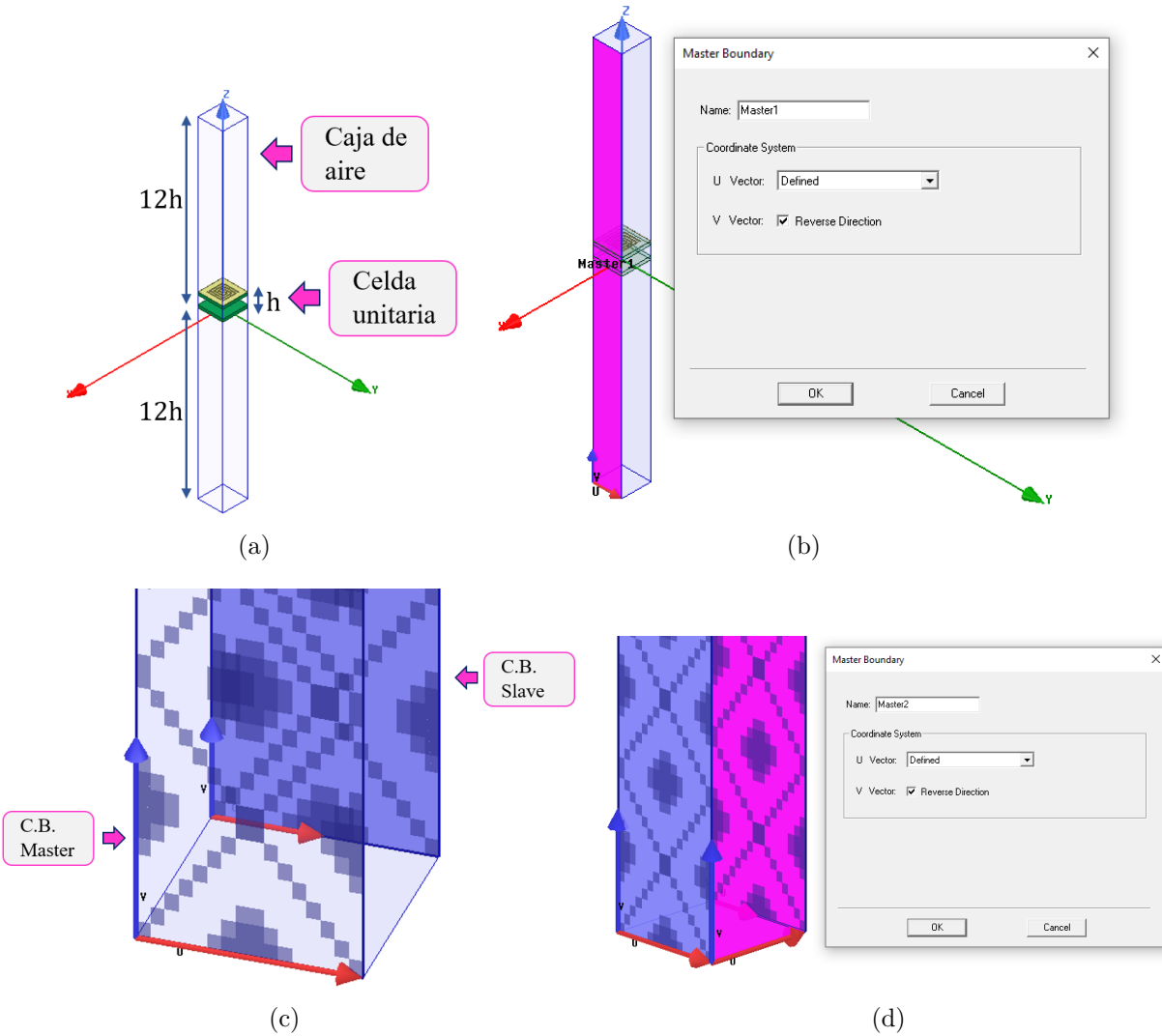
Figura A.2: Creación de los bordes de la estructura e incorporación de las condiciones de borde (C.B.). (a) Dimensiones de la caja de aire. (b) Creación de la primera C.B. master . (c) Disposición de las C.B. master y slave . (d) Creación de la segunda C.B. master (en magenta). Se muestra además su disposición con respecto a la primera C.B. master (en azul).
