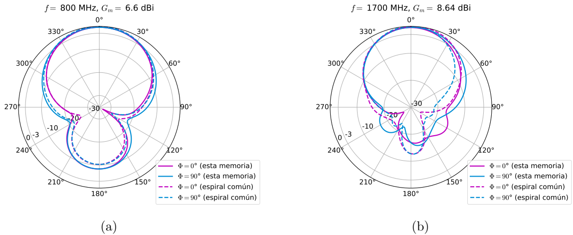
Figura 6.12: Ganancia total normalizada (en dB) de la espiral común con un plano reflector PEC y de la espiral de este trabajo con el plano reflector MTM. (a) 800 MHz. (b) 1700 MHz.
