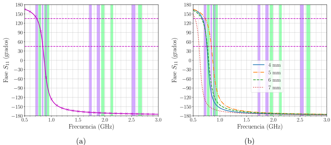
Figura 5.5: Fase del parámetro S_{11} de la celda unitaria de la Figura 5.4. El plano de referencia se ubica en el parche superior del MTM. (a) Valor nominal en la separación de aire (5 mm). (b) Sensibilidad en la separación de aire.
