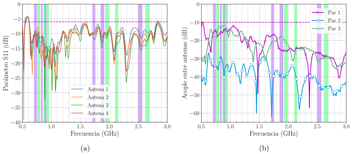
Figura 7.8: Magnitud de los parámetros S del arreglo de la Figura 7.3.b. La nomenclatura de antenas se muestra en la Figura 7.9. (a) Parámetro S_{11} . (b) Acople entre antenas.
