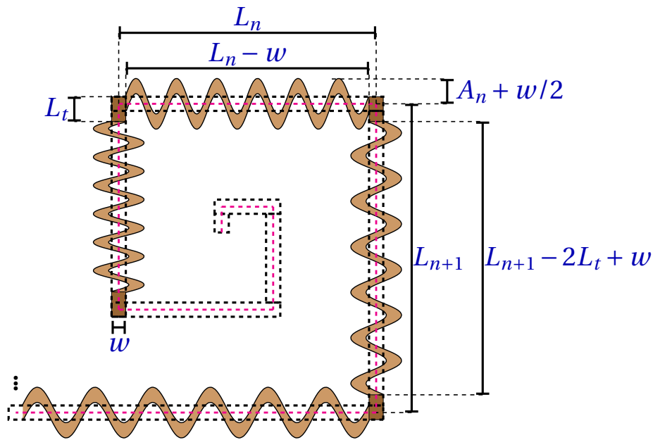
Figura 4.6: Implementación de las transiciones entre tramos. En línea punteada magenta se muestran los largos efectivos y en línea punteada negra se muestran las líneas de la espiral original de la Figura 4.2. L_t es el largo de la transición y su ancho es el mismo que el de las líneas que conforman la espiral ( w ).
