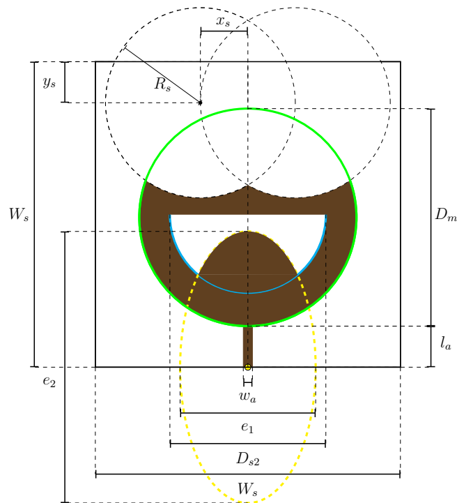
Figura 4.17: Diseño de la cara superior del monopolo circular miniaturizado. Se incorporaron agujeros para aumentar la inductancia y el factor de miniaturización. El contorno color cyan es un semicírculo centrado en el centro del sustrato. El contorno color amarillo es una elipse cuyo semieje mayor está alineado con el eje de simetría del diseño. El contorno color verde es el círculo principal que constituye el monopolo.
