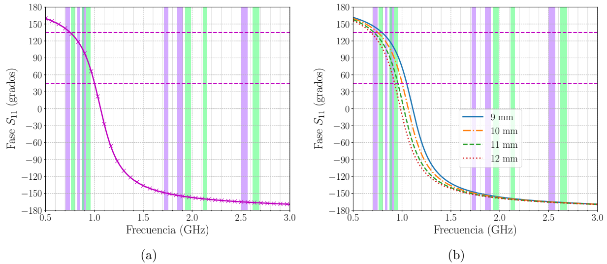
Figura 5.11: Fase del parámetro S_{11} de la celda unitaria de la Figura 5.9. El plano de referencia se ubica en el parche superior del MTM. (a) Valor nominal en la separación de aire (10 mm). (b) Sensibilidad en la separación de aire.
