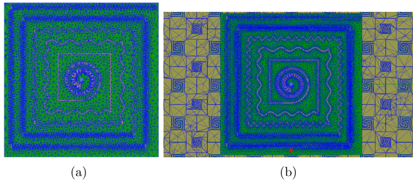
Figura 6.9: Ejemplo de la malla de discretización final en la simulación de la antenna con Kappa438 a 800 MHz. (a) Antena individual. (b) Antena con MTM.
