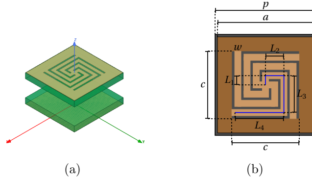
Figura 5.6: Unidad base del tercer metamaterial diseñado. El diseño se compone de dos placas de FR4 de 1.5 mm de espesor separadas por una distancia de 5 mm. La placa inferior no tiene ningún diseño (es decir, solo consta de un plano PEC en una cara). La unidad base tiene un tamaño de 15 mm \times 15 mm. La placa superior tiene brechas de 0.2 mm (es decir, el parche superior tiene un tamaño de 14.9 mm \times 14.9 mm). Las dos láminas de FR4 son de una sola cara. (a) Dibujo en HFSS. (b) Parámetros físicos. Al igual que con la antena espiral, se puede formar un solo brazo en las inductancias de espira. Los tres brazos restantes se obtienen con la ejecución de tres rotaciones consecutivas en 90°.
