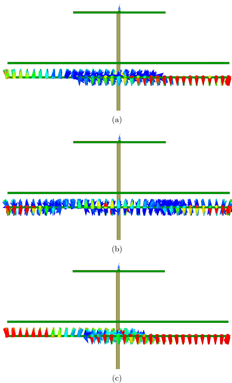
Figura 6.5: Campo eléctrico vectorial en una de las láminas de FR4 del MTM. (a) 800 MHz. (b) 1900 MHz. (c) 990 MHz. Como se puede observar, en 990 MHz el sustrato concentra más líneas de campo con intensidad máxima. Todas las figuras están sujetas a la misma escala: el color rojo representa el máximo y el color azul representa el mínimo.
