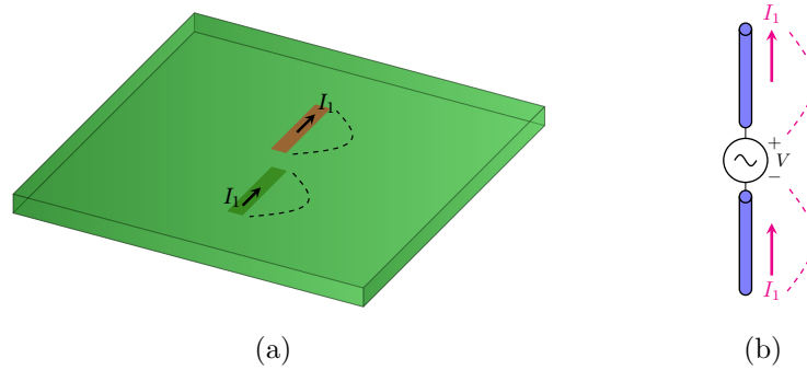
Figura 2.11: Distintas implementaciones de una antena dipolo. En línea punteada se muestra la amplitud de la corriente en función de la distancia al centro. (a) Implementación planar. En color café se muestran los conductores. El conductor café transparente se encuentra en la cara inferior del sustrato. (b) Implementación con alambres cilíndricos.
