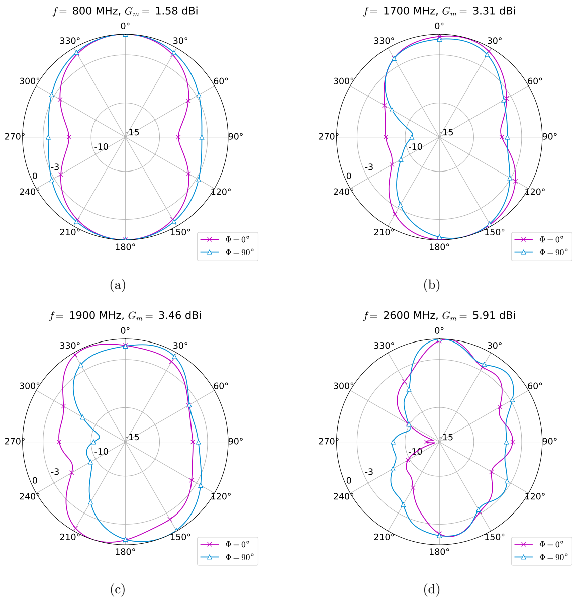
Figura 4.13: Ganancia total normalizada (en dB) de la espiral diseñada con Kappa438 en los planos xz ( \Phi = 0^\circ ) e yz ( \Phi = 90^\circ ). (a) 800 MHz. (b) 1700 MHz. (c) 1900 MHz. (d) 2600 MHz. Los valores máximos ( G_m ) se muestran sobre los gráficos.
