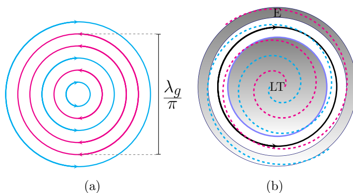
Figura 2.16: Descomposición de las antenas espirales de la Figura 2.15 en espiras equivalentes conectadas en serie. (a) Descomposición en espiras. (b) Zonas definidas en la espiral completa. El círculo LT corresponde a la zona de línea de transmisión, la espira con flechas corresponde a la zona de radiación y el área con la letra E es la zona de extinción de corriente.
