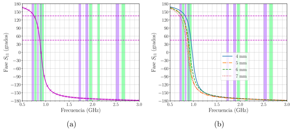
Figura 5.7: Fase del parámetro S_{11} de la celda unitaria de la Figura 5.6. El plano de referencia se ubica en el parche superior del MTM. (a) Valor nominal en la separación de aire (5 mm). (b) Sensibilidad en la separación de aire.
