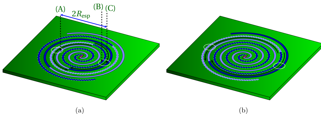
Figura 2.15: Distribución de corrientes en las antenas espirales. El centro es alimentado por una fuente ideal (puerto concentrado) idéntico al mostrado en la Figura 2.14. Los colores para representar la dirección del flujo de corriente son idénticos a los de la Figura 2.14. R_{\text{esp}} es el radio de las espiras equivalentes. (a) Frecuencia de alimentación: \omega_1 . Por definición, los puntos (A) y (B) tienen igual amplitud pero están desfasados en 180^\circ . Por ende, si la distancia entre (A) y (C) a través de la espiral (es decir, \pi R_{\text{esp}} ) es igual a \lambda_g/2 , la polaridad es invertida, con lo que (B) y (C) están en fase. (b) Frecuencia de alimentación: \omega_2 < \omega_1 .
