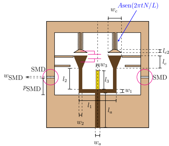
Figura 4.19: Diseño final del monopolo tenedor miniatura. En color café claro se muestra la cara inferior y en color café oscuro y amarillo se muestra la cara superior. El eje de simetría es marcado con línea punteada. t es la variable de parametrización que recorre el meandro.
