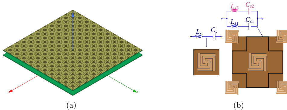
Figura 5.8: (a) Plano MTM de 20 cm \times 20 cm. La celda unitaria se compone de dos parches distintos y se muestra en la Figura 5.9. (b) Modelos circuitales del diseño de la Figura 5.6 y del último diseño propuesto.
