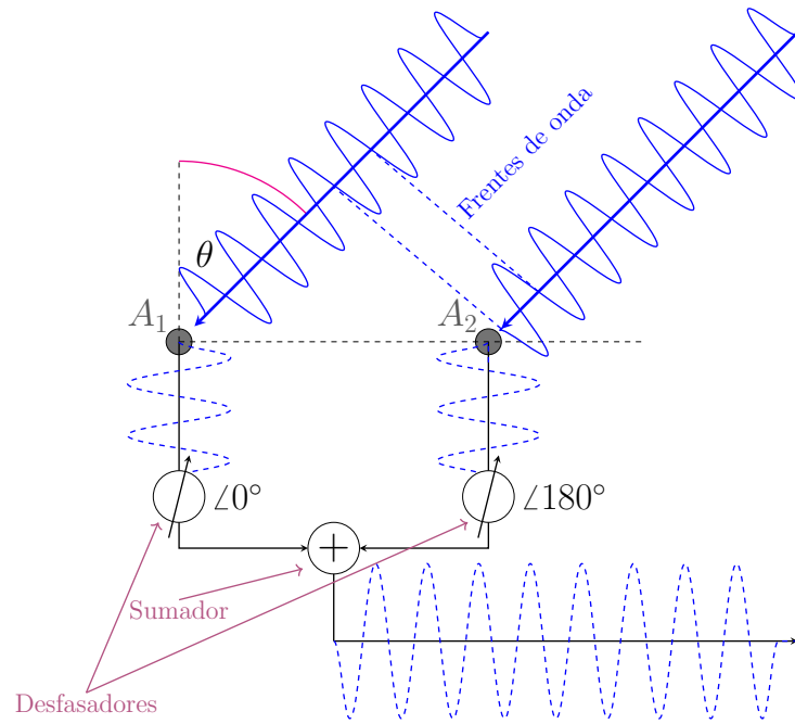
Figura 2.17: Diagrama de un arreglo de 2 antenas operando en el modo de recepción. Las ondas en espacio libre se representan con señales senoidales en línea continua y las ondas en cables se representan en línea punteada. Las antenas se representan con círculos negros ( A_1 y A_2 ). Como se puede observar, las señales en espacio libre llegan desfasadas en 180^\circ a las antenas. Si este desfase es corregido, se puede lograr que las ondas interfieran constructivamente en la dirección mostrada.
