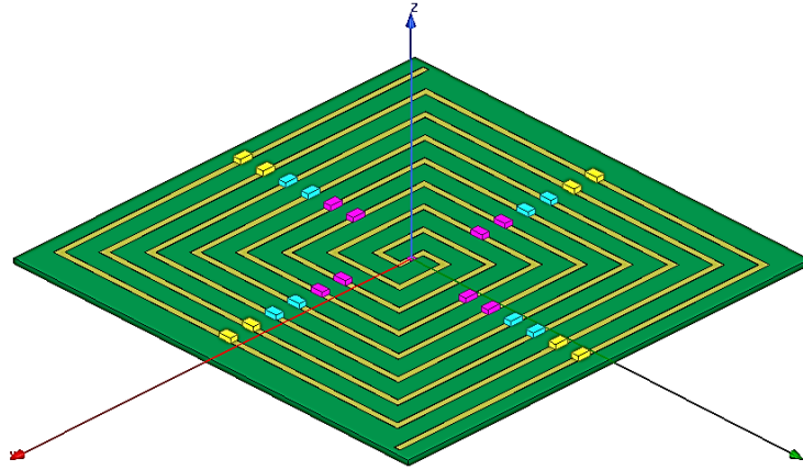
Figura 4.3: Dibujo en HFSS de una espiral cuadrada cargada con inductancias SMD. En esta simulación se usó un puerto concentrado ( lumped port ) en lugar de un coaxial. La impedancia del puerto se configuró de manera tal que se obtuviera la mejor adaptación posible. En magenta se muestra el primer grupo de inductancias (todas con valor L_1 ), en cian el segundo grupo (con valor L_2 ) y en amarillo el tercer grupo (con valor L_3 ).
