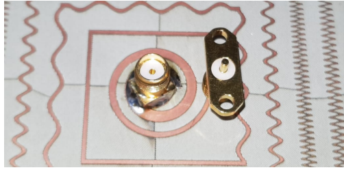
Figura 3.5: Conector SMA de panel usado. A la derecha se muestra el conector original. A la izquierda se muestra el conector cortado y montado en el prototipo final de la antena espiral.
