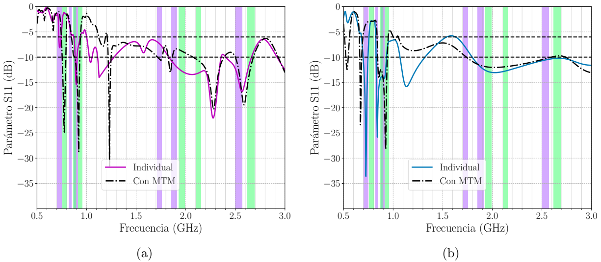
Figura 6.2: Magnitud del parámetro S_{11} . (a) Sustrato de la espiral: Kappa438. (b) Sustrato de la espiral: FR4.
