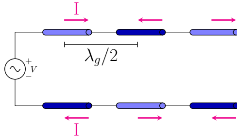
Figura 2.14: Línea de transmisión convencional con propagación en modo TEM. I es la corriente que circula por los conductores. Los semiciclos positivos y negativos se representan con colores de distintas tonalidades. La fuente de alimentación es ideal (amplitud de voltaje constante y tamaño infinitesimal). El cambio de polaridad cada \lambda_g/2 se da incluso cuando el modo de propagación no es TEM.
