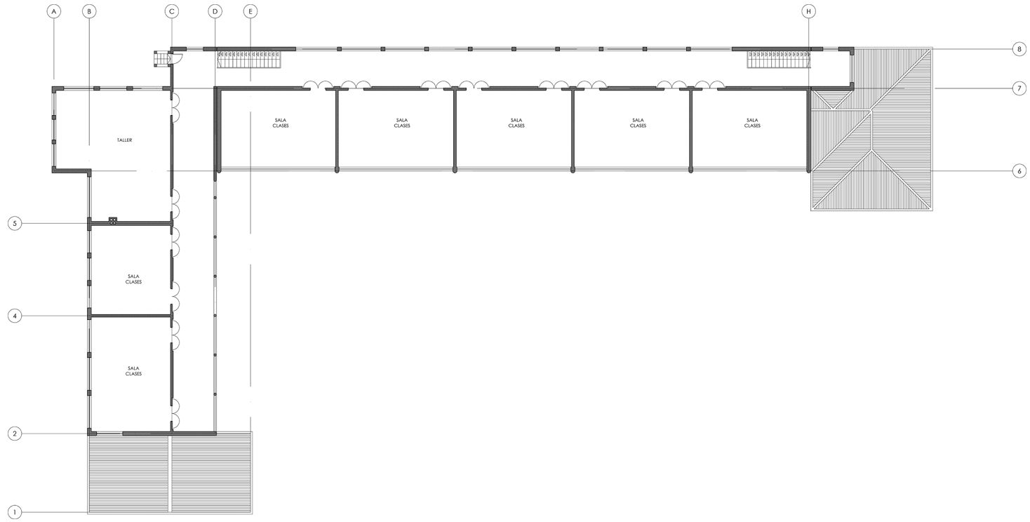
Figura 3.3: Planta Segundo Nivel Escuela Española de San Antonio
