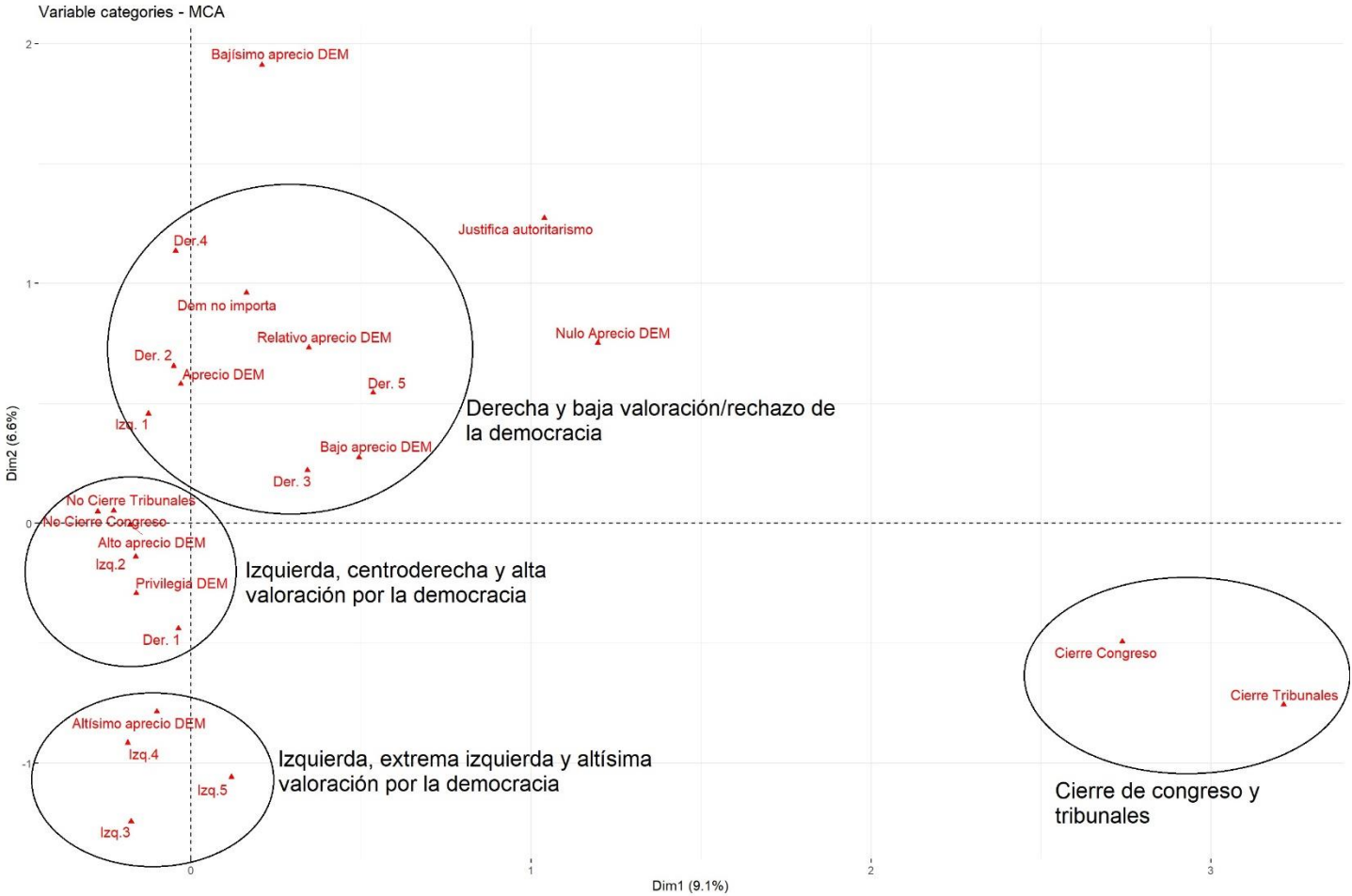
Gráfico 3: Cierre del congreso (JC15), Cierre del poder judicial (JC16), escala de preferencia por la democracia (ING4) y valoración personal de la democracia (DEM2) en LAPOP 2010.
