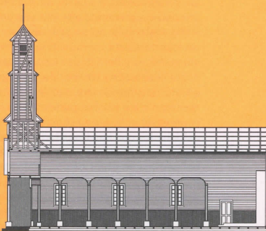
Corte _ Section
