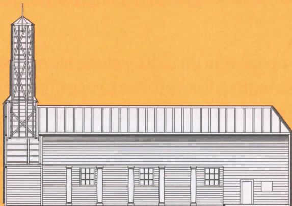
Corte _ Section
