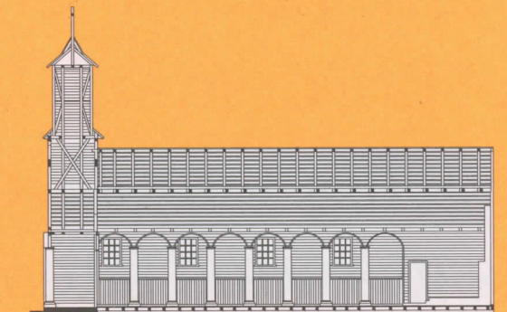
Corte _ Section
