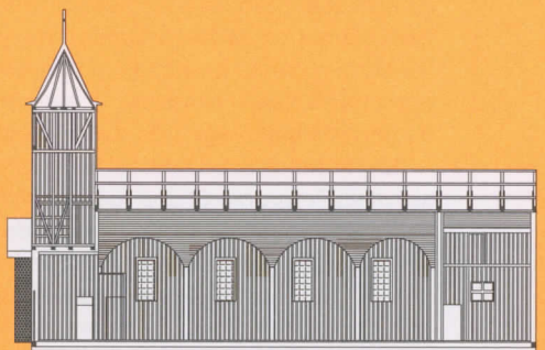
Corte _ Section
