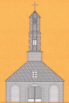
Elevación _ Elevation
