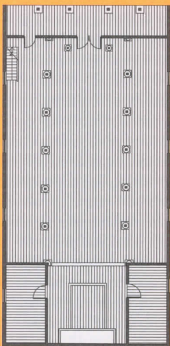
Planta _ Plan
