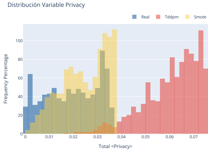
Figura 4.8: Frecuencia del campo Privacy en el modelo real y Top 2, King county (A-1)
