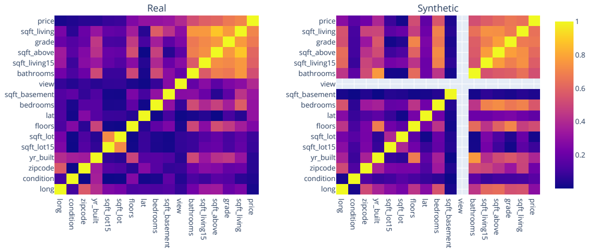
Figura A.2: Correlación de conjunto original de entrenamiento y Tvae, King county (A-3)
