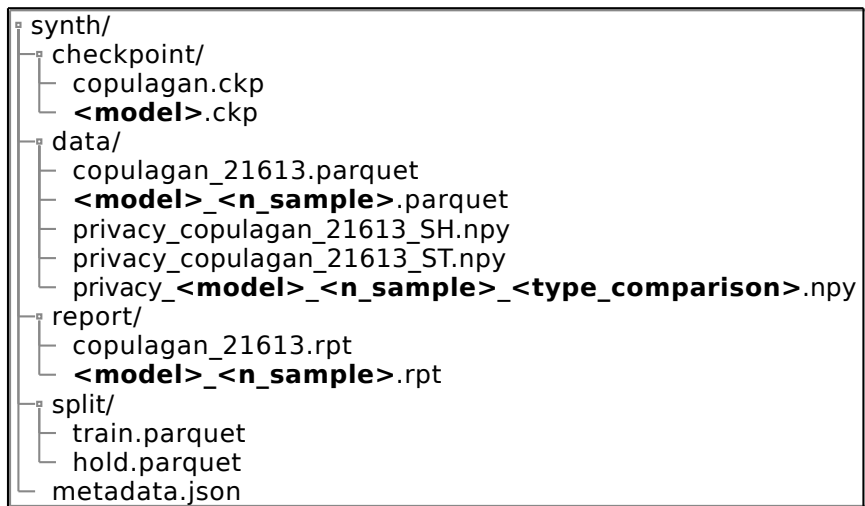
Figura 3.3: Carpetas y archivos esperados generados por Synthetic
