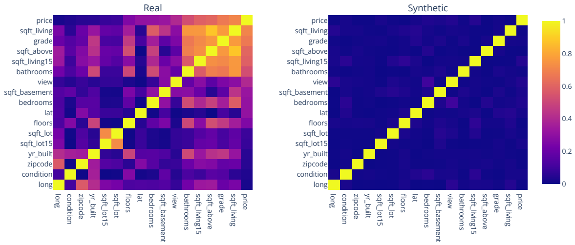
Figura A.4: Correlación de conjunto original de entrenamiento y Ctgan, King county (A-3)
