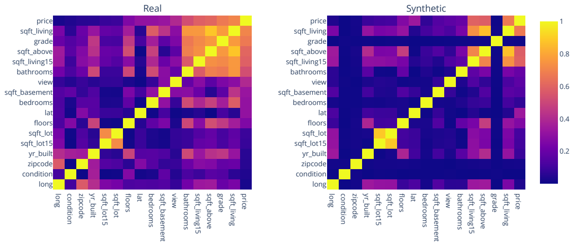
Figura A.3: Correlación de conjunto original de entrenamiento y Gaussiancopula, King county (A-3)
