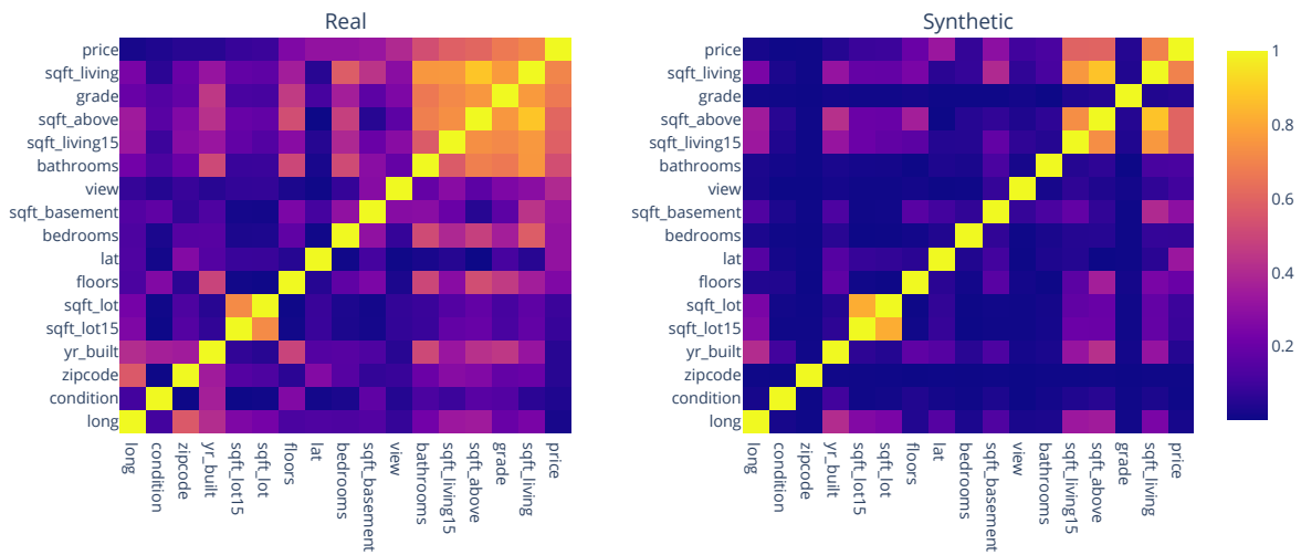
Figura A.5: Correlación de conjunto original de entrenamiento y Tablepreset, King county (A-3)
