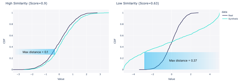
Figura 2.1: Ejemplo de SDMetric en calculo de CDF [30]
