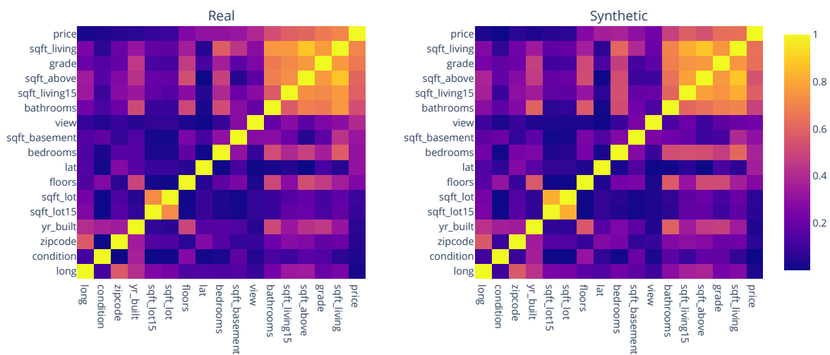
Figura A.6: Correlación de conjunto original de entrenamiento y Smote, King county (A-3)
