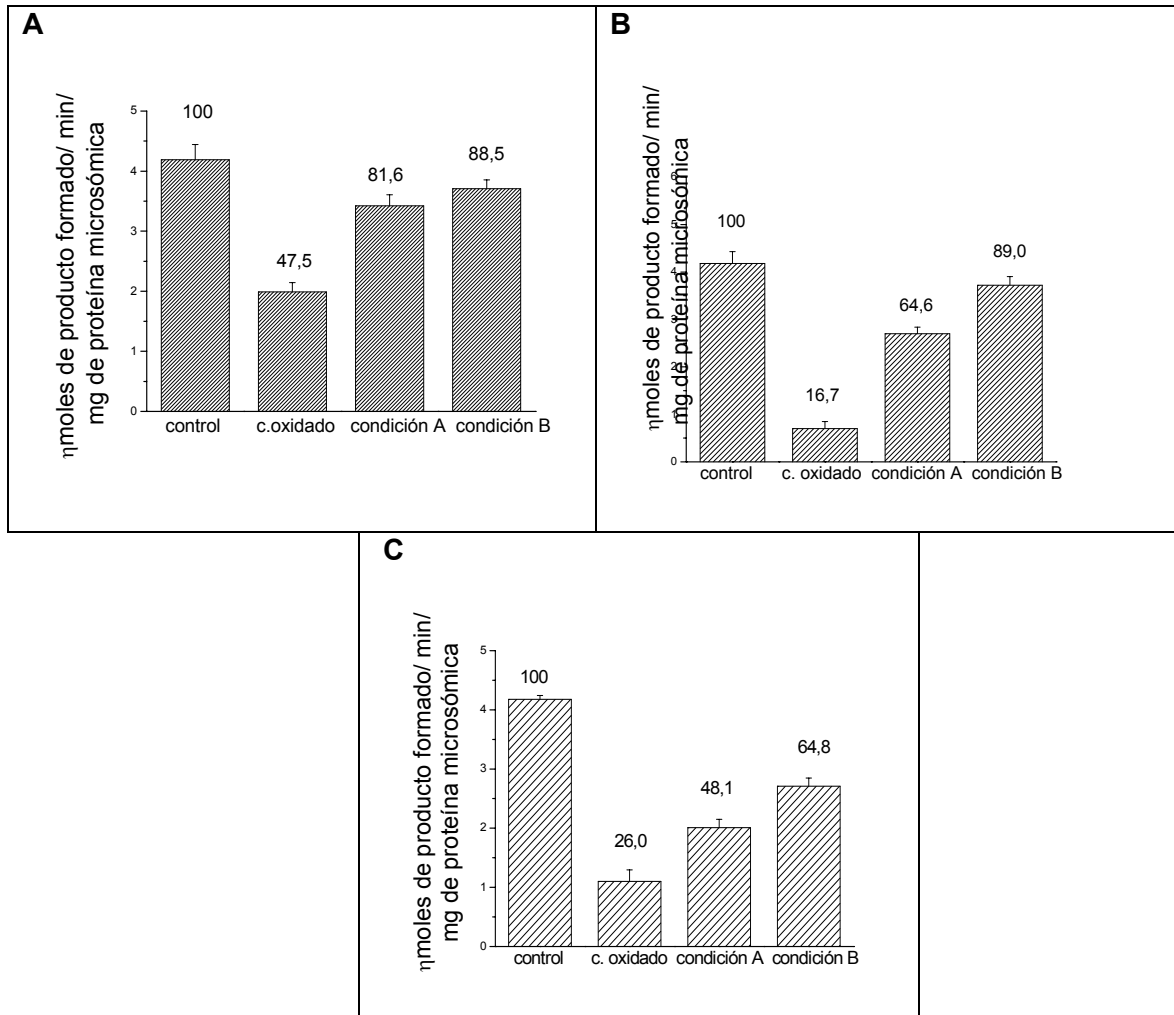
Figura 11. O-Desmetilación de p-nitroanisol en presencia de naftaleno (A), Nitrofurantoína (B) y Nifurtimox (C). Efecto de GSH y DTT. [Proteína microsómica]: 2 mg/mL; [naftaleno]: 0,5 mM; [Nitrofurantoína] 10 \mu M; [Nifurtimox] 10 \mu M. Control: sistema en ausencia de los xenobióticos. C. oxidado: sistema en presencia de los xenobióticos. Condición A: La proteína microsómica se preincubó durante 5 minutos con GSH 2 mM y luego se adicionaron los xenobióticos. Condición B: La proteína microsómica se preincubó durante 5 minutos con DTT 2 mM y luego se adicionaron los xenobióticos. La O-desmetilación se determinó de acuerdo a lo descrito en Métodos. Los valores representan la media de al menos 4 experimentos independientes \pm su desviación estándar
