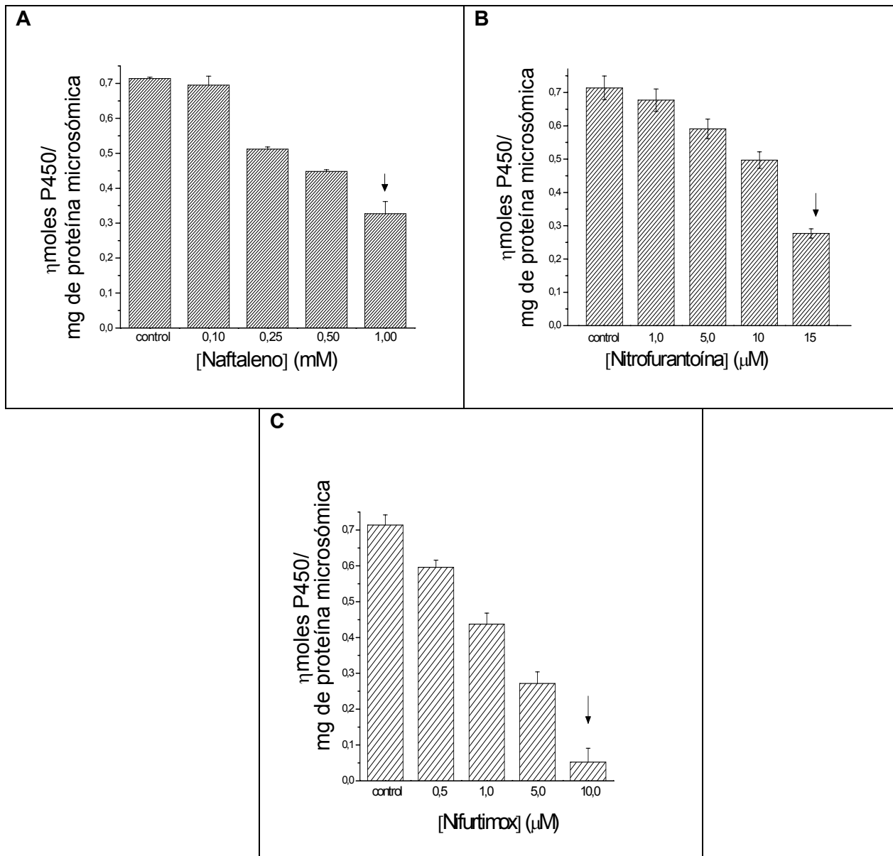
Figura 7. Efecto de naftaleno (A), Nitrofurantoina (B) y Nifurtimox (C) sobre el contenido microsómico de la monooxigenasa citocromo P450. [Proteína microsómica]: 1,0 mg/mL. El contenido de citocromo P450 se determinó de acuerdo a lo descrito en Métodos. Los valores corresponden a la diferencia entre los ηmoles de citocromo P450 obtenidos al adicionar los xenobióticos a los microsomas antes de adicionar ditionito de sodio y después de adicionar este reductor. Las flechas sobre las barras corresponden a las concentraciones elegidas para realizar los experimentos posteriores. Los valores representan la media de al menos 4 experimentos independientes \pm su desviación estándar.
