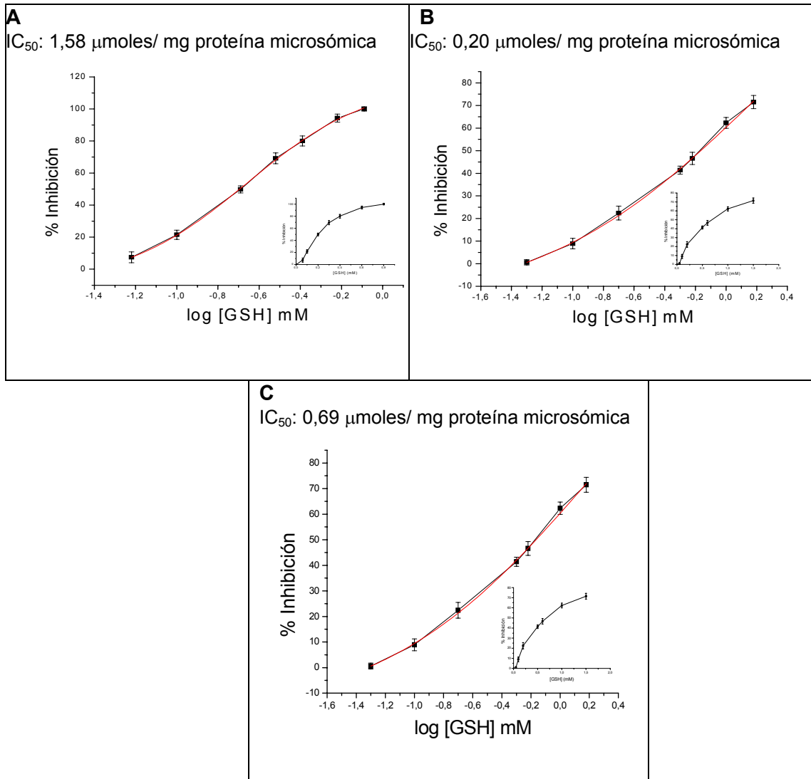
Figura 4. Lipoperoxidación microsómica inducida por biotransformación a través del sistema citocromo P450 de naftaleno (A), Nitrofurantoina (B) y Nifurtimox (C). Efecto de GSH. A: [Naftaleno] 0,5 mM y [proteína microsómica] 0,2 mg/mL; B: [Nitrofurantoina] 1 mM y [proteína microsómica] 1,0 mg/mL; C: [Nifurtimox] 1mM y [proteína microsómica] 1,0 mg/mL. La proteína microsómica fue preincubada a 37° C durante 10 minutos antes de inducir la lipoperoxidación de acuerdo a lo descrito en Métodos. C Los gráficos insertos representan las curvas concentración-respuesta obtenidas de los datos experimentales directos. El valor de IC_{50} corresponde a la concentración de GSH que inhibió en un 50% la lipoperoxidación inducida por metabolismo de los xenobióticos. Los valores representan la media de al menos 4 experimentos independientes \pm su desviación estándar.
