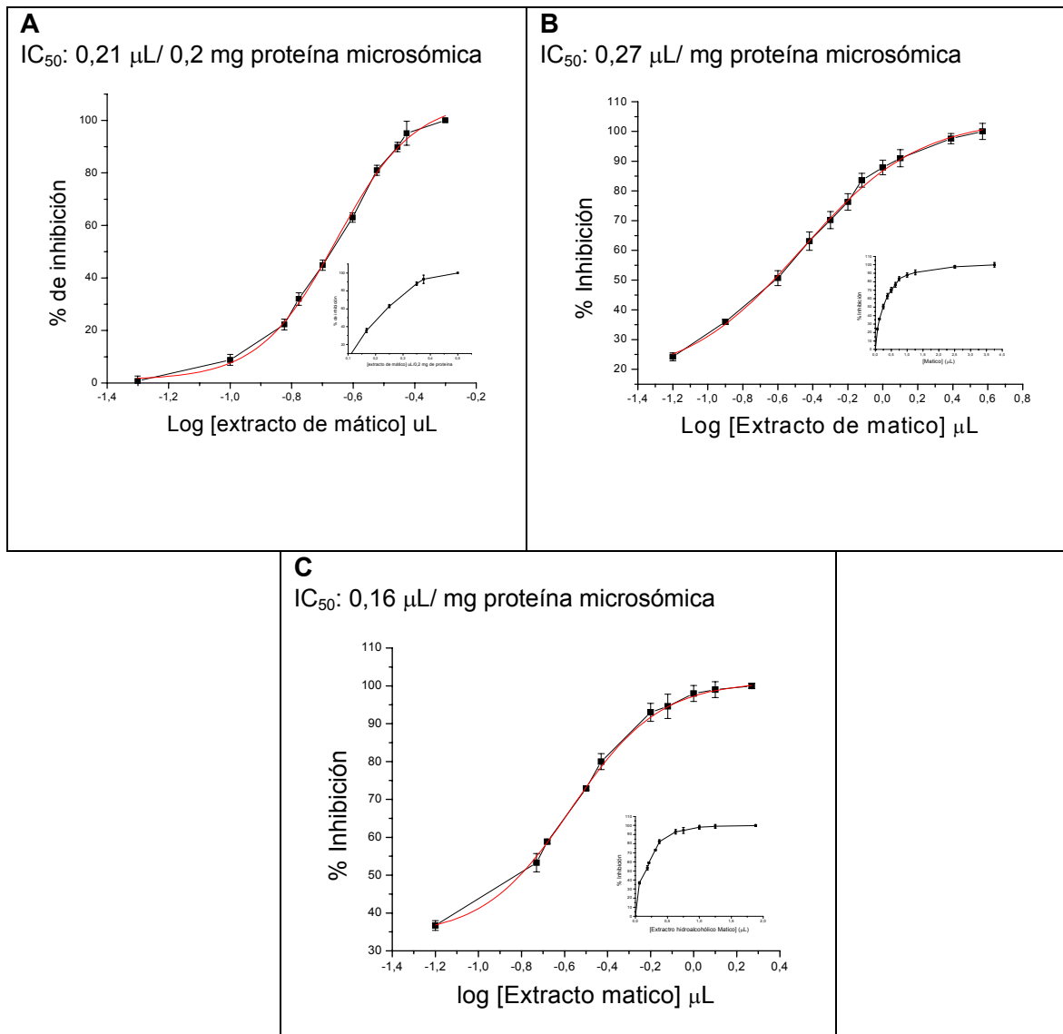
Figura 5. Lipoperoxidación microsómica inducida por metabolismo oxidativo de Naftaleno (A), Nitrofurantoina (B) y Nifurtimox (C). Efecto del extracto hidroalcohólico de Buddleja globosa (matico). A:[Naftaleno] 0,5 mM y [proteína microsómica] 0,2 mg/mL; B: [Nitrofurantoina] 1 mM y [proteína microsómica] 1,0 mg/mL; C: [Nifurtimox] 1mM y [proteína microsómica] 1,0 mg/mL. La proteína microsómica fue preincubada a 37° C durante 10 minutos con el extracto de matico antes de inducir la lipoperoxidación de acuerdo a lo descrito en Métodos. Los gráficos insertos representan las curvas concentración-respuesta obtenidas de los datos experimentales directos. El valor de IC_{50} corresponde a la concentración de matico que inhibió en un 50% la lipoperoxidación inducida por metabolismo de los xenobióticos. Los valores representan la media de al menos 4 experimentos independientes \pm su desviación estándar.
