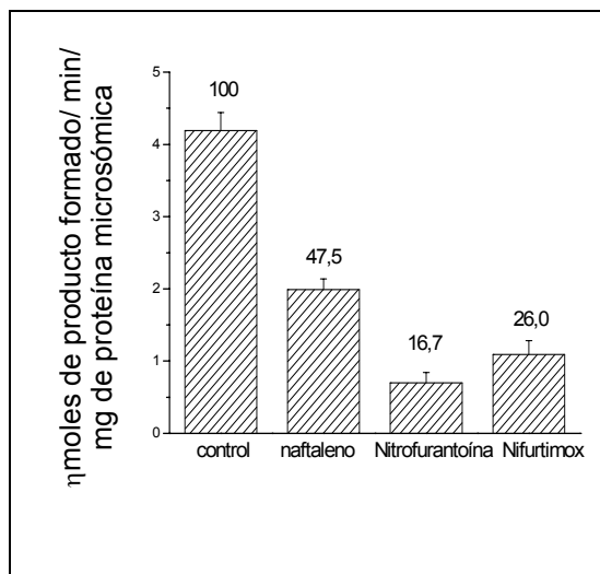
Figura 10. Efecto de naftaleno, Nitrofurantoina y Nifurtimox sobre la O-desmetilación de p-nitroanisol. [Proteína microsómica]: 2 mg/mL; [naftaleno]: 0,5 mM; [Nitrofurantoina] 10 \mu M; [Nifurtimox] 10 \mu M. Control: sistema en ausencia de los xenobióticos. La O-desmetilación se determinó de acuerdo a lo descrito en Métodos. Los valores representan la media de al menos 4 experimentos independientes \pm su desviación estándar.
