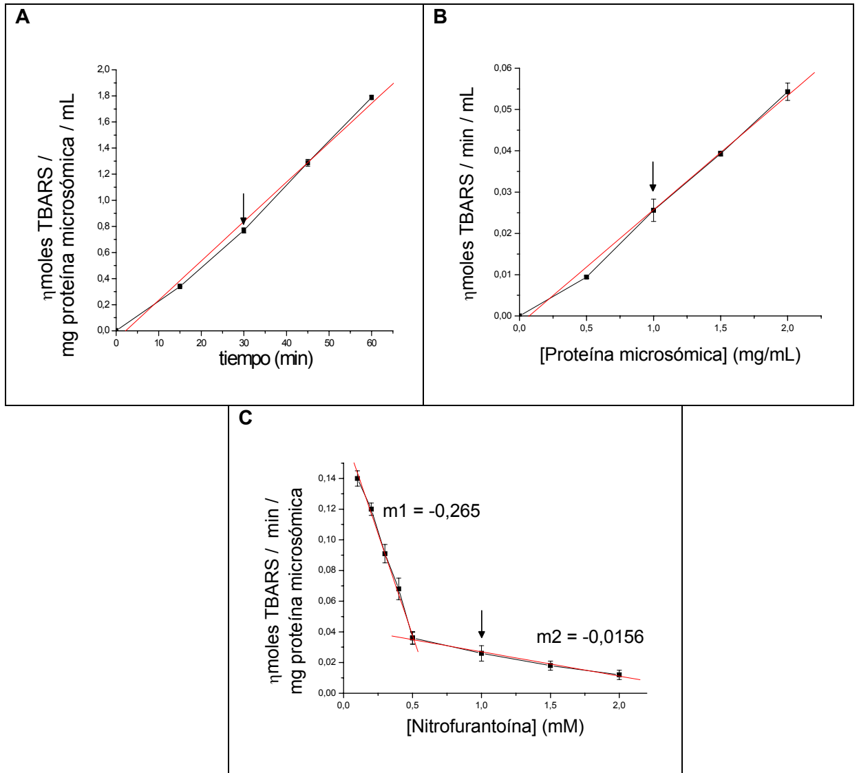
Figura 2. Lipoperoxidación microsómica inducida por metabolismo de Nitrofurantoína a través del sistema citocromo P450. A: [Proteína microsómica]: 1,0 mg/mL; [Nitrofurantoína]:1,0 mM. B: [Nitrofurantoína]:1,0 mM; tiempo de incubación: 30 minutos. C: [Proteína microsómica]: 1,0 mg/mL; tiempo de incubación: 30 minutos. Las flechas sobre los gráficos indican las condiciones de tiempo de incubación, concentración de proteína y de Nitrofurantoína seleccionadas para realizar los experimentos posteriores. La determinación de lipoperoxidación fue realizada de acuerdo a lo descrito en Métodos. Los valores representan la media de al menos 4 experimentos independientes \pm su desviación estándar. Los valores de regresión lineal de las rectas fueron: rA: 0,9967; rB: 0,9972; rCm1: 0,9935; rCm2: 0,9978.
