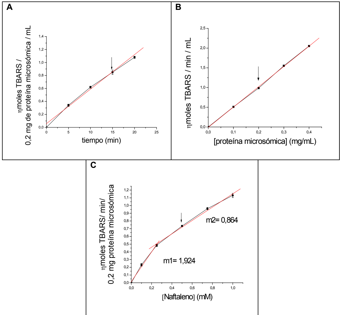
Figura 1. Lipoperoxidación microsómica inducida por metabolismo oxidativo de Naftaleno a través del sistema citocromo P450. A: [Proteína microsómica]: 0,2 mg/mL; [Naftaleno] 0.5 mM. B: [Naftaleno]: 0.5 mM; tiempo de incubación: 15 minutos C: [Proteína microsómica]: 0.2 mg/mL; tiempo de incubación: 15 minutos. Las flechas sobre los gráficos indican las condiciones de tiempo de incubación, concentración de proteína y de naftaleno seleccionadas para realizar los experimentos posteriores. La determinación de lipoperoxidación fue realizada de acuerdo a lo descrito en Métodos. Los valores representan la media de al menos 4 experimentos independientes \pm su desviación estándar. Los valores de regresión lineal de las rectas fueron: rA: 0,9916; rB: 0,99972; rCm1: 0,99606; rCm2:0,99666
