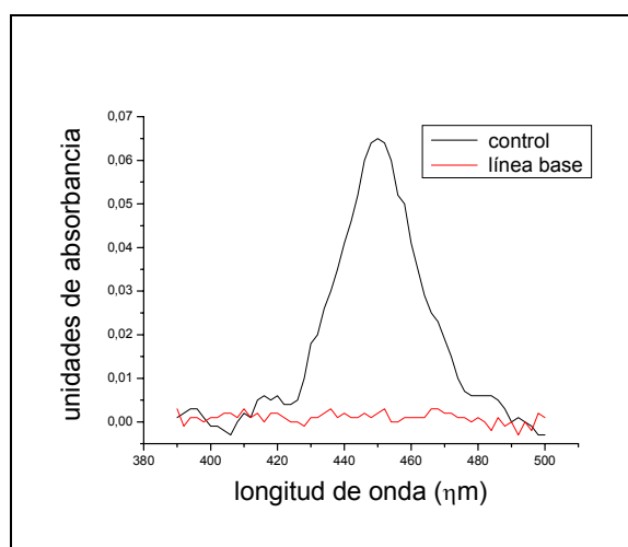
Figura 6. Espectro control de la absorbancia de la monooxigenasa citocromo P450 microsómica. [Proteína microsómica]: 1,0 mg/mL. La técnica utilizada para realizar la determinación del espectro de absorción de la monooxigenasa citocromo P450 está descrita en Métodos.
