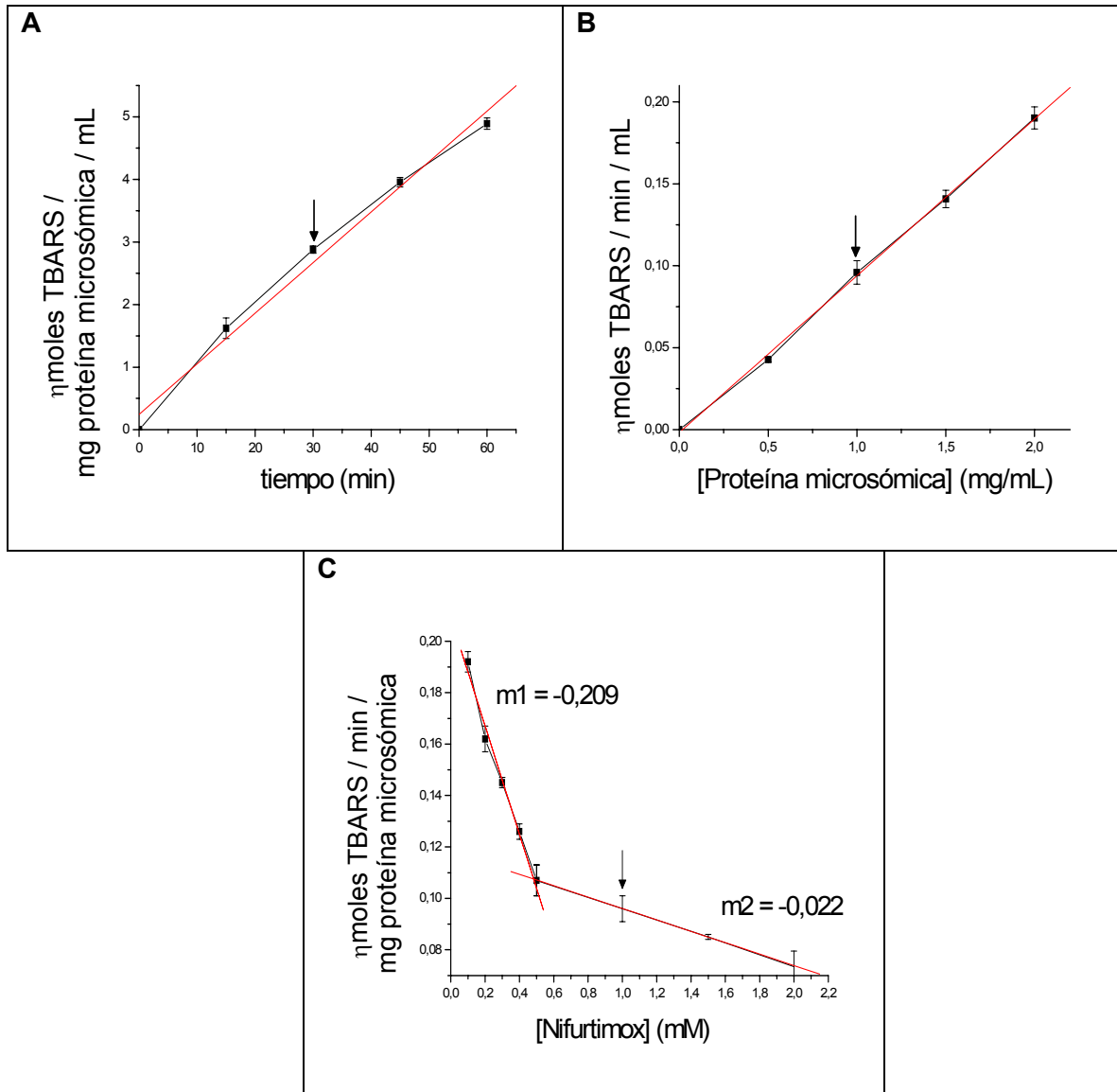
Figura 3. Lipoperoxidación microsómica inducida por metabolismo de Nifurtimox a través del sistema citocromo P450. A: [Proteína microsómica]: 1,0 mg/mL; [Nifurtimox]:1,0 mM. B: [Nifurtimox]: 1,0 mM; tiempo de incubación: 30 minutos. C: [Proteína microsómica]: 1,0 mg/ mL; tiempo de incubación: 30 minutos. Las flechas sobre los gráficos indican las condiciones de tiempo de incubación, concentración de proteína y de Nifurtimox seleccionadas para realizar los experimentos posteriores. La determinación de lipoperoxidación fue realizada de acuerdo a lo descrito en Métodos. Los valores representan la media de al menos 4 experimentos independientes \pm su desviación estándar. Los valores de regresión lineal de las rectas fueron: rA: 0,9940; rB: 0,9996; r m1 : 0,9943; r m2 : 0,9998.
