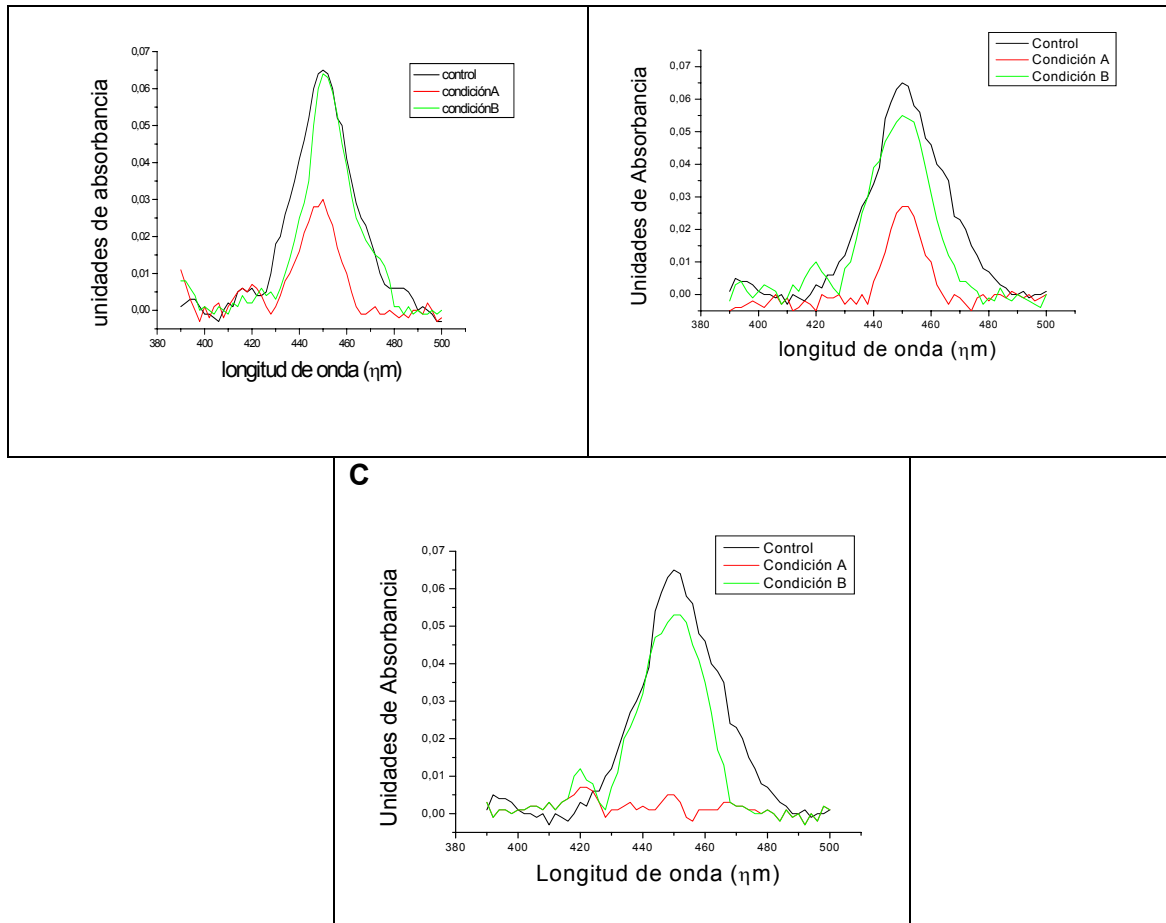
Figura 8. Efecto de naftaleno (A) Nitrofurantoína (B) y Nifurtimox (C) sobre el espectro de absorbancia de la monooxigenasa citocromo P450 microsómica. [Proteína microsómica]: 1,0 mg/mL. [Naftaleno]: 0,5 mM; [Nitrofurantoína]: 15 \mu M; [Nifurtimox]: 10 \mu M. Condición A: los microsomas fueron preincubados 5 min con el xenobiótico y luego se adicionó ditionito de sodio para determinar el espectro de absorbancia. Condición B: los microsomas, el xenobiótico y el ditionito fueron incubados durante 5 min antes de realizar el espectro de absorbancia. La determinación del espectro de absorbancia se realizó de acuerdo a lo descrito en Métodos. Los valores representan la media de al menos 4 experimentos independientes \pm su desviación estándar.
