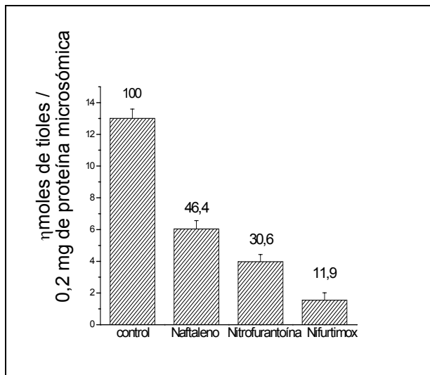
Figura 9. Contenido total de tioles microsómicos. Efecto de naftaleno, Nitrofurantoína y Nifurtimox en condiciones de biotransformación por el sistema citocromo P450. [Proteína microsómica]: 0,2 mg/mL; [naftaleno]: 0,5 mM; [Nitrofurantoína]: 10 \mu M; [Nifurtimox]: 10 \mu M. El contenido total de tioles se determinó de acuerdo a lo descrito en Métodos. Los valores representan la media de al menos 4 experimentos independientes \pm su desviación estándar.
