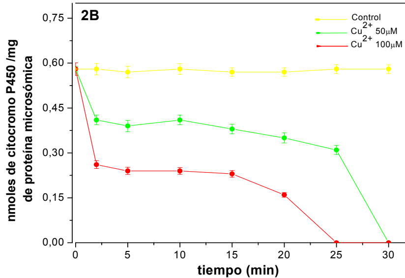
Figura 2. Efecto temporal de Cu +2 (2A) y Cu +2 /ascorbato (2B) sobre el espectro de absorbancia de la monooxigenasa citocromo P450. [Proteína microsómica]: 1mg/mL; [ascorbato]: 1mM. Los microsomas fueron incubados durante 15 minutos con las distintas concentraciones de Cu +2 y Cu +2 /ascorbato antes de medir el espectro de absorbancia. La concentración de ascorbato utilizada fue 1mM. La absorbancia del complejo monooxigenasa citocromo P450-CO fue convertida a nanomoles de enzima usando su coeficiente de extinción 91 mM -1 x cm -1 . Los valores representan el promedio de 4 experimentos independientes ± S.D.
