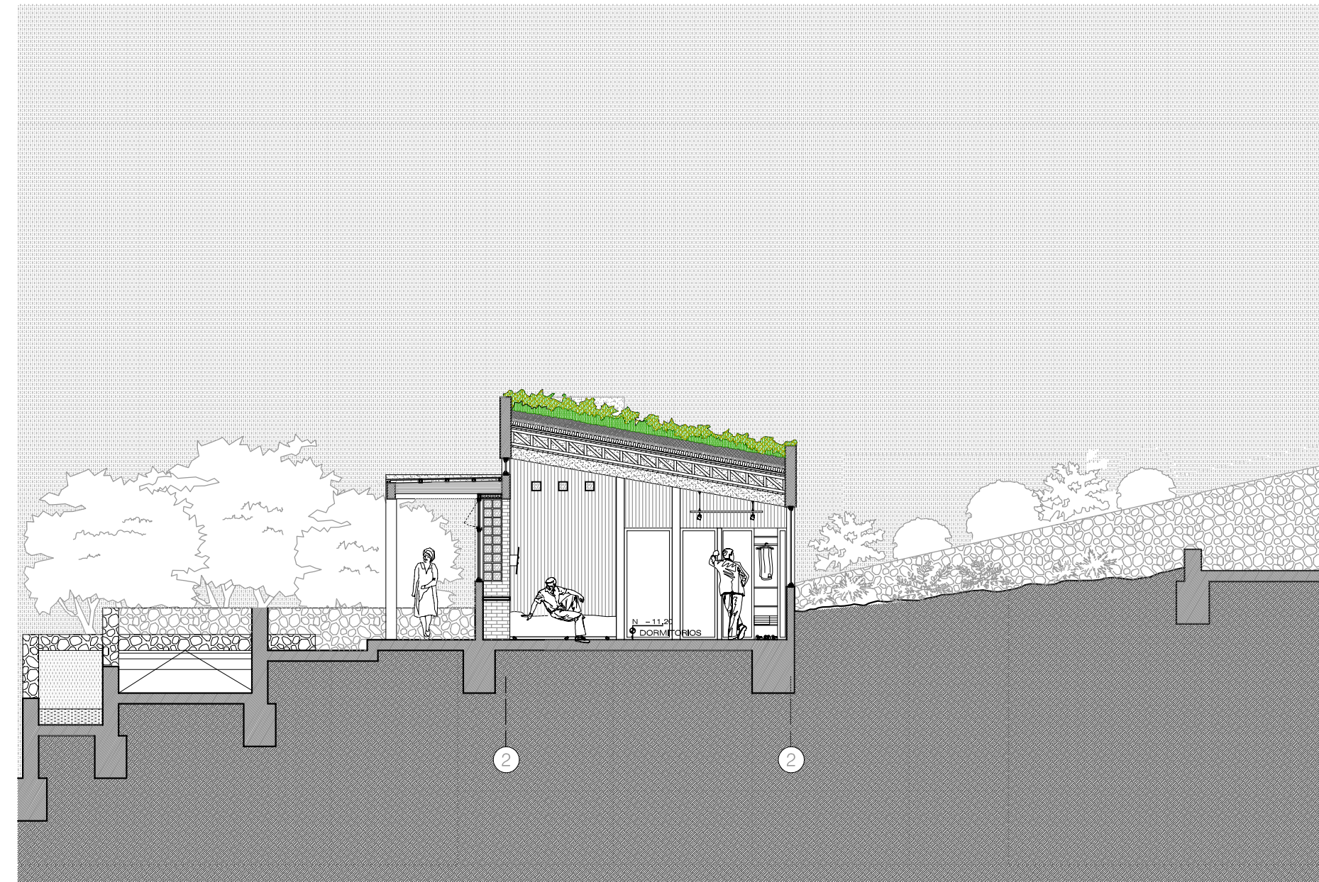
CORTE DORMITORIOS VARONES
