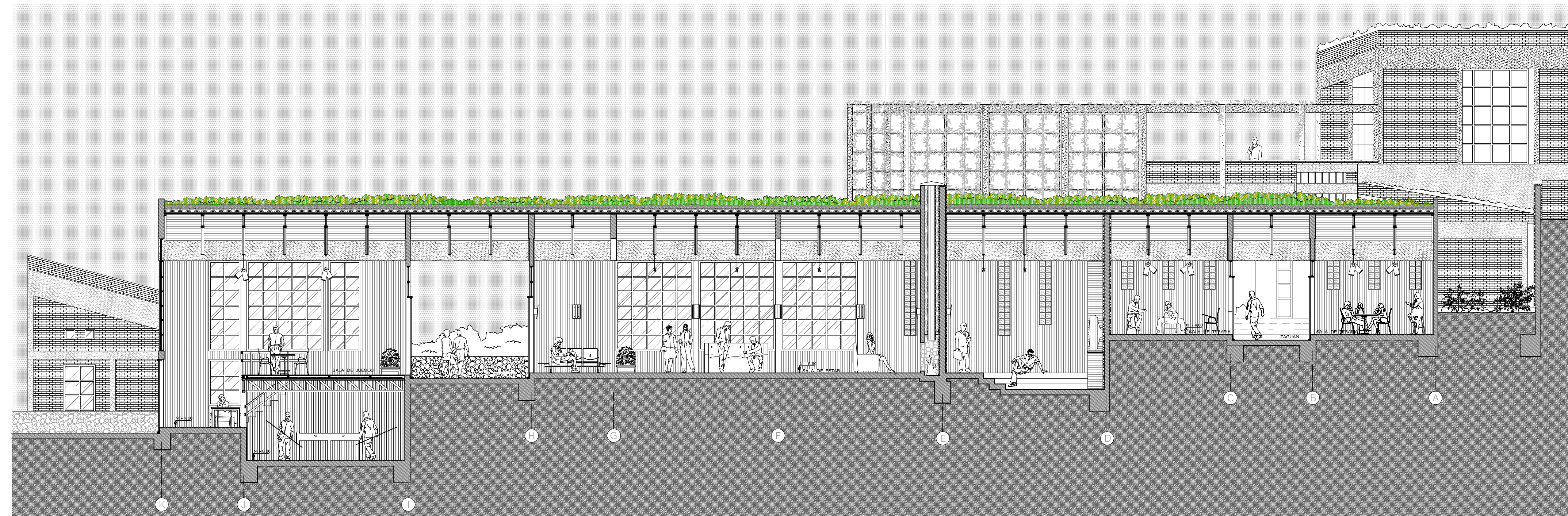
CORTE SALA DE ESTAR - TERAPIAS
