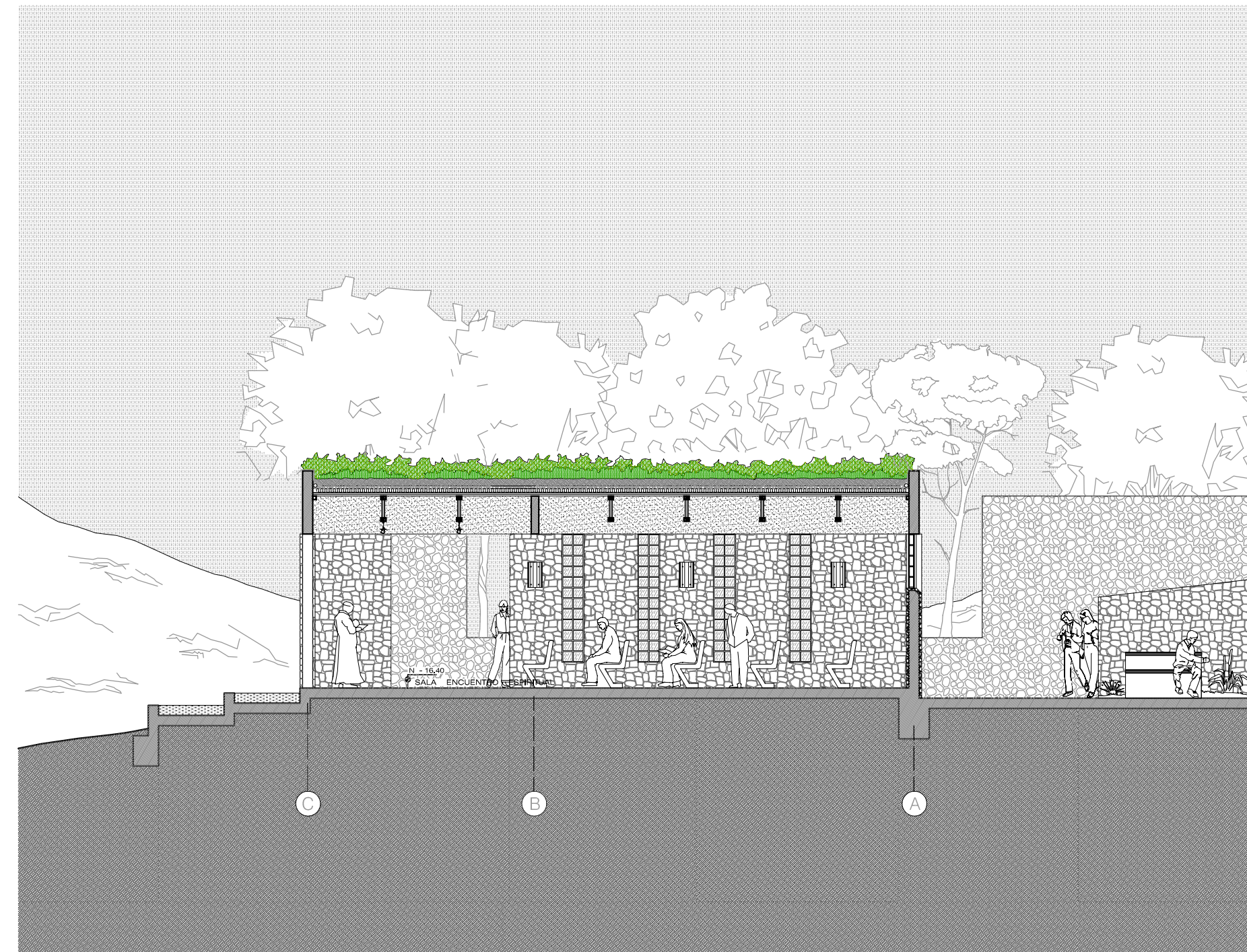
CORTE SALA DE ENCUENTRO ESPIRITUAL
