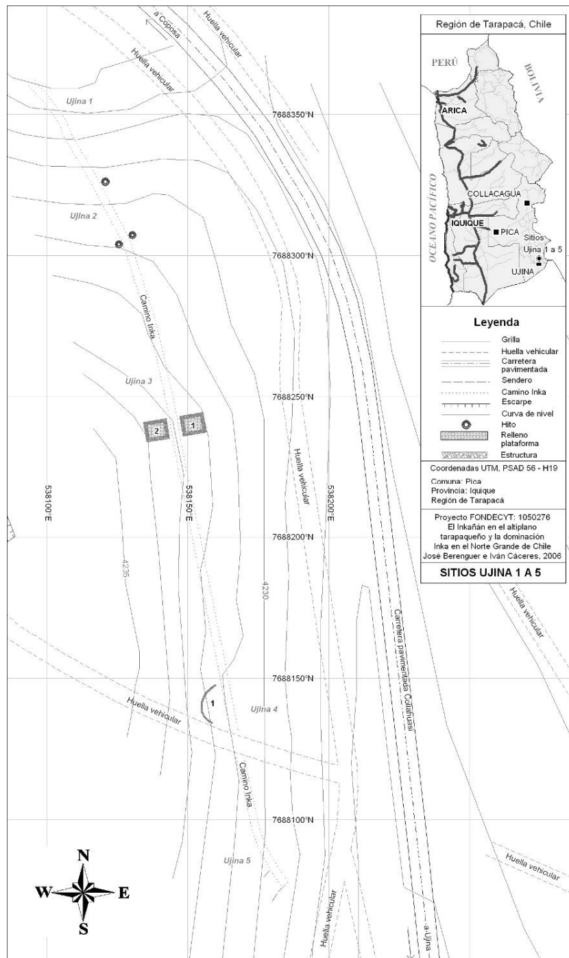
Fig. 22 Levantamiento topográfico segmento vial y plataformas en sector de Ujina (Berenguer et al 2011, figura 8).
