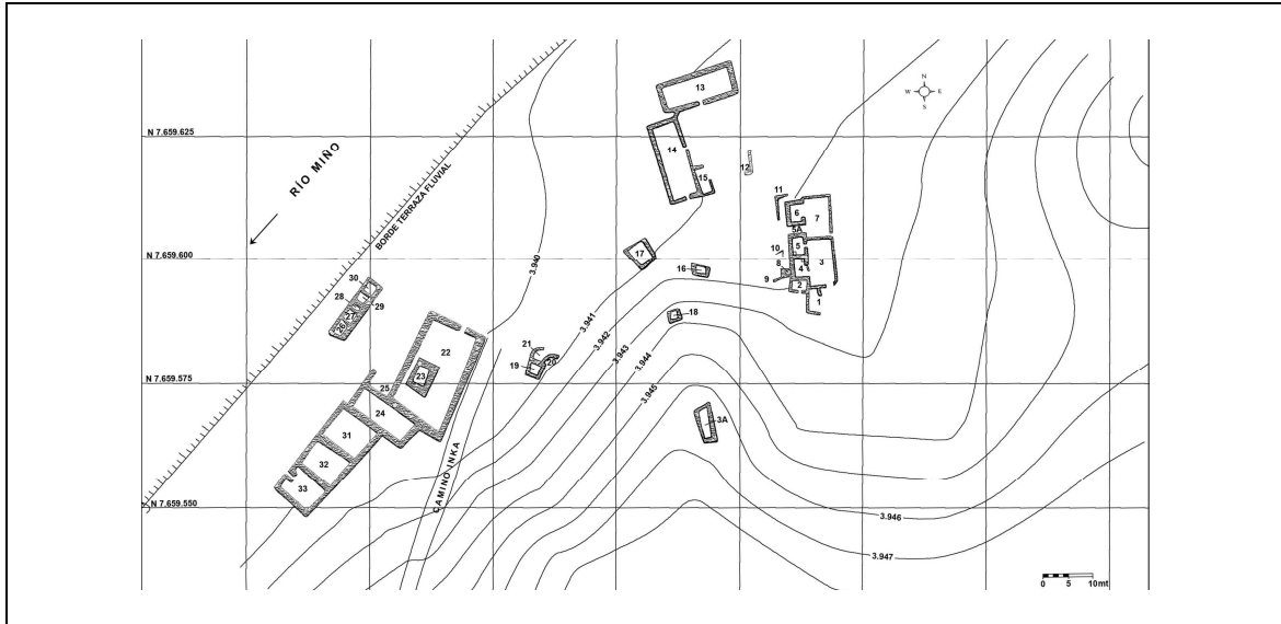
Fig. 30 Levantamiento topográfico de sitio MI2, sector Miño (Uribe y Urbina 2009, figura 10).
