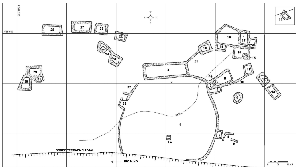
Fig.34 Levantamiento topográfico de sitio MI1, sector Miño (Uribe y Urbina 2009, figura 9).
