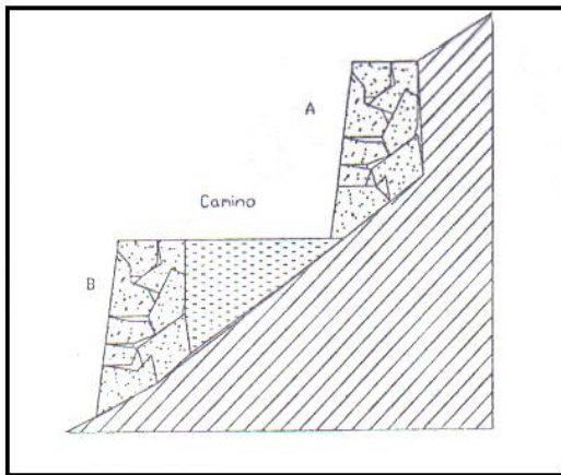
Figura 5. Muro de contención o retención
