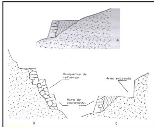
Figura 7. Camino tipo con talud
