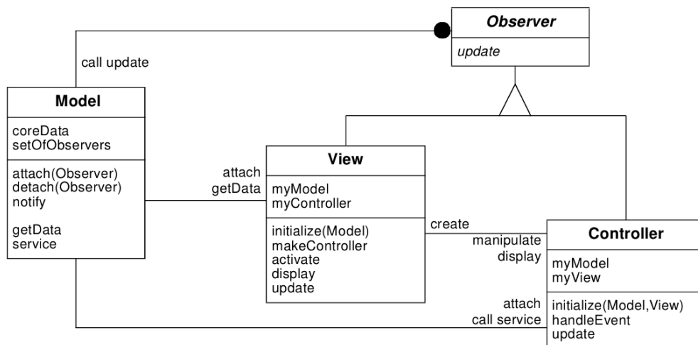
Figura 2.8: Diagrama de clases del patrón de diseño MVC. Fuente: A System of Patterns. Pattern-Oriented Software Architecture [11].
