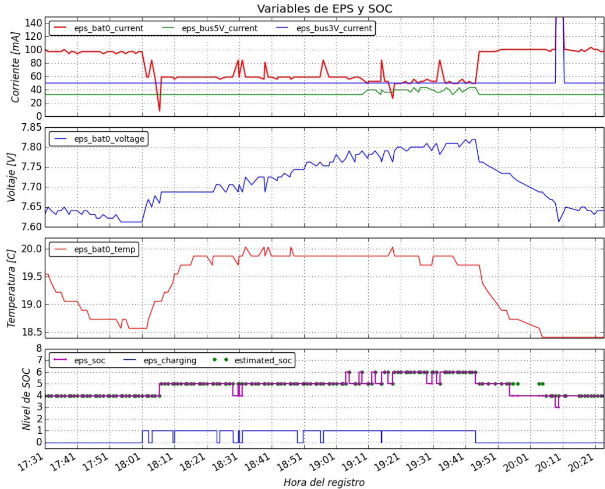
Figura 5.10: Gráfico con variables de EPS y estimación de SOC. El sistema de energía se comporta según lo esperado, según lo indicado por las variables de corriente y voltaje. Se observa una correspondencia entre la variable eps_charging y el voltaje de las baterías. El nivel de SOC estimado por el software de vuelo corresponde a los calculados a posteriori.
