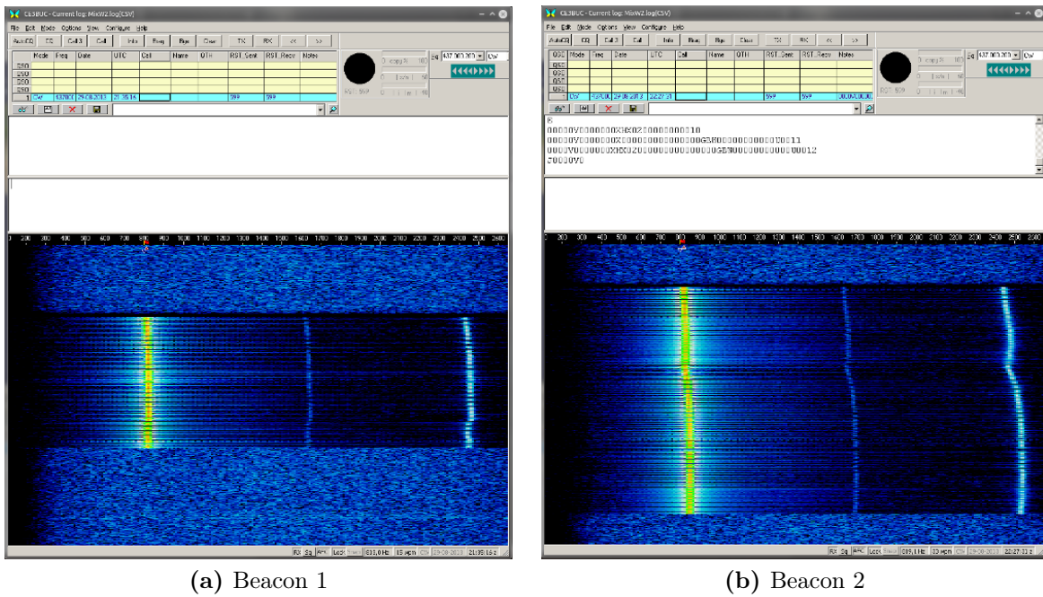
Figura 5.5: Beacon recibido en la estación terrena. Se utiliza el software MixW para decodificar una transmisión de radio demodulada por la estación terrena.
