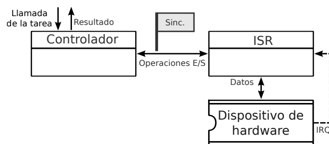
Figura 3.4: Arquitectura para controladores síncronos.
