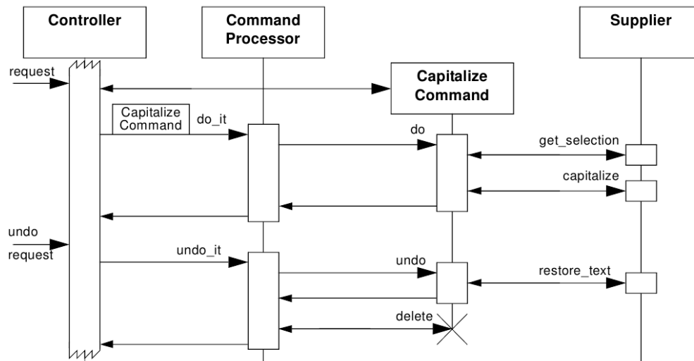
Figura 2.11: Esquema de colaboración del patrón de diseño procesador de comandos. Fuente: A System of Patterns. Pattern-Oriented Software Architecture [11].
