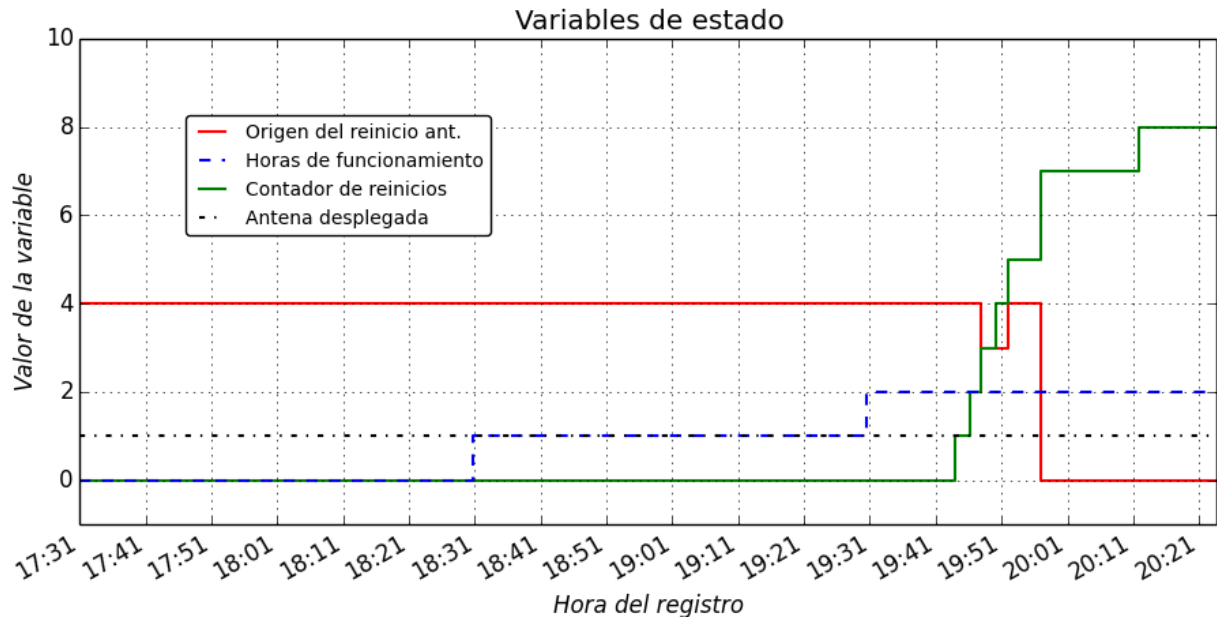
Figura 5.9: Variables de estado ante un reinicio. El repositorio de estados mantiene consistente el valor de las variables ante fallas o reinicios.
