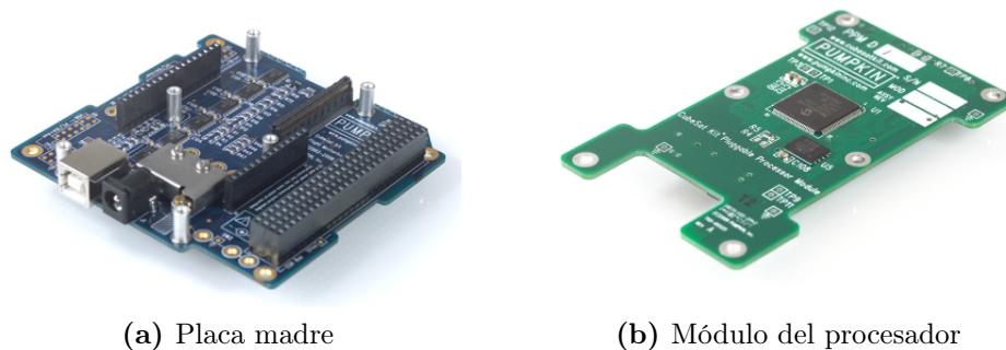
Figura 3.2: Dos módulos que componen el computador a bordo del satélite. A la izquierda, la placa madre que incluye un conector PC104. En la derecha un microcontrolador PIC24FJ256GA110. Fuente: http://www.cubesatkit.com/ .
