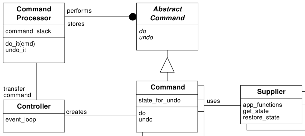
Figura 2.10: Diagrama de clases del patrón de diseño procesador de comandos. Fuente: A System of Patterns. Pattern-Oriented Software Architecture [11] .
