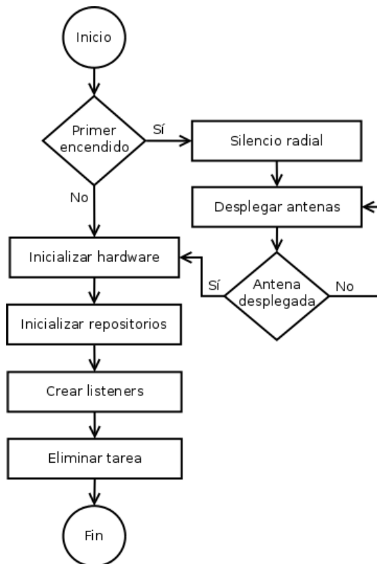
Figura 4.13: Diagrama de flujo para taskDeployment .
