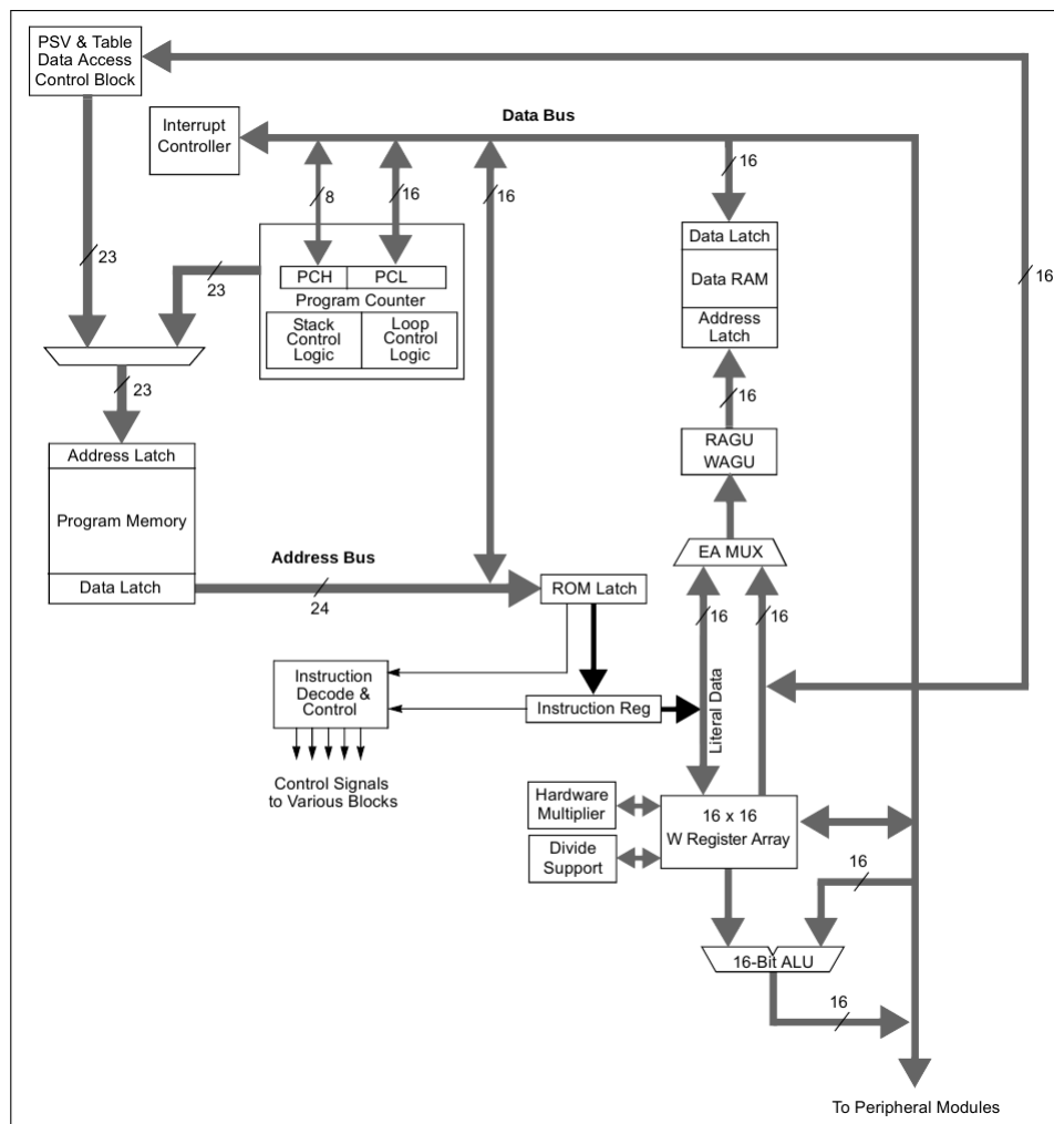
Figura 2.1: Arquitectura de la CPU del PIC24F. Fuente: PIC24F Family Reference Manual [7].
