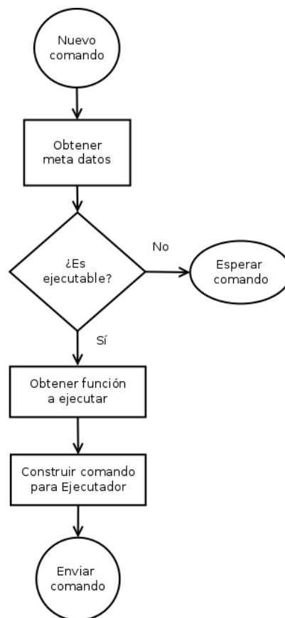
Figura 4.6: Diagrama de flujo para dispatcher .
