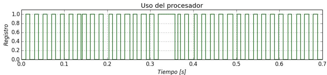
Figura 5.1: Registro de uso del procesador. El registro cambia de 0 a 1 cada vez que se entra en estado idle . Si no hay tareas que ejecutar esto ocurre cada 100 ms, de otro modo se observan periodos más largos.
