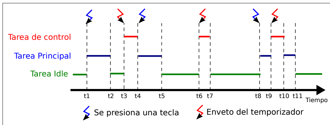
Figura 2.4: Real time scheduling. En un sistema operativo de tiempo real las interrupciones deben ser atendidas sin retrasos y las operaciones de cambio de contexto se realizan en un tiempo constante e independiente de la cantidad de tareas presentes.
