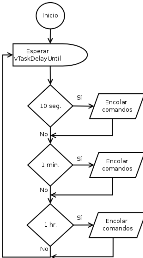
Figura 4.9: Diagrama de flujo para housekeeping.
