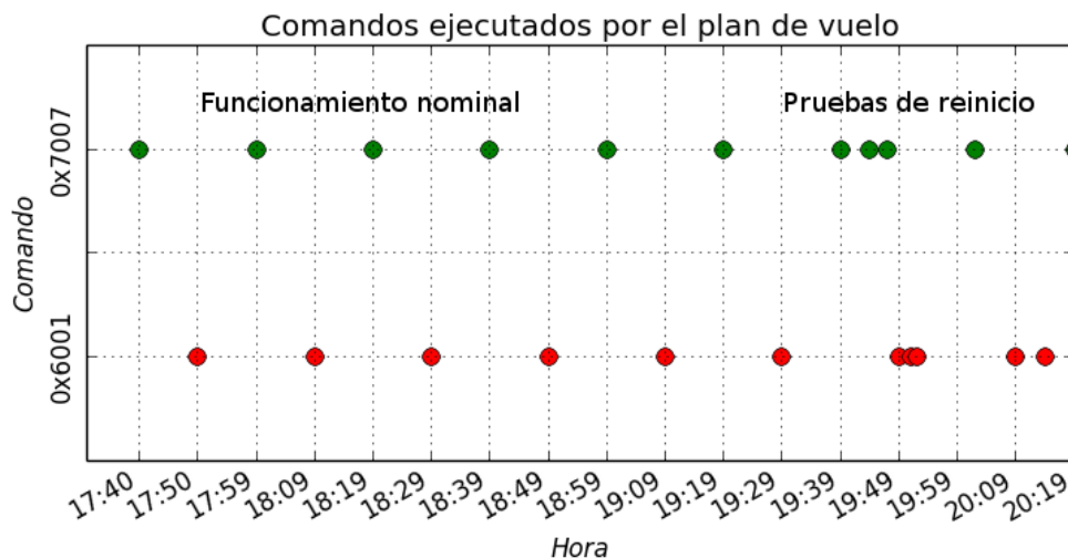
Figura 5.7: Gráfico de funcionamiento del plan de vuelo. Se observan los dos comandos programados ejecutándose cada 10 minutos. Cerca de las 19:39 hrs. se produce un reinicio del sistema y como respuesta a la falla, el plan de vuelo ejecuta el comando pendiente.
