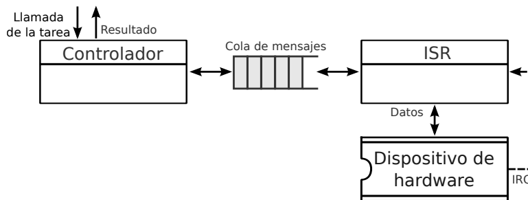
Figura 3.5: Arquitectura para controladores asíncronos.
