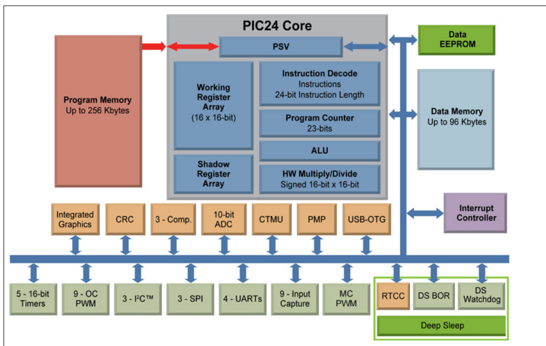
Figura 2.2: Periféricos del PIC24F. Además de la CPU, el PIC24F consta de una serie de periféricos. Fuente: Microchip, http://www.microchip.com/pagehandler/en-us/family/16bit/architecture/pic24f.html .
