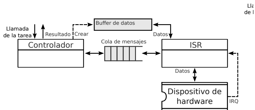
Figura 3.6: Arquitectura de un controlador de entrada serial asíncrono.
