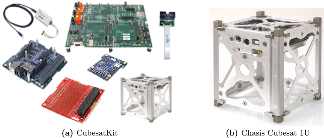
Figura 3.1: CubesatKit de Pumpkin Inc. A la izquierda, los componentes del kit, que incluye una placa de desarrollo, procesador, programador y la estructura del satélite. En la derecha la estructura metálica de un Cubesat de una unidad. Fuente: http://www.cubesatkit.com/ .
