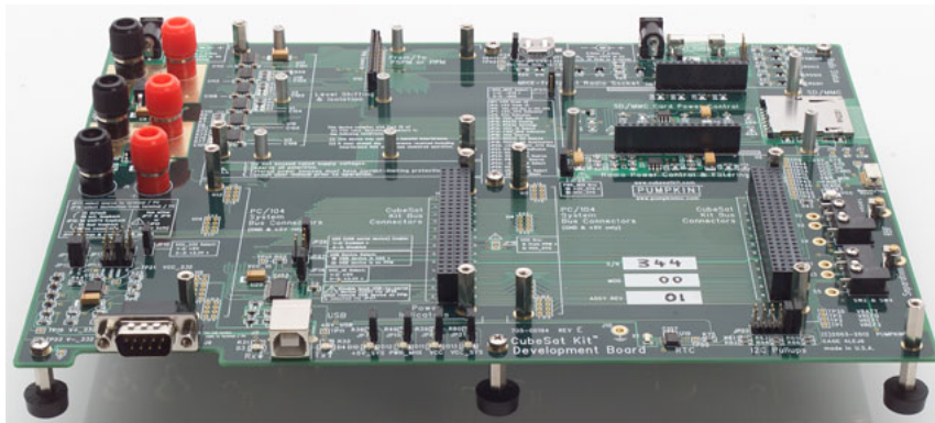
Figura 4.2: Tarjeta de desarrollo para Cubesat Kit de Pumpkins. Es eléctricamente igual a la placa madre del computador abordo del satélite. Permite conecta un módulo de procesador al bus PC104, cuenta con un conector de memoria SD, conversor RS232 a USB, alimentación y protección de sobre corriente.
