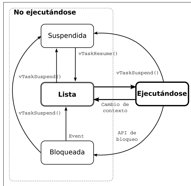
Figura 2.5: Tareas de FreeRTOS, diagrama de estados.
