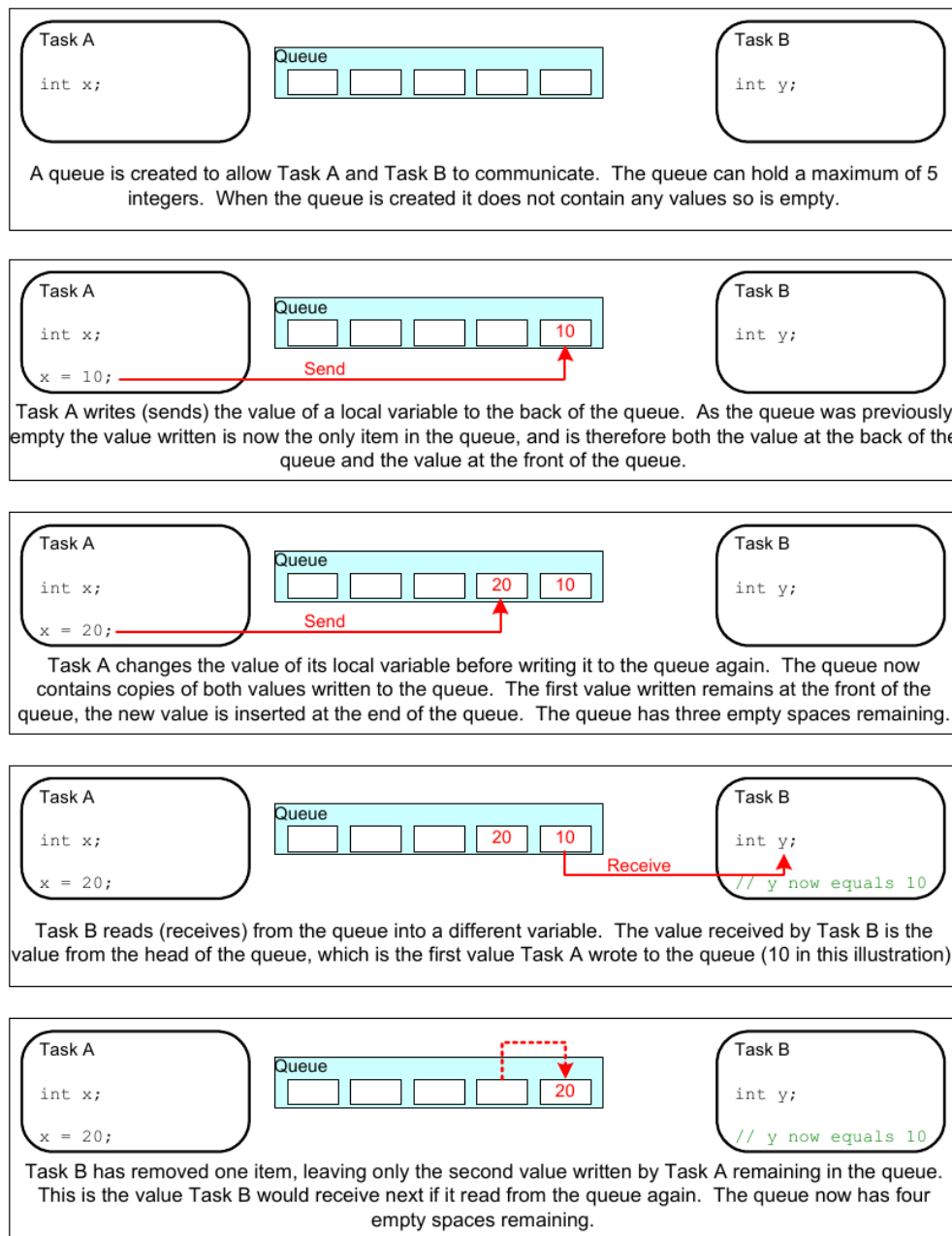
Figura 4.5: FreeRTOS Queue. Permiten el acceso sincronizado a datos en una cola, para la comunicación entre tareas. Se crean con un tamaño fijo y los elementos son almacenados por copia. Fuente: http://www.freertos.org/Embedded-RTOS-Queues.html
