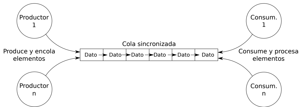
Figura 4.4: Problema del productor-consumidor. Múltiples productores almacenan datos en una cola, la cual también es accedida por múltiples consumidores. Para evitar condiciones de data race el acceso a los datos debe estar sincronizado.
