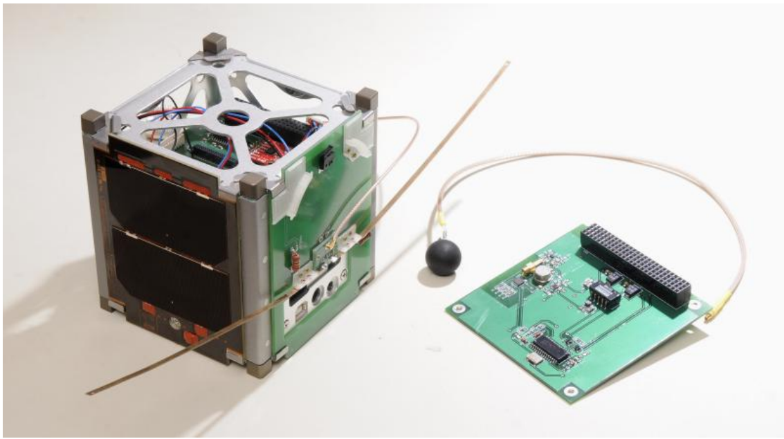
Figura 2.15: Satélite SUCHAI junto a una langmuir probe. Imagen tomada durante etapas tempranas de integración.
