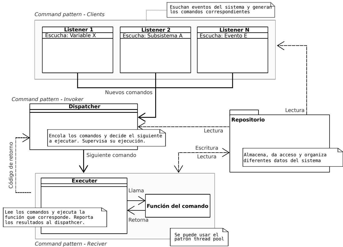
Figura 3.7: Arquitectura del software de vuelo en la capa de aplicación.. Corresponde a una adaptación de command pattern .
