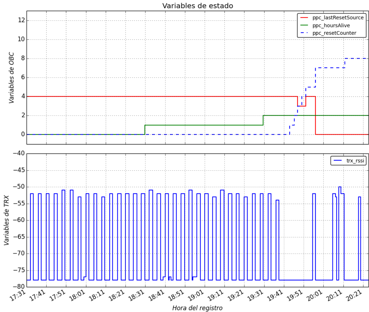
Figura 5.8: Gráfico con el valor de las variables de estado en el tiempo. Arriba, variables relacionadas con el computador a bordo. Abajo, el valor del Received Signal Strength Indicator (RSSI) del transceiver, los máximos coinciden con las transmisiones de beacon.
