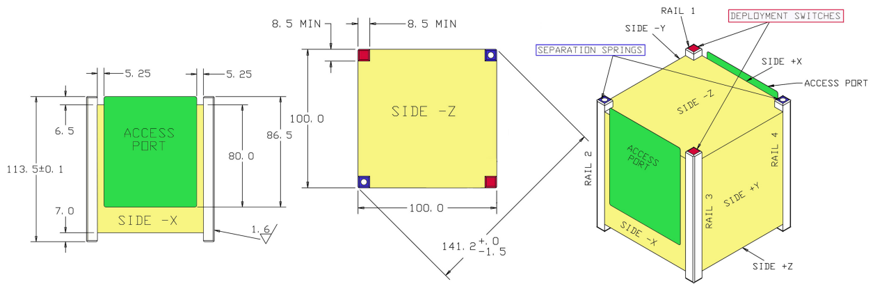
Figura 2.13: Especificaciones de diseño del estándar Cubesat de una unidad. Fuente: http://www.cubesat.org/index.php/documents/developers .
