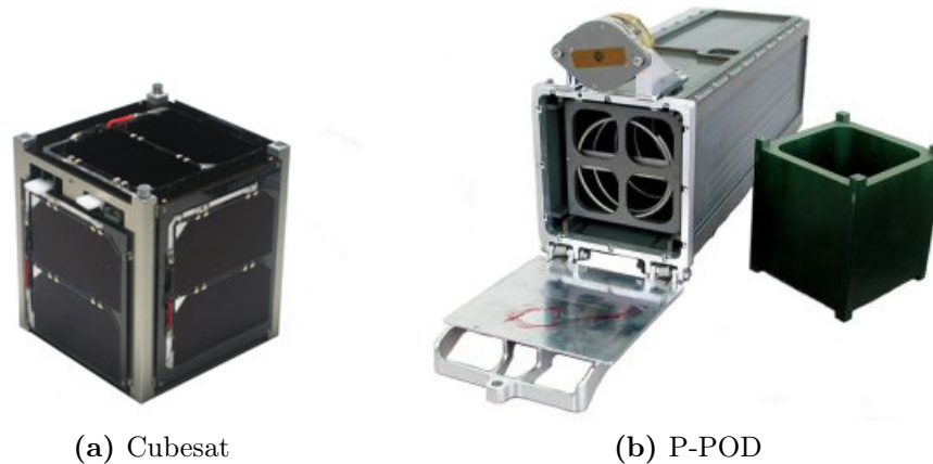
Figura 2.12: Satélite tipo Cubesat. A la izquierda el satélite japonés OSCAR-66, lanzado el año 2008. A la derecha un P-POD, dispositivo desde el cual se despliega un Cubesat. Fuente: http://cubesat.aero.cst.nihon-u.ac.jp/english/index.html
