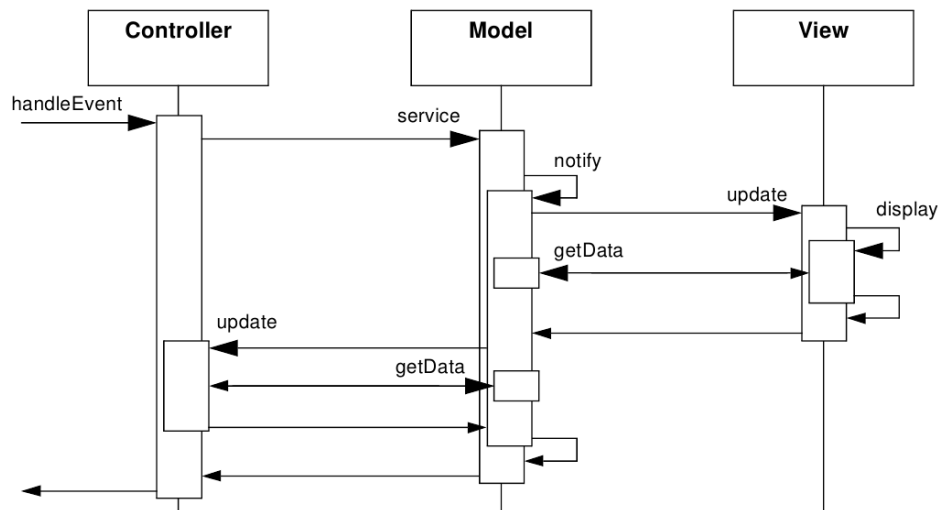
Figura 2.9: Esquema de colaboración del patrón de diseño MVC. Fuente: A System of Patterns. Pattern-Oriented Software Architecture [11].
