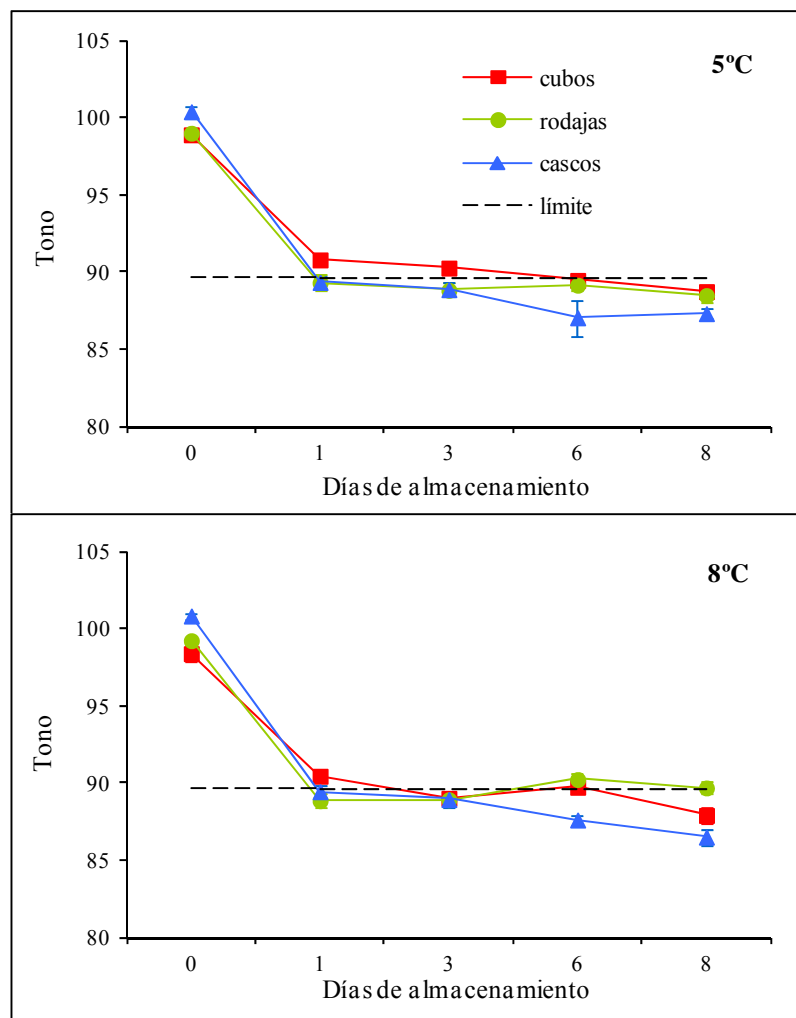
Figura 7. Evolución del tono ( H_{ab} ) de manzanas “Red Delicious” aplicando tipos de cortes (cascos, cubos y rodajas) y temperaturas de almacenamiento (5 y 8°C). Medias ( n=3 ) con error estándar.
