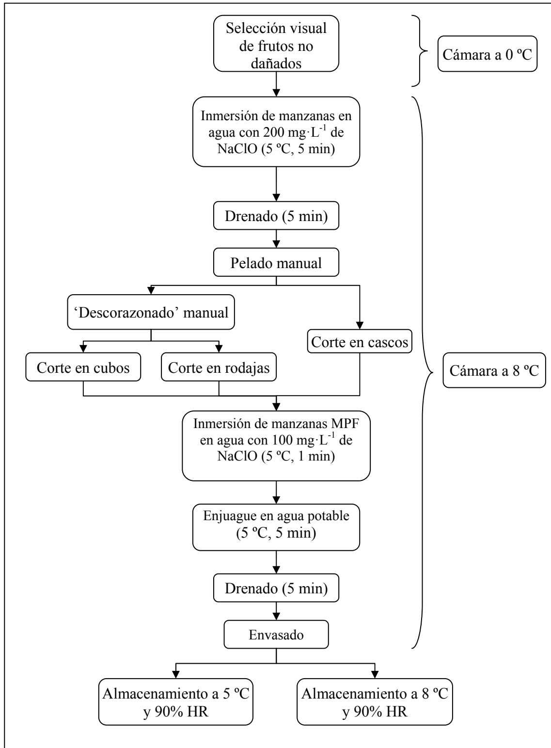
Figura 1. Línea de proceso para manzanas ‘Red Delicious’ y ‘Cripps Pink’ MPF.
