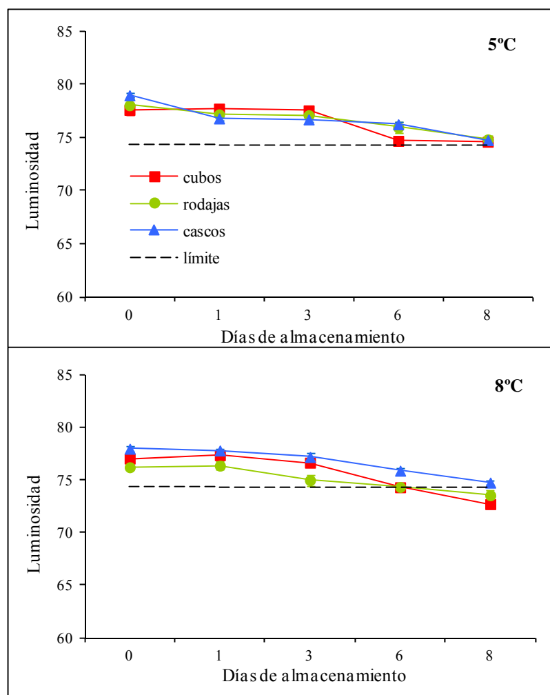
Figura 15. Evolución de la luminosidad (L) de manzanas “Cripps Pink” aplicando tipos de cortes (cascos, cubos y rodajas) y temperaturas de almacenamiento (5 y 8°C). Medias (n=3) con error estándar.
