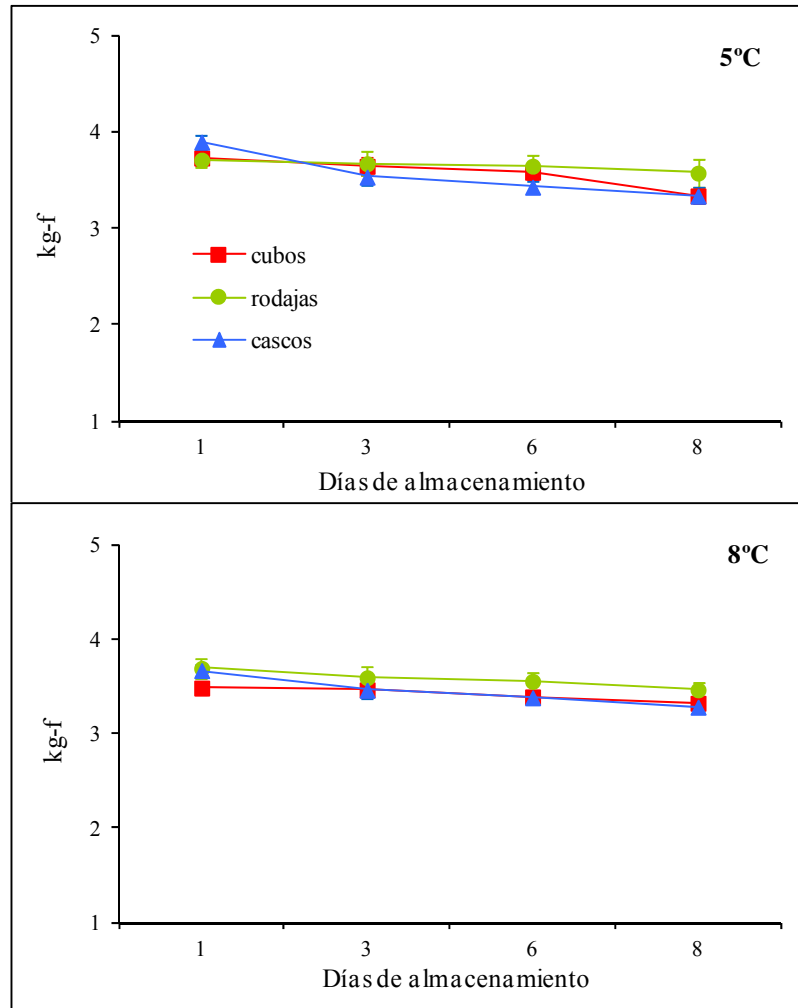
Figura 18. Evolución de la firmeza (kg-f) de manzanas “Cripps Pink” aplicando tipos de cortes (cascos, cubos y rodajas) y temperaturas de almacenamiento (5 y 8°C). Medias (n=3) con error estándar.
