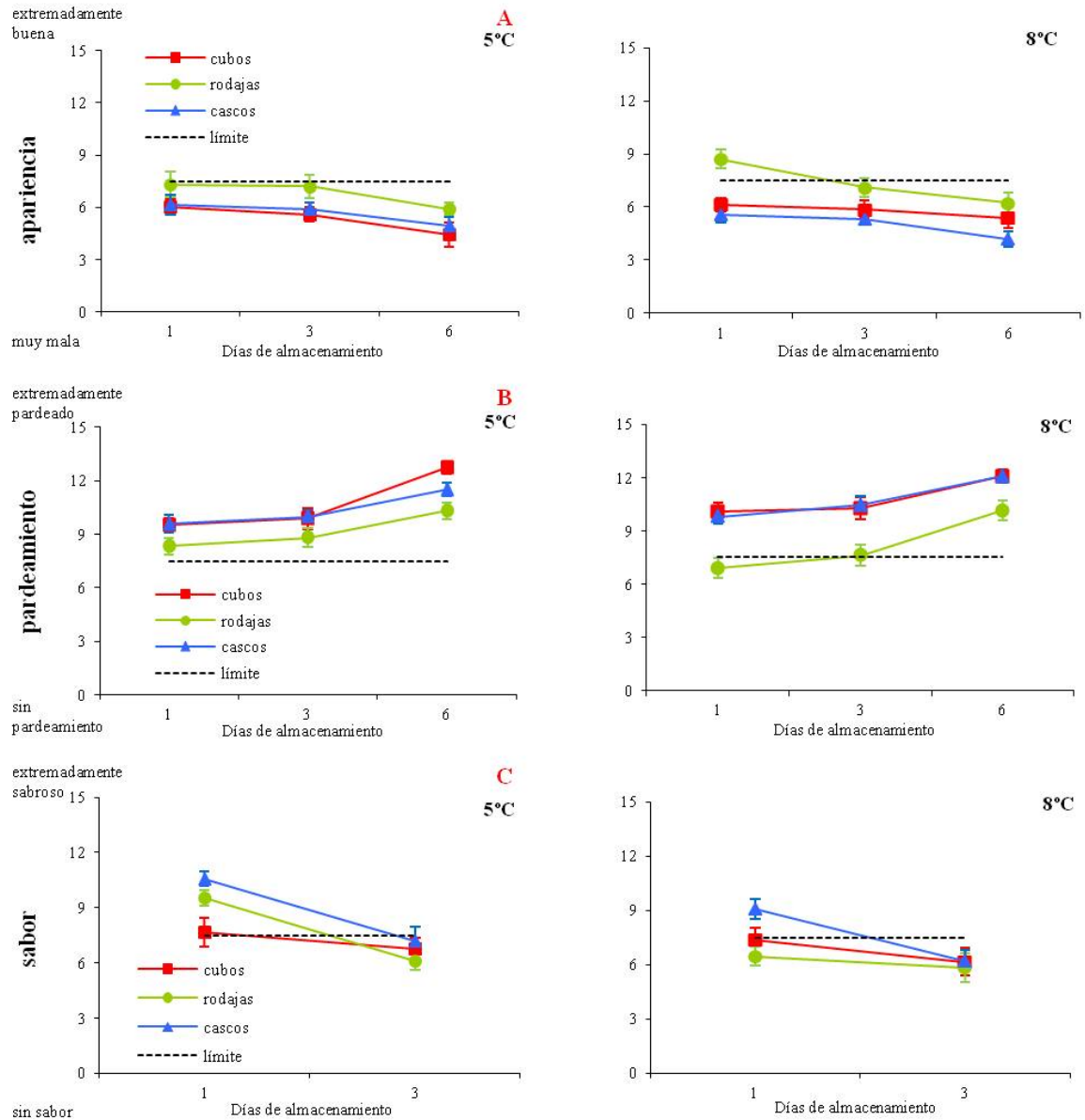
Figura 13. Evolución de diferentes parámetros sensoriales en manzanas “Red Delicious” aplicando tipos de cortes (cascos, cubos y rodajas) y temperaturas de almacenamiento (5 y 8°C). Apariencia (A), pardeamiento (B) y sabor (C). Apariencia: 0=muy mala; 7,5=me es indiferente; 15=extremadamente buena. Pardeamiento: 0=sin pardeamiento; 15=extremadamente pardeado. Sabor: 0= sin sabor; 15=extremadamente sabroso. Medias (n=12) con error estándar.
