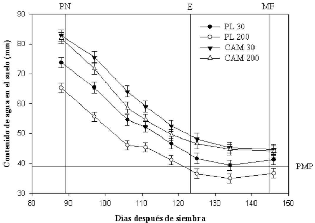
Figura 4. Balance hídrico durante de los ensayos plano (PL) y camellón (CAM) de las dosis de semilla 30 y 200 Kg ha -1 . PN: Primer nudo; E: Espigadura; MF; Madurez fisiológica; PMP: Punto de marchitez permanente. Las Barras corresponden al error estándar de la media de la media.
