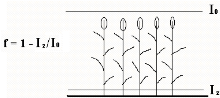
Figura 3. Esquema de medición del PARi donde f es la fracción de radiación incidente que es interceptada por el cultivo desde 0 a z.
