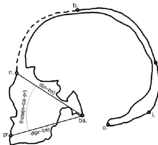
Figura 4.2: Sección transversal de un cráneo humano, mostrando los distintos tipos de datos morfométrico e.g. distancia (ba-n), contorno (b-n), ángulo (theta(n-ba-pr)) y coordenadas: b.— bregma, n.—nasion, pr.—prosthion, ba.— basion, o.—opisthion, i.—inion, l.—lambda. (Slice 2005).
