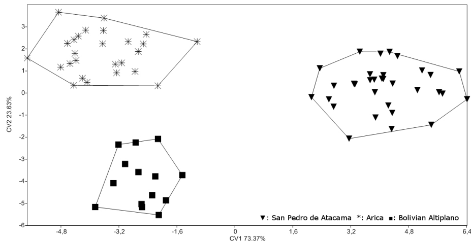
Figura 3.2: Análisis Canónico Sincrónico entre diferentes poblaciones del Período Medio de la Región Andina. ▼ : San Pedro de Atacama; * : Arica; ■ : Altiplano Boliviano. La figura muestra dos ejes canónicos que dan cuenta del 73.37 % y 23.63 % de la varianza inter-grupal respectivamente. Las distancias de Mahalanobis fueron altamente significativas tras 10,000 rondas de permutación. Comparaciones pareadas de Hottelling T2 con corrección de Bonferroni confirman este resultado mostrando diferencias significativas entre los grupos ( p < 0.0001 ).
