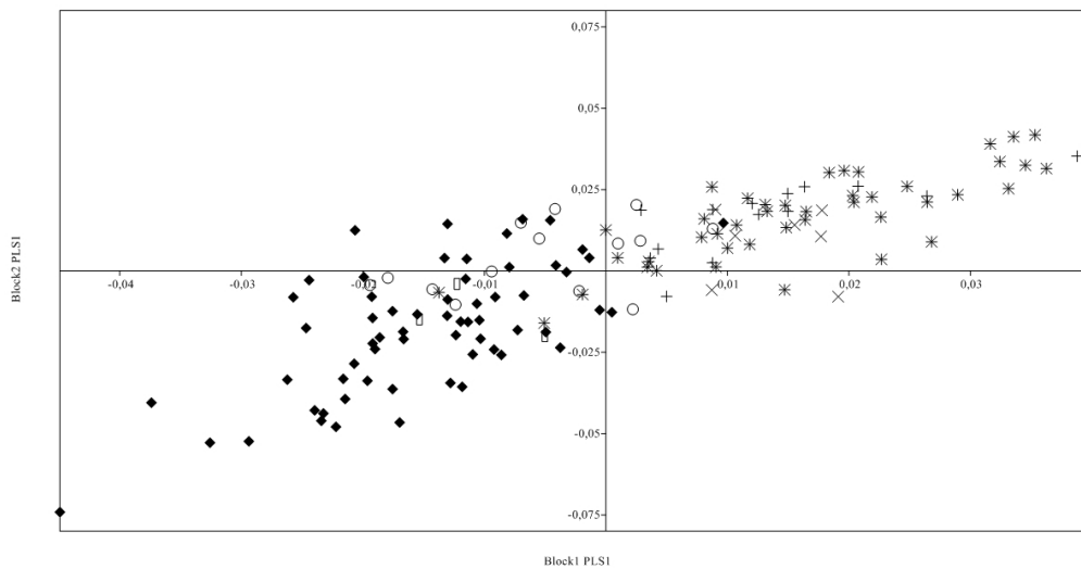
Figura 3.5: Gráfico de correlación para el PLS1 para los dos módulos (neurocráneo y esplanocráneo) en Individuos Deformados.
