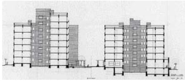
Fig.20. Corte transversal. A la iz. calle de Gaztambide, a la der. calle de Hilarión Eslava. Fte.: Biblioteca Nacional de España, 2006, op. cit. Reproducción con fines estrictamente culturales.
