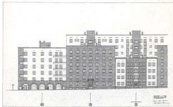
Fig.17. Elevación parcial de la Casa de las Flores, calle de Gaztambide. Fte.: COAM, 1983, op.cit. Reproducción con fines estrictamente culturales.
