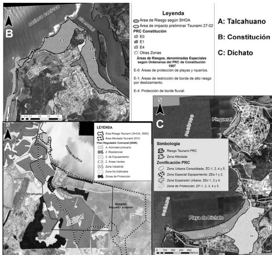
Figura 3. Zonas de riesgo de tsunamis y planes reguladores comunales de A) Talcahuano, B) Constitución y C) Dichato. Fuente: elaboración propia con base en PRC Talcahuano (2006), Constitución (1987) y Tomé (2008), cartas de riesgo de Tsunami del SHOA (2000) e imágenes Google Earth (2010).
