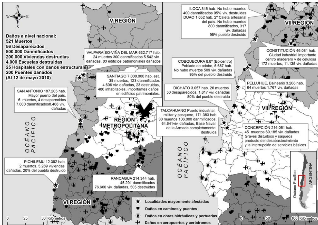
Figura 1. Regiones y ciudades afectadas y principales daños producidos por el terremoto y tsunami del 27 de febrero de 2010 en Chile. Fuente: elaboración propia con base en información del Sistema Nacional de Coordinación de Información Territorial (SNIT), periódico El Mercurio y el Sistema Integrado de Información Territorial (SIIT) del Congreso Nacional.
