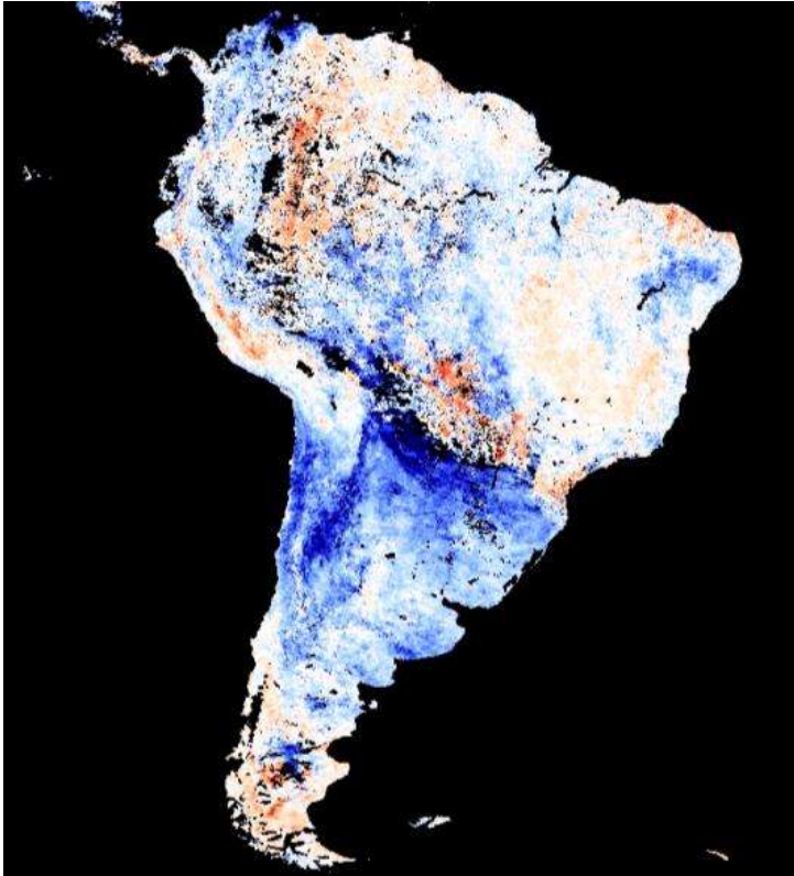
Figura 4. Desplazamiento de los sistemas atmosféricos centrales y localización de las anomalías negativas de temperatura (color azul) registradas en América del Sur entre 12 e 19 de julio de 2010, comparadas con las medias del período 2000-2008, según NASA.
