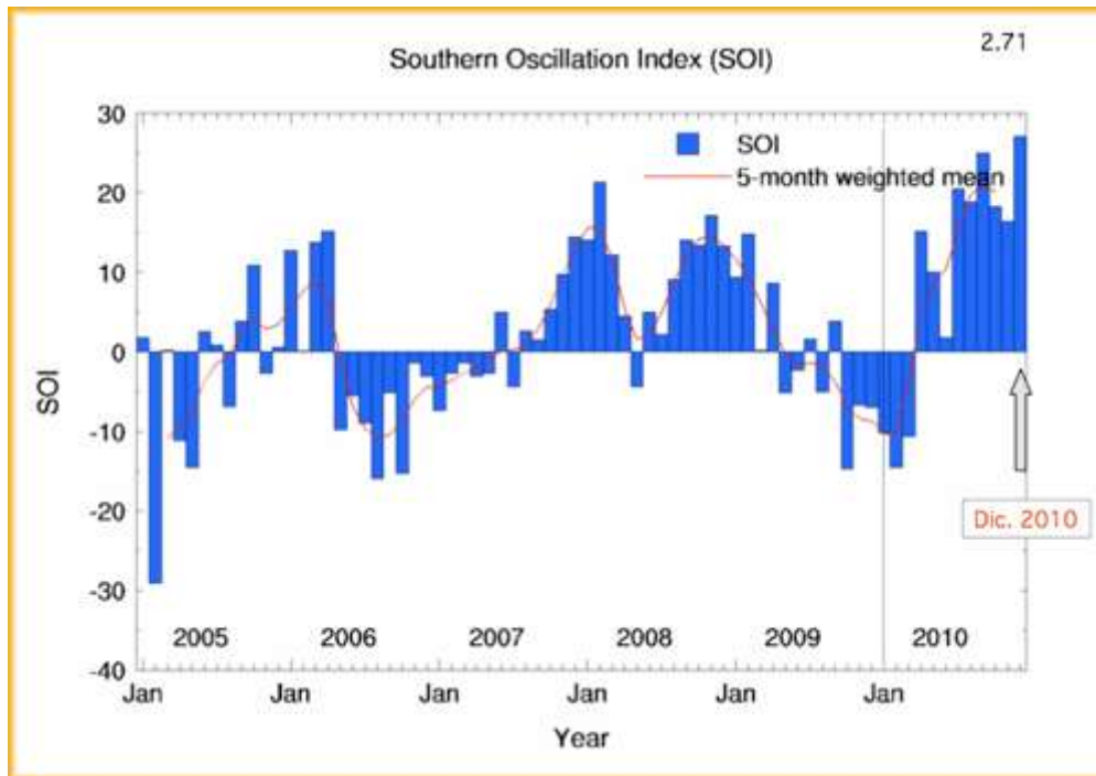
Figura 1: Índice de Oscilación del Sur entre enero de 2005 y diciembre de 2010. Fuentes: Bureau of Meteorology – Australia ; Boletín Climático de Chile , Departamento de Geofísica de la Universidad de Chile , enero 2011.
