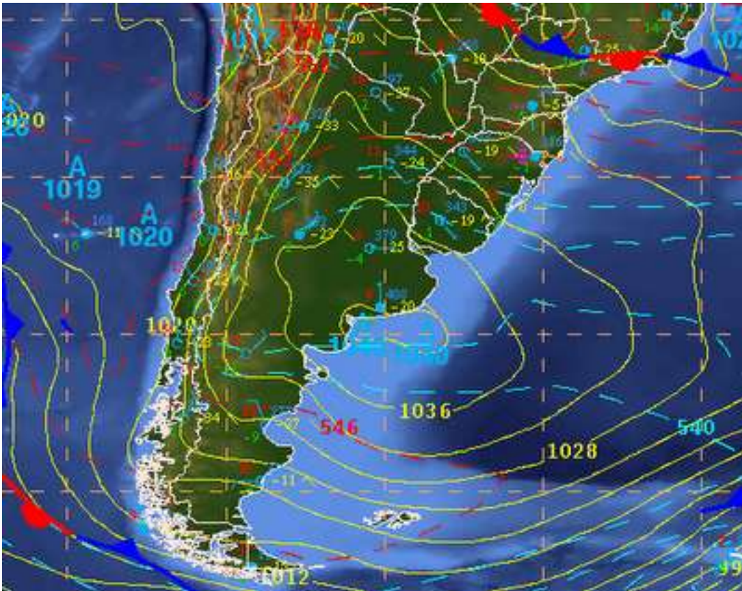
Figura 5: Distribución de las presiones atmosféricas promedio en Sudamérica en julio de 2010.
