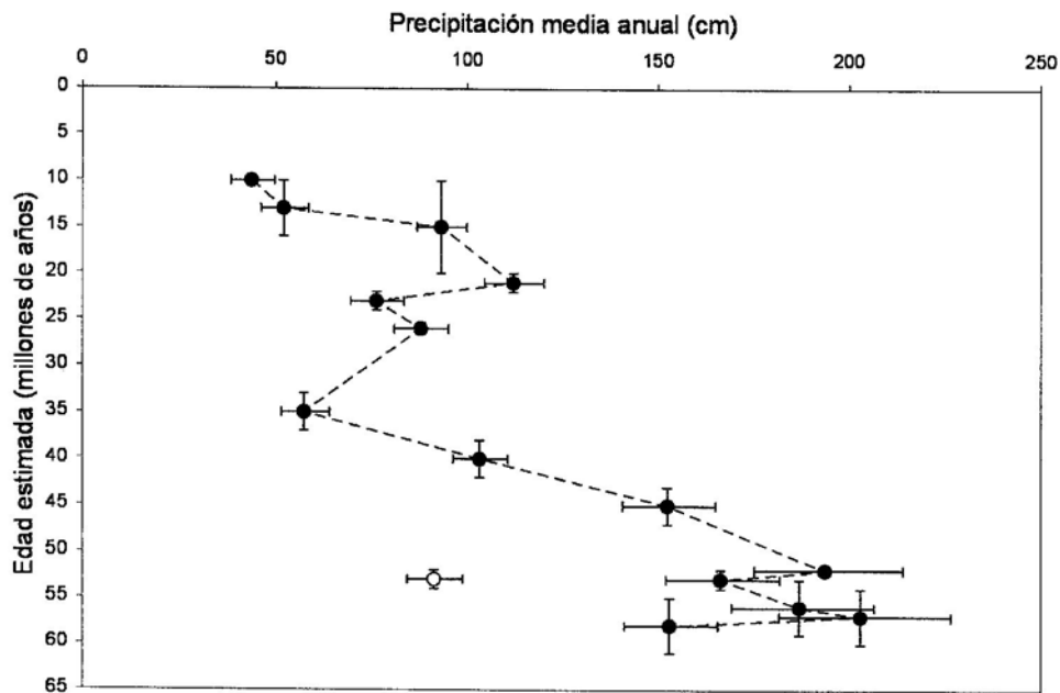
FIG. 4-. Variación de la precipitación media anual a través del Cenozoico del sur de Sudamérica, de acuerdo al modelo univariado y usando como variable dependiente el Ln del área foliar. Las barras en el eje de las precipitaciones indican el intervalo de confianza al 95% (los intervalos son diferentes ya que fueron obtenidos a partir de logaritmos).
