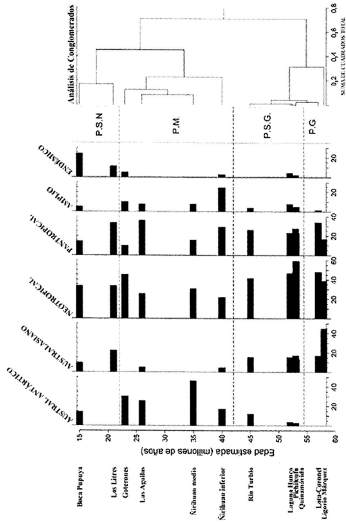
FIG. 7. Distribución de elementos fitogeográficos en las tafofloras cenozoicas consideradas en este trabajo. P.G: Paleoflora Subtropical Gondwánica; P.M.: Paleoflora Mixta; P.S.N.: Paleoflora Subtropical Neogena.
