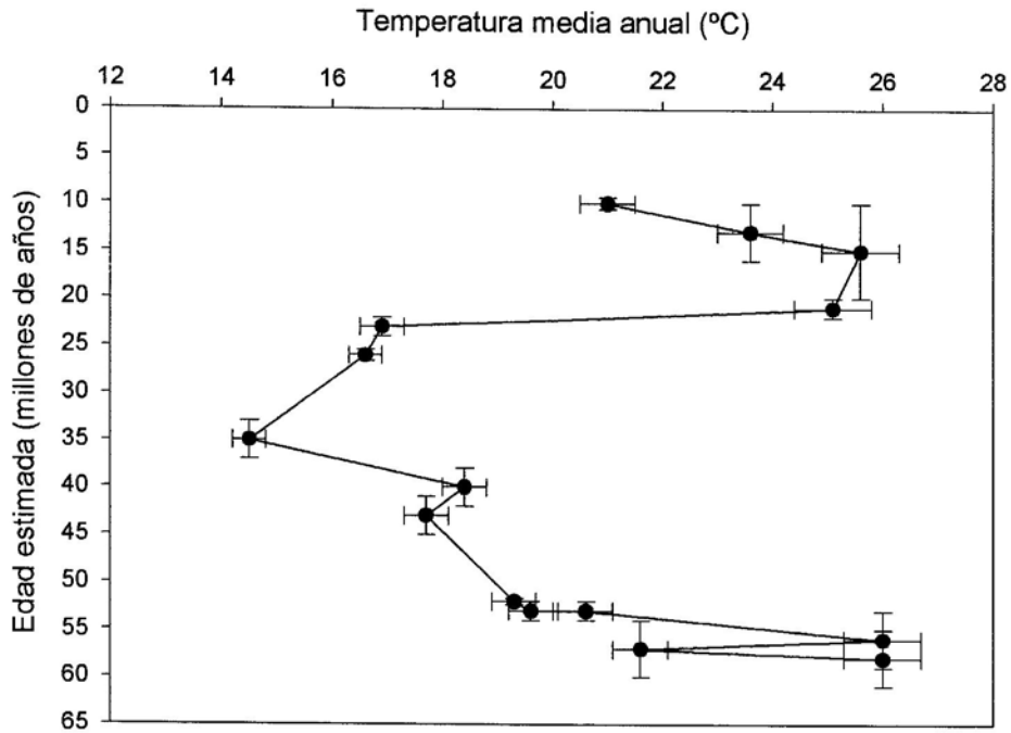
FIG. 2. Variación de la temperatura media anual a través del Cenozoico del sur de Sudamérica, de acuerdo al modelo univariado. Las barras en el eje de las temperaturas indican el intervalo de confianza al 95%.
