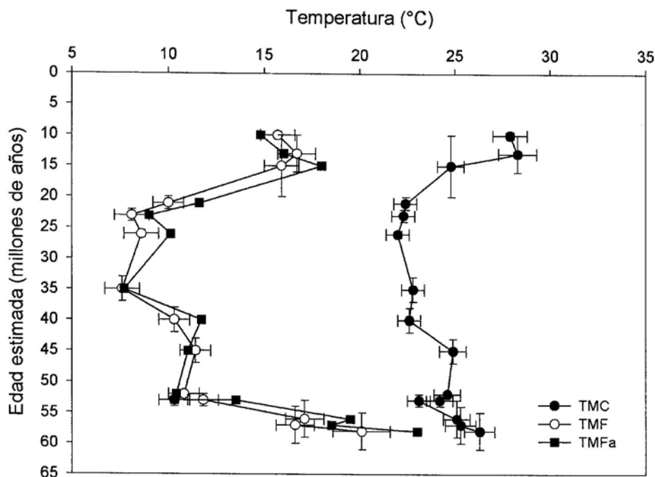
FIG. 6. Temperaturas medias del mes más frío (TMF, círculos blancos, y TMFa, cuadrados negros) y del mes más cálido (TMC, círculos negros) a través del Cenozoico del sur del Sudamérica. Las barras en el eje de las temperaturas indican el intervalo de confianza al 95%. Los valores fueron obtenidos a partir del análisis de correspondencia canónica (TMF y TMC) y de acuerdo a J. Wolfe (TMFa, comunicación oral, 2002).
