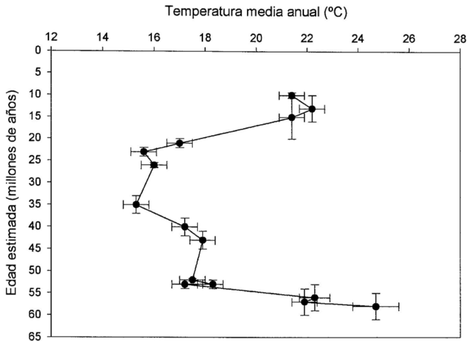
FIG. 3. Variación de la temperatura media anual a través del Cenozoico del Sur de Sudamérica, de acuerdo al modelo multivariado. Las barras en el eje de las temperaturas indican el intervalo de confianza al 95%.
