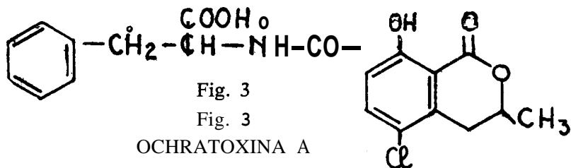
7-[N-(alfa-carboxi-beta-fenil-etil)-carbamil] -5-cloro-3-metil-8-hidroxibenzo[c] 1,Z-oxanona.
