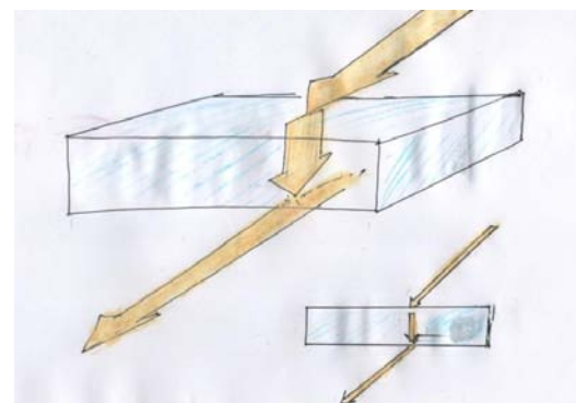
Un rayo de luz viene por el aire y cruza más rápido una zona densa (como vidrio o agua) cruzándola de ese modo con menos desgaste; cambiando luego su ángulo, sigue su camino por el aire retomando su ángulo original. Sabiduría de la naturaleza, economía natural.-
