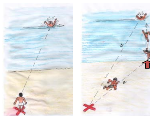
Caso N° 2: El observador ve al niño en peligro, corre hasta un punto adelantado porque la corriente está arrastrando al niño. Además, se corre más rápido por la arena que lo que se nada en el mar; Luego, se zambulle y nada recto al punto de encuentro. Se gana un tiempo vital, porque T_2 < T_1
