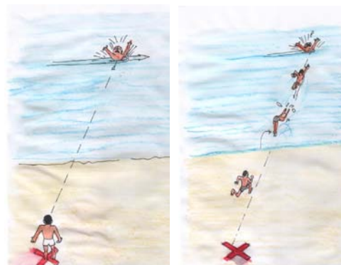
Caso N° 1: El observador ve al niño en peligro, corre derecho, se zambulle y nada derecho hacia su objetivo y se demora un tiempo “ T_1 ”
