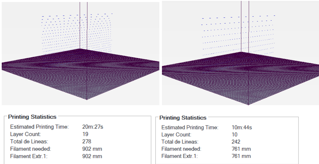
Figura 4-52 Izquierda: Experimento A y sus estadísticas de impresión. Derecha: Experimento B y sus estadísticas de impresión. Fuente: Elaboración Propia.
