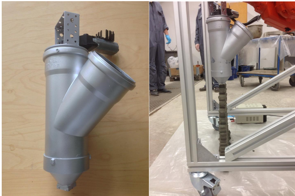
Figura 4-2 a) Extrusor modelo b) extrusor en funcionamiento. Fuente: (Anell, 2015)
