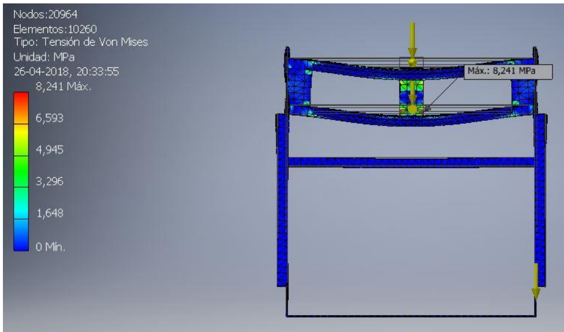
Figura 4-19 Resultados para el estudio de Tensión de Von Mises del diseño final del subsistema "Puente". Fuente: Elaboración propia
