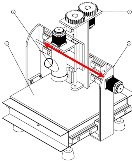
Figura 4-7 Esquema del desplazamiento en X. Fuente: Elaboración personal
