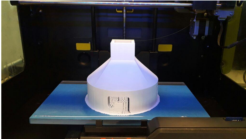
Figura 4-32 Boquilla finalizada. Fuente: Elaboración propia
