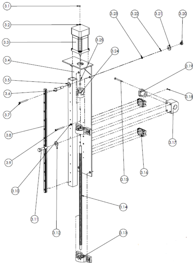
Figura 4-27 Explosiónado del subsistema Mesa Horizontal. Fuente: Elaboración propia
