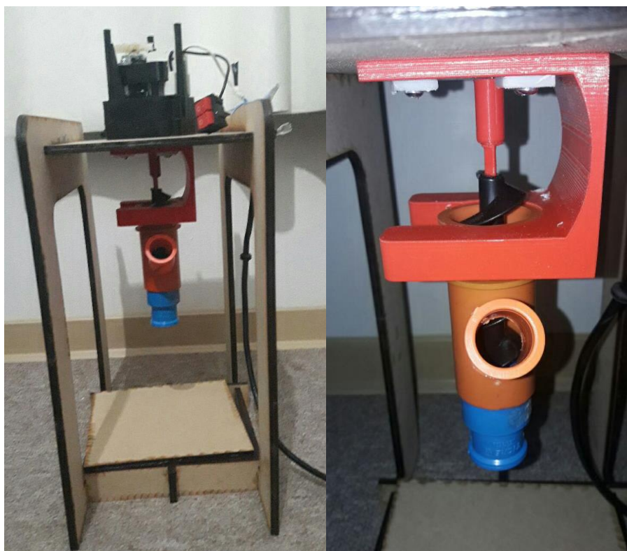
Figura 4-21 a) Maqueta del extrusor de concreto y su montaje. b) Vista enfocada al extrusor. Fuente: Elaboración propia
