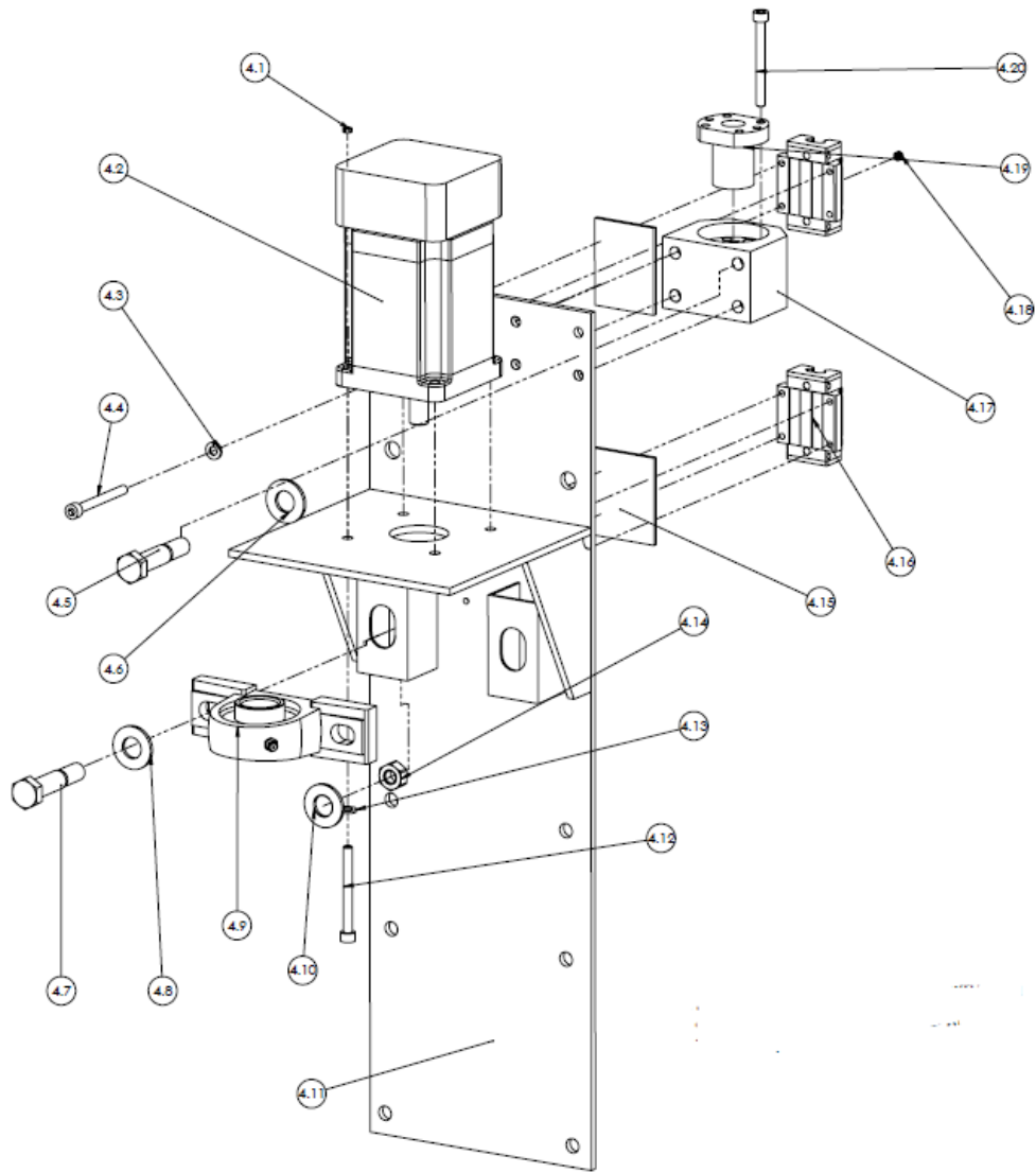
Figura 4-28 Explosionado del subsistema Porta Extrusor Fuente: Elaboración propia
