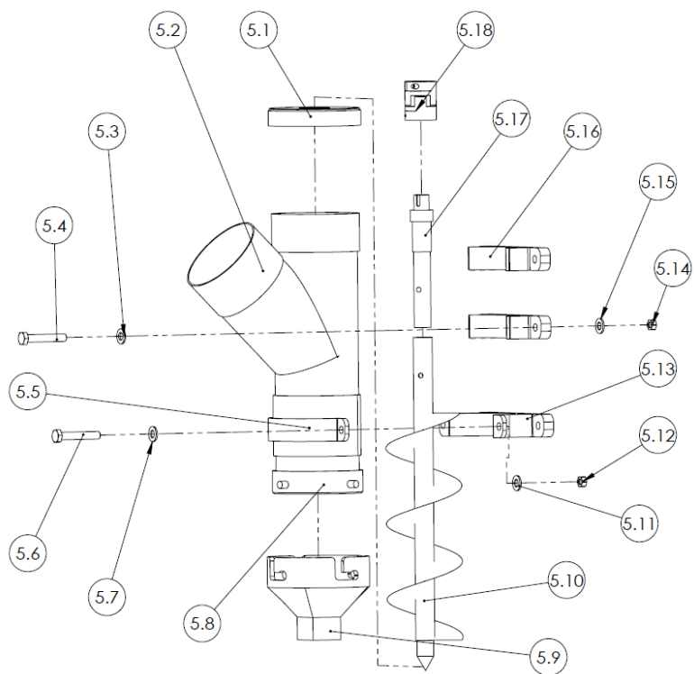
Figura 4-29 Explosionado del subsistema Extrusor Fuente: Elaboración propia
