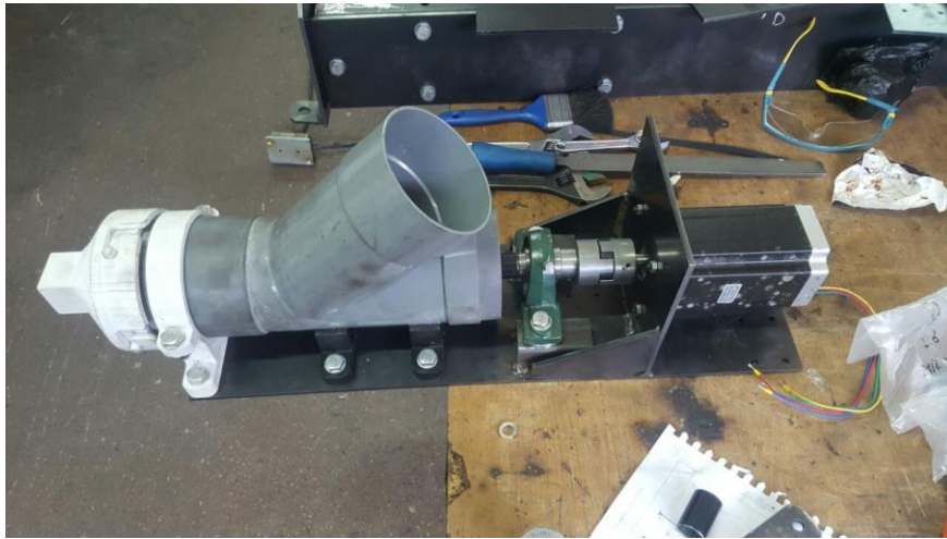
Figura 4-38 Extrusor y porta Extrusor. Fuente: Elaboración propia
