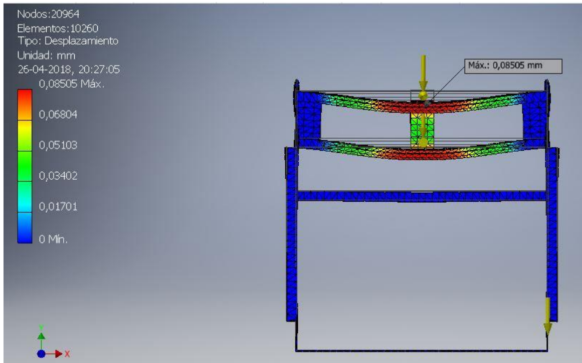
Figura 4-20 Resultados para el estudio de desplazamientos en el subsistema "Puente" del diseño final. Fuente: Elaboración Propia
