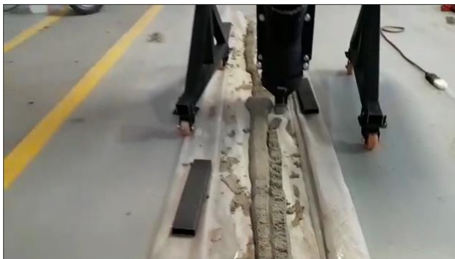
Figura 4-46 Muestra de extrusión con hormigón de alto porcentaje Agua/Concreto. Fuente: Elaboración propia
