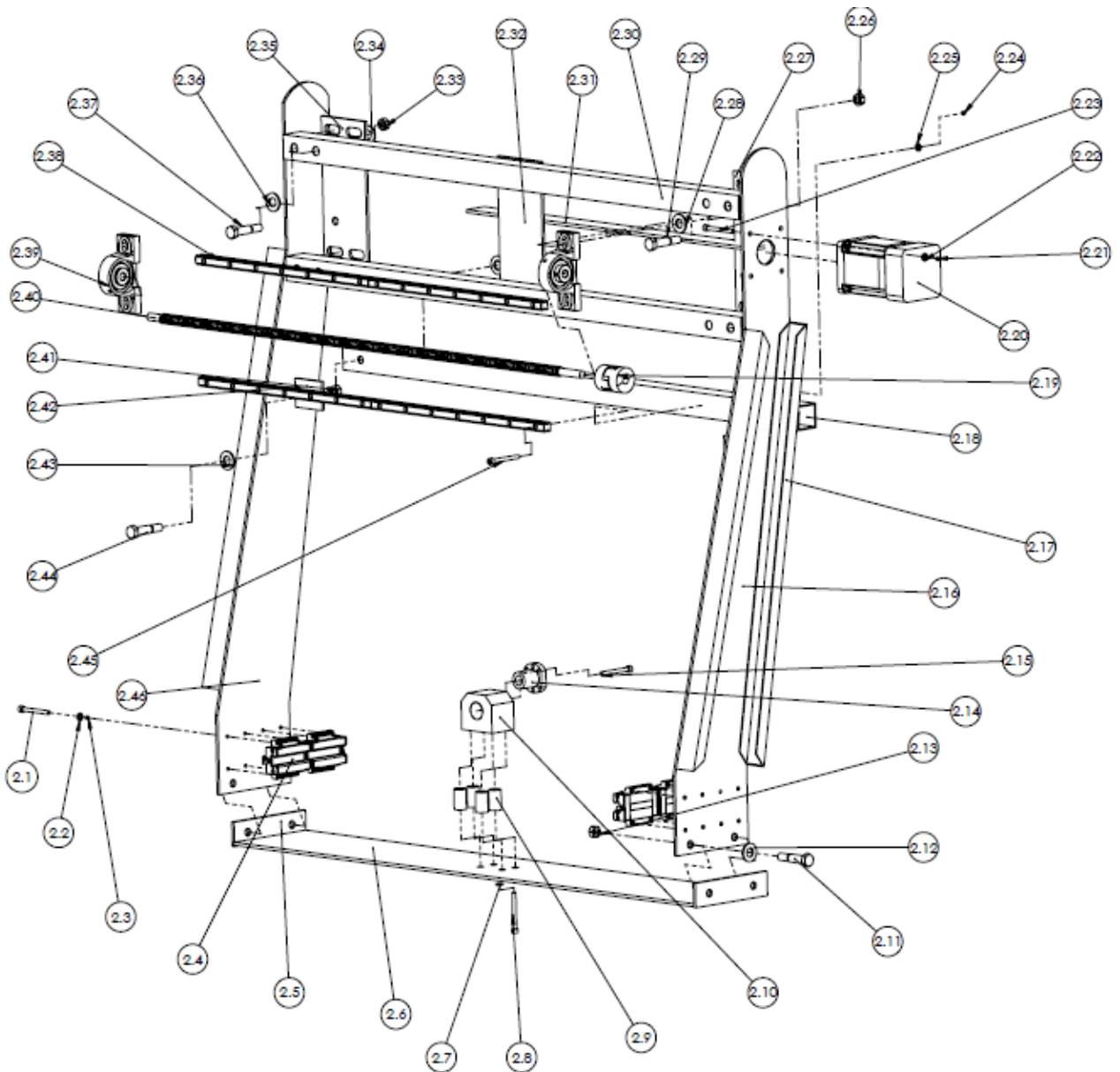
Figura 4-26 Explosionado del subsistema Puente. Fuente: Elaboración propia
