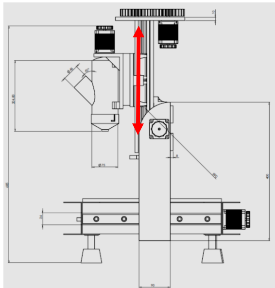
Figura 4-3 Esquema del desplazamiento en Z. Fuente: Elaboración propia
