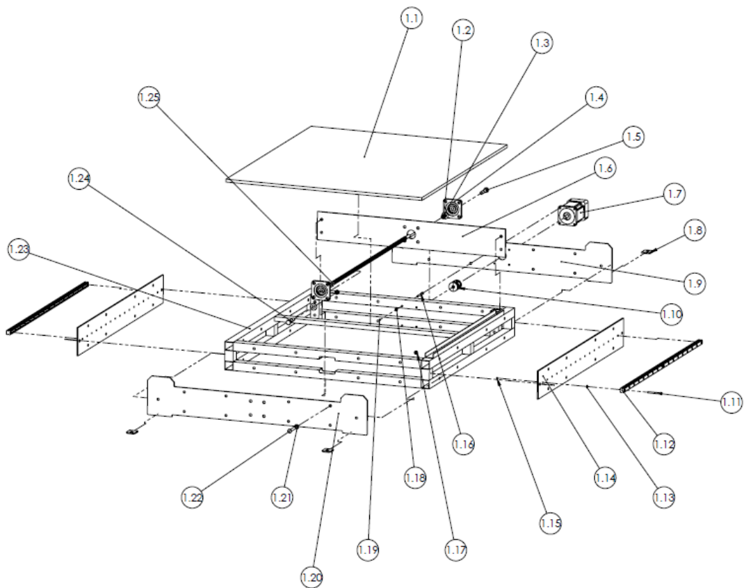
Figura 4-25 Explosionado del subsistema Base. Fuente: Elaboración propia
