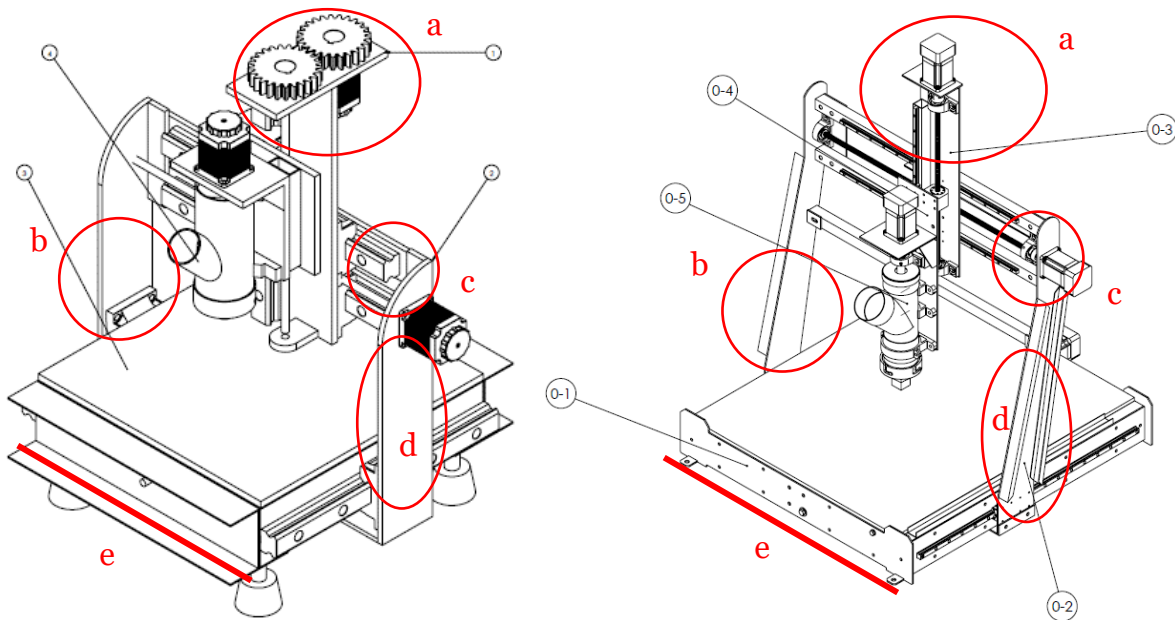
Figura 4-24 Comparación del diseño conceptual, en contraste con el diseño en detalle. Fuente: Elaboración propia.
