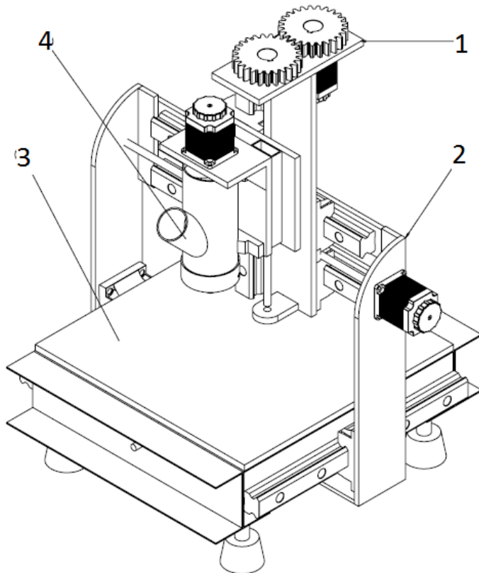
Figura 4-1 Bosquejo conceptual del conjunto. Fuente: Elaboración propia
