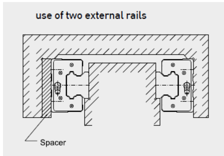
Figura 4-13 Montaje de las guías lineales para el desplazamiento en Y. Fuente: Extracto de catálogo HIWIN
