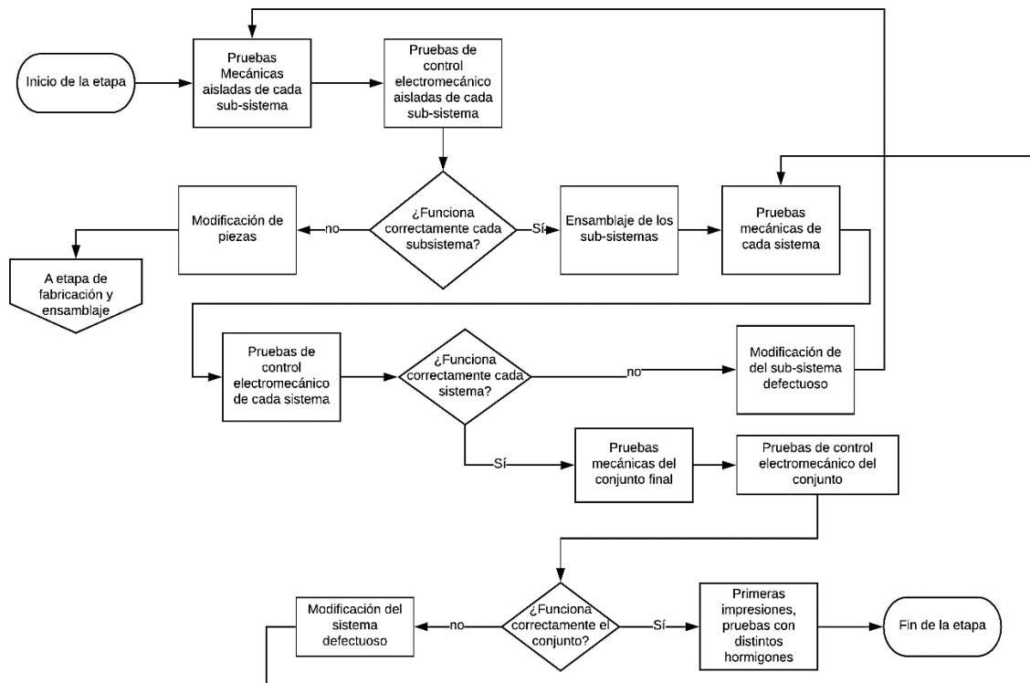
Figura 2-5 Metodología de etapa de pruebas. Fuente: Elaboración propia.
