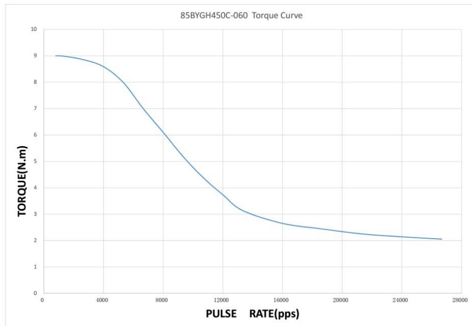
Figura 3-5 Curva de Torque según los pulsos por segundo. Fuente: https://es.aliexpress.com
