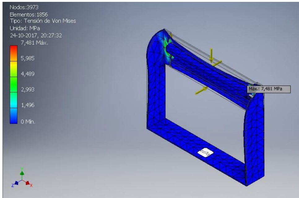
Figura 4-16 Resultados para el estudio de Tensión de Von Mises. Fuente: Elaboración propia
