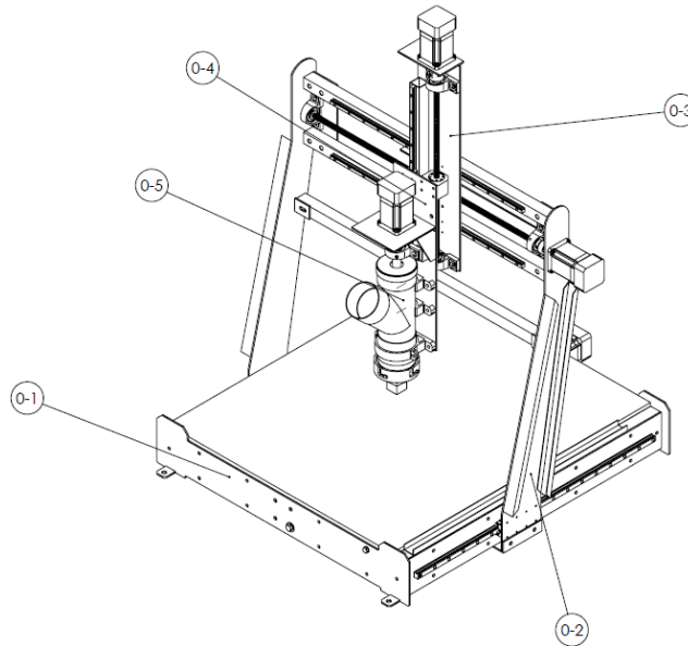
Figura 4-23 Vista isométrica de la impresora 3D extrusora de hormigón. Fuente: Elaboración propia
