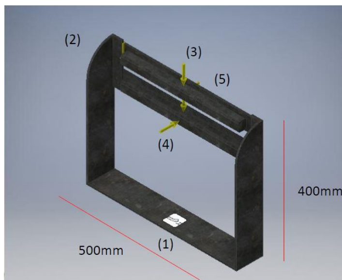
Figura 4-15 Modelación utilizada para el estudio mecánico del subconjunto puente. Fuente: Elaboración Propia
