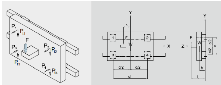
Figura 4-9 Montaje de las guías lineales para el desplazamiento en x e y. Fuente: Extracto de catálogo HIWIN
