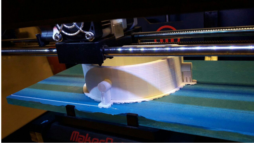
Figura 4-30 Impresión de la pieza "Porta Boquilla" en dependencias del FabLab. Fuente: Elaboración propia
