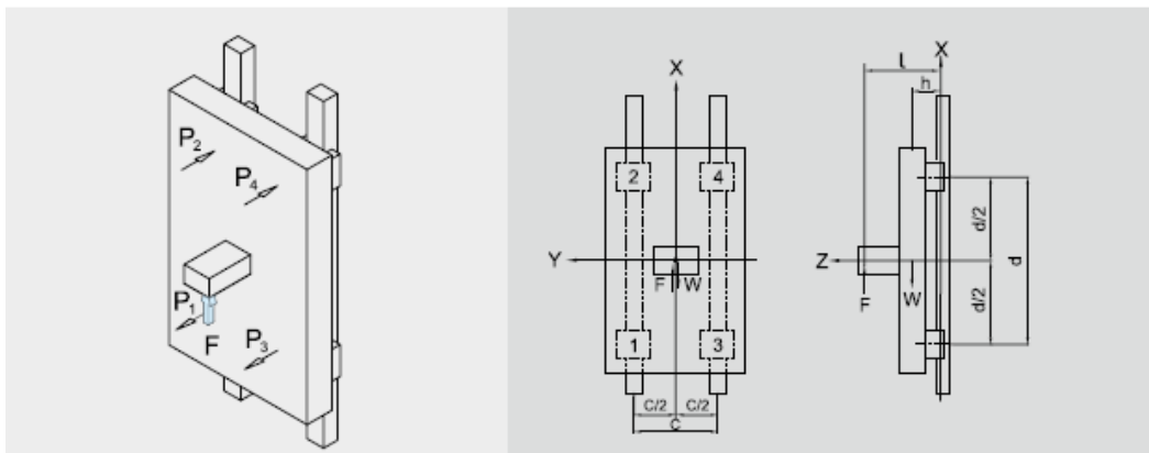
Figura 4-5 Montaje de las guías lineales para el desplazamiento en z. Fuente: Extracto de catálogo HIWIN
