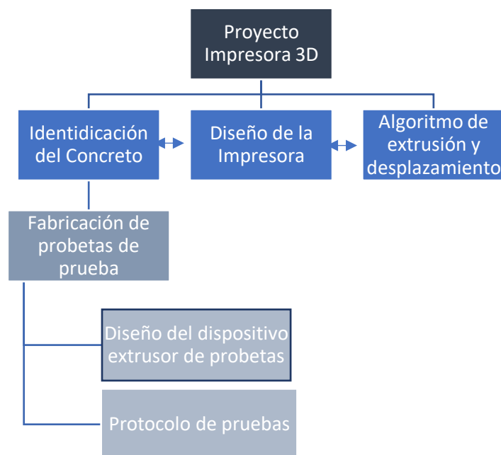
Figura 3-1 Esquema proyecto Impresora 3D de concreto. Fuente: Elaboración propia.
