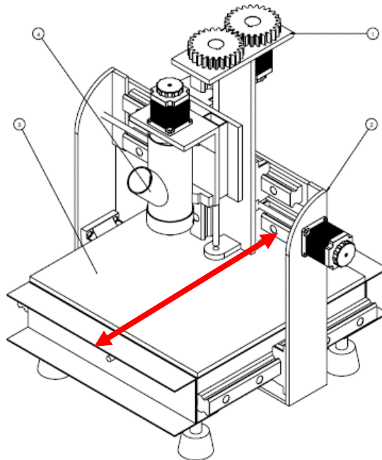
Figura 4-11 Esquema del desplazamiento en Y. Fuente: Elaboración Propia
