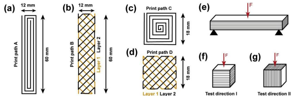
Figura 3-2 a) y b) corresponden a las especificaciones de la impresión de una barra, c) y d) son las especificaciones de impresión de un cubo. e) corresponde a la dirección de la fuerza de ensayo de la barra. f) y g) es la fuerza de ensayo para el cubo. Fuente: (Kazemian, 2017)
