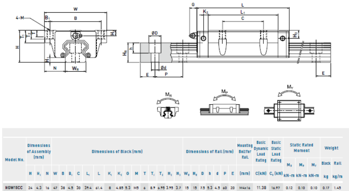
Figura 4-6 Guía Lineal preseleccionada. Fuente: Extracto de catálogo HIWIN
