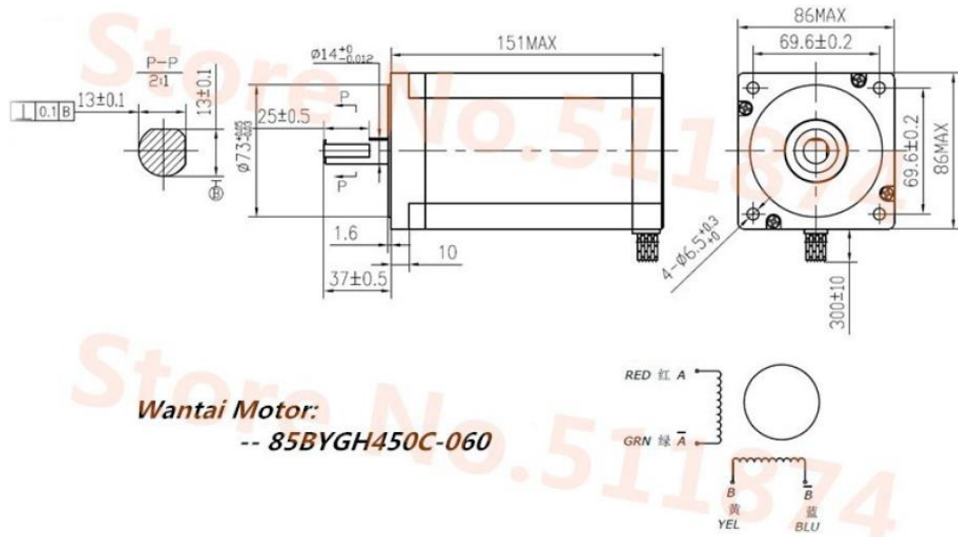
Figura 3-4 Plano del motor con sus principales cotas. Fuente: (Anell, 2015)
