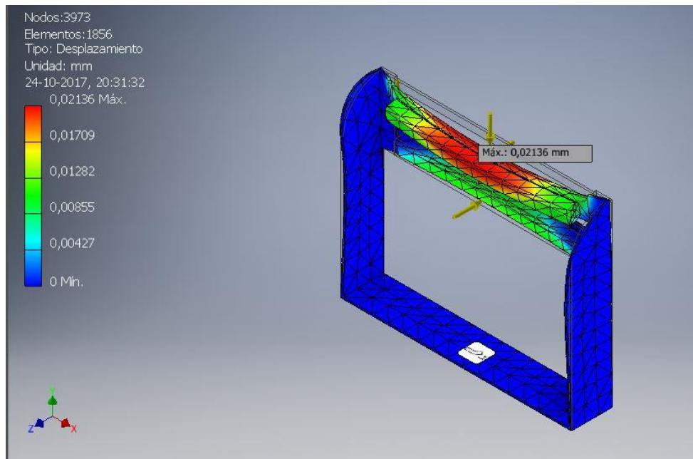
Figura 4-17 Resultados para el estudio de desplazamientos en el subsistema. Fuente: Elaboración Propia
