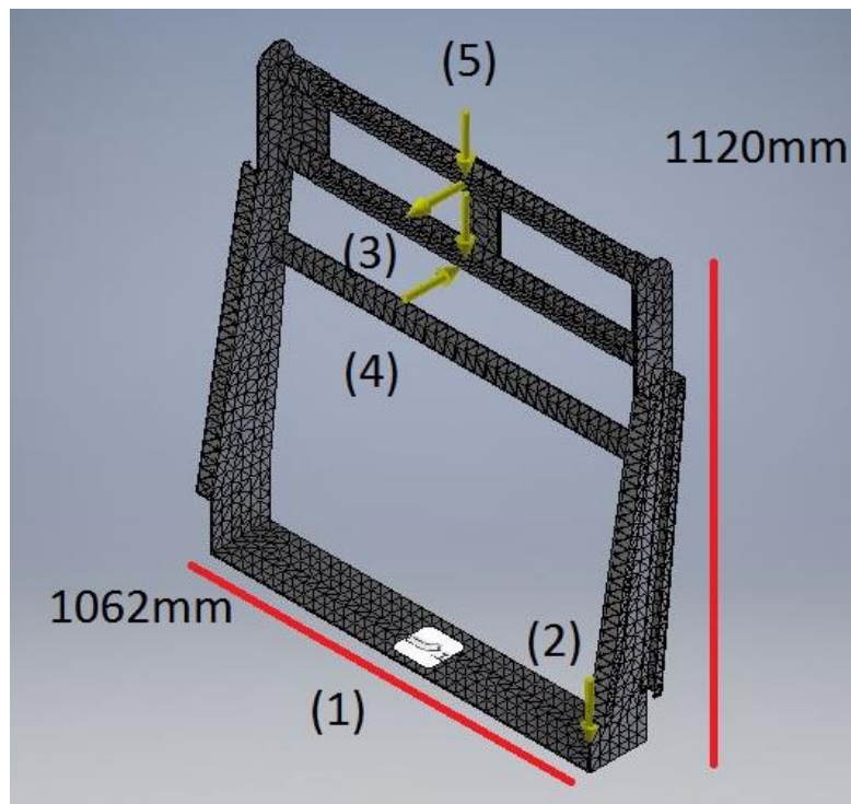
Figura 4-18 Modelación utilizada para el estudio mecánico del subconjunto Puente de la Ingeniería Conceptual. Fuente: Elaboración Propia
