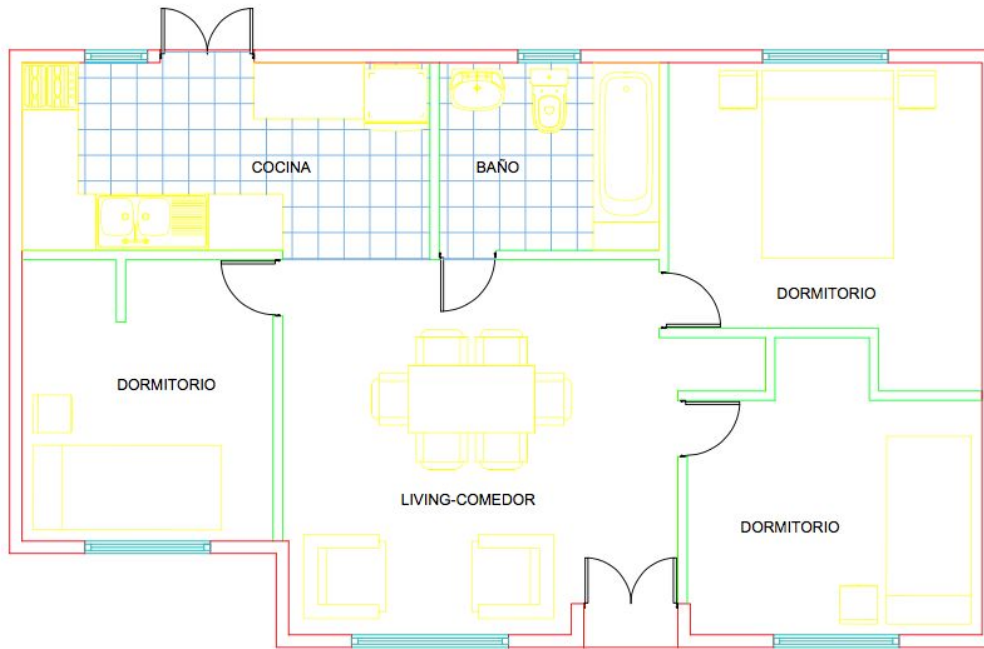
PLANTA DE ARQUITECTURA
