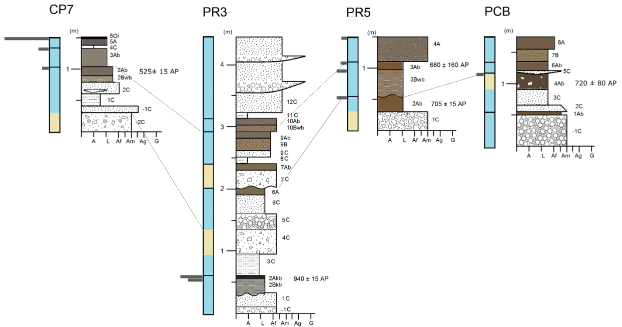
Figura 5.19: Perfiles CP7, PR3, PR5 y PCB. Correlaciones para el período 1000 - 400 AP.
