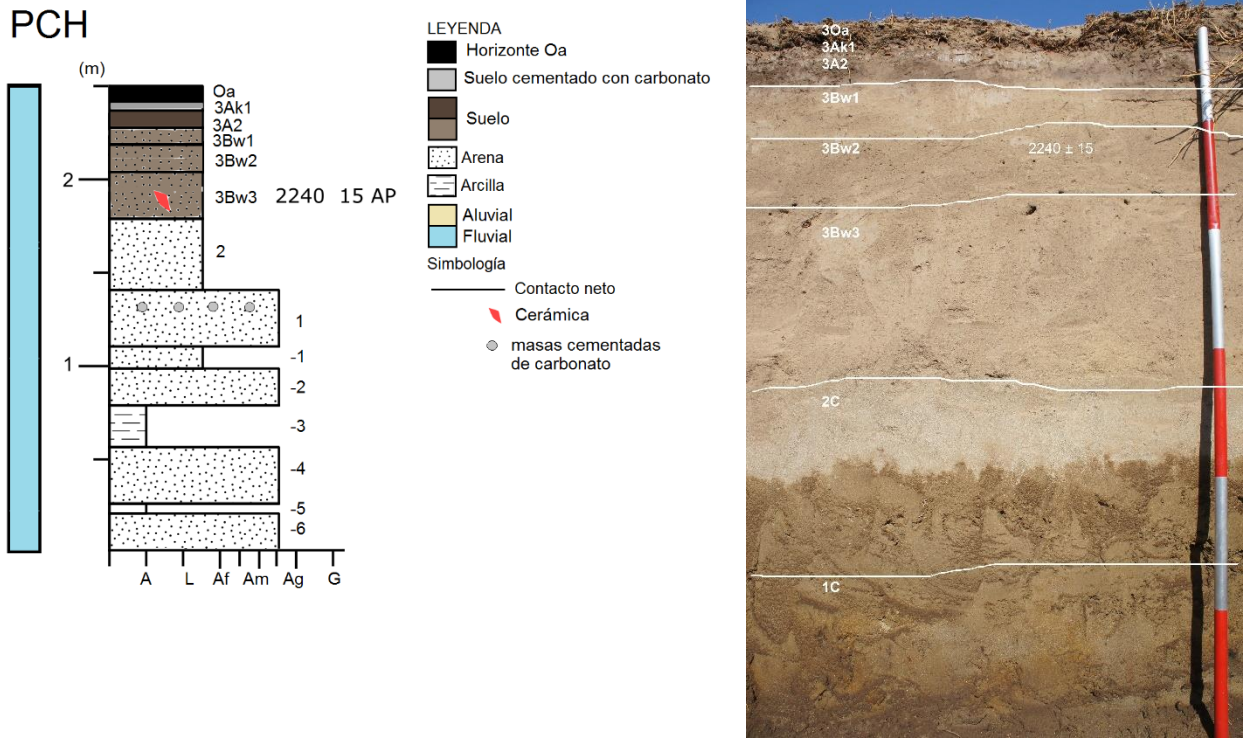
Figura 5.7: columna y foto del perfil PCH.
