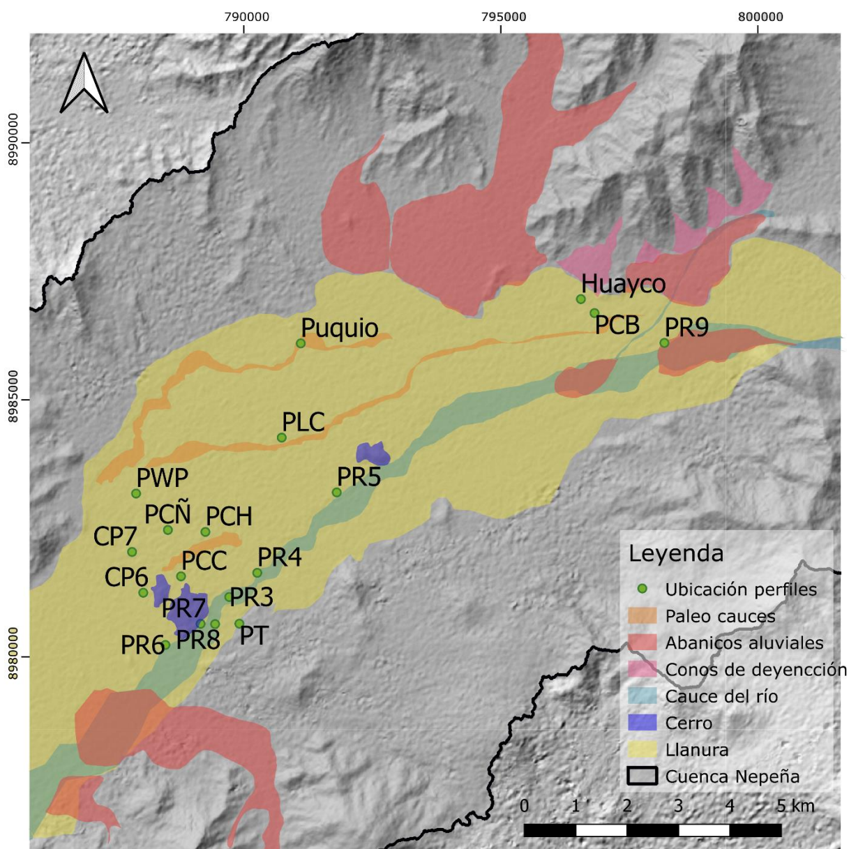
Figura 5.2: Mapa geomorfológico de la zona de estudio escala 1:90000. Los círculos verdes muestran la ubicación de los perfiles descritos en terreno. Elaboración propia.
