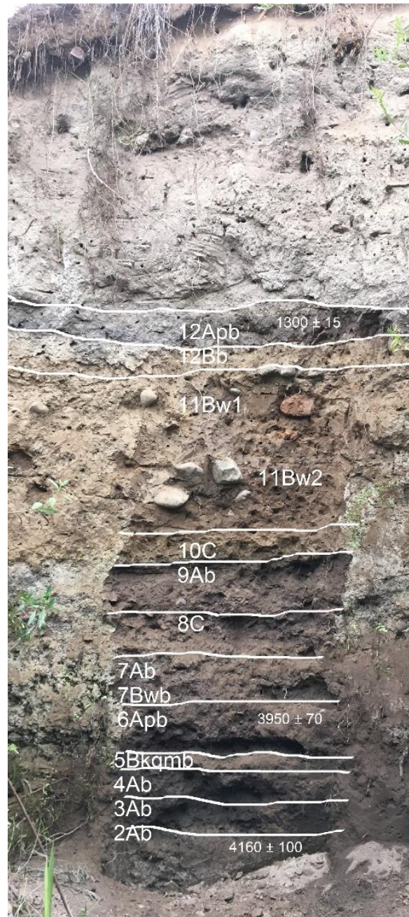
Figura 5.4: Foto del perfil PR7
