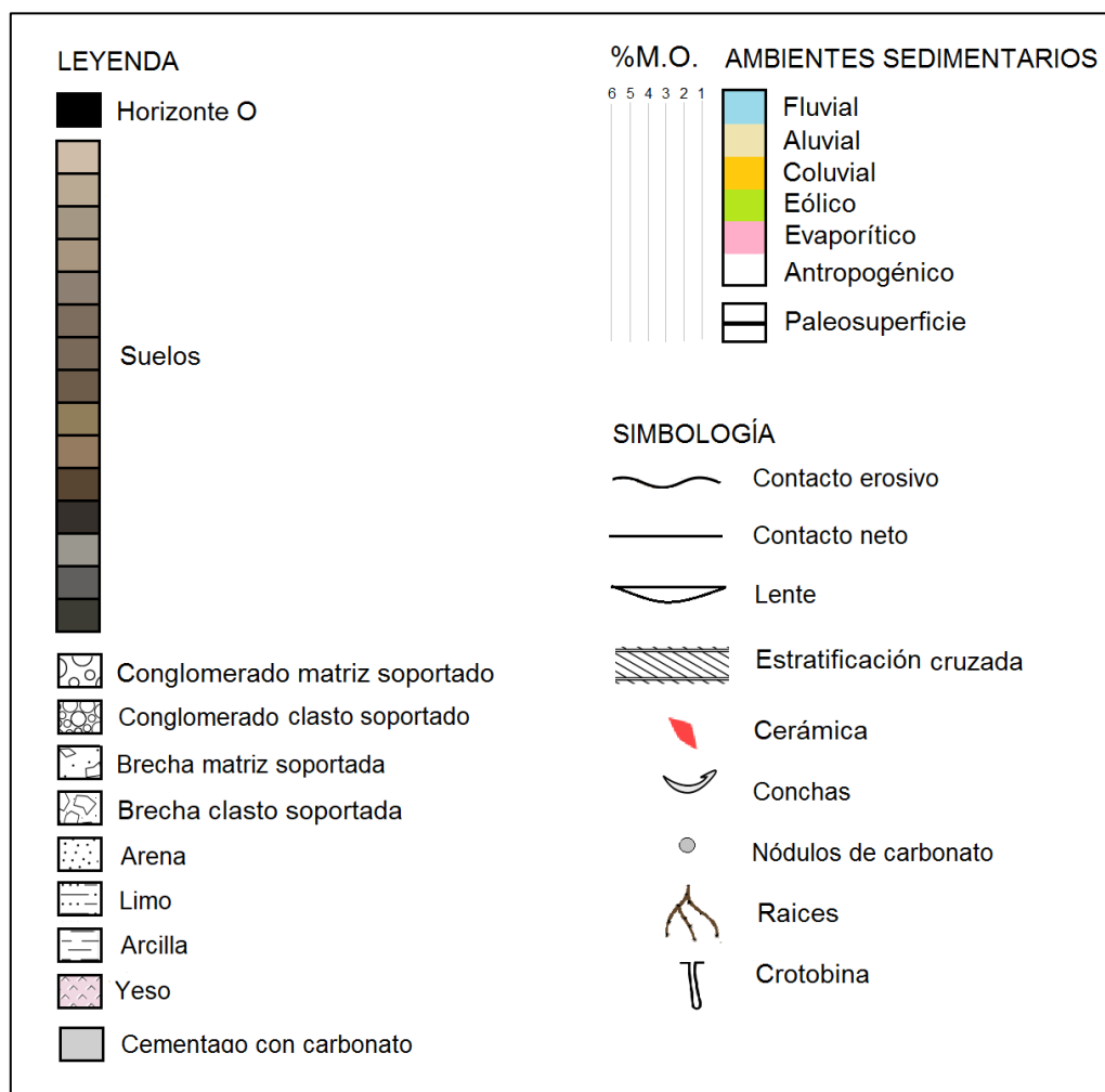
Figura 5.17: Leyenda y simbología para las figuras 5.18 a 5.22.
