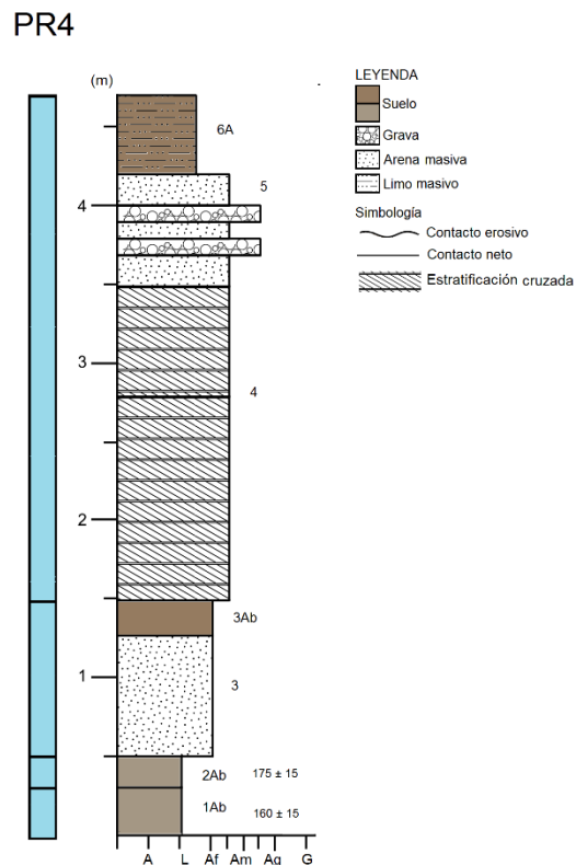
Figura 8.3: Foto y columna del perfil PR4.
