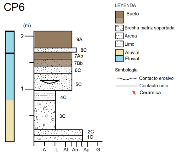
Figura 8.17: Foto y perfil CP6.
