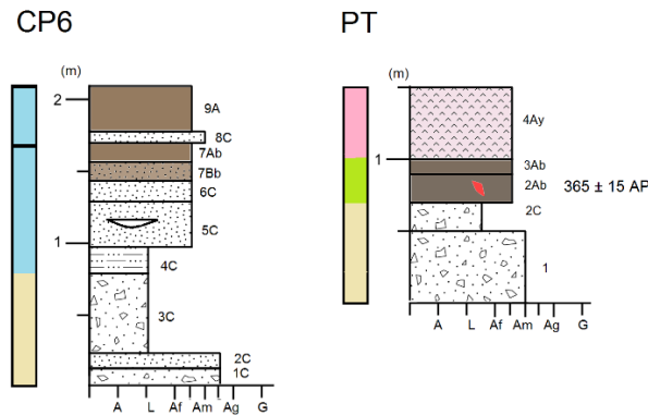
Figura 5.20: Perfiles CP6 y PT.
