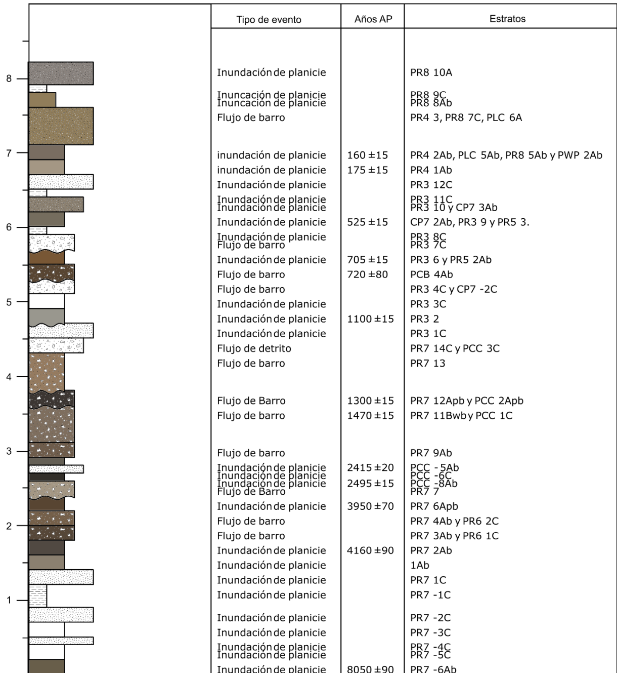
Figura 5.23: Columna que sintetiza las inundaciones y flujos de barro encontradas en terreno. Los estratos que aparecen en color indican que tuvieron formación de suelo.
