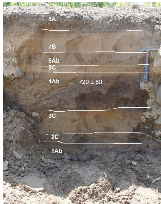
Figura 8.15: Columna y foto del perfil PCB.
