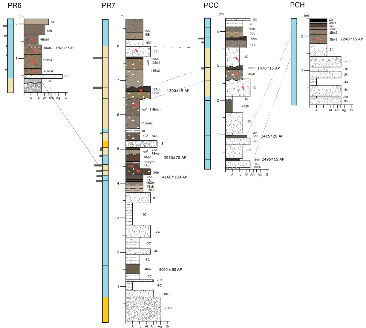
Figura 5.18: Perfiles PR6, PR7, PCC y PCH. Correlaciones para los períodos 10000 – 3500 AP y 3500 - 1000 AP.
