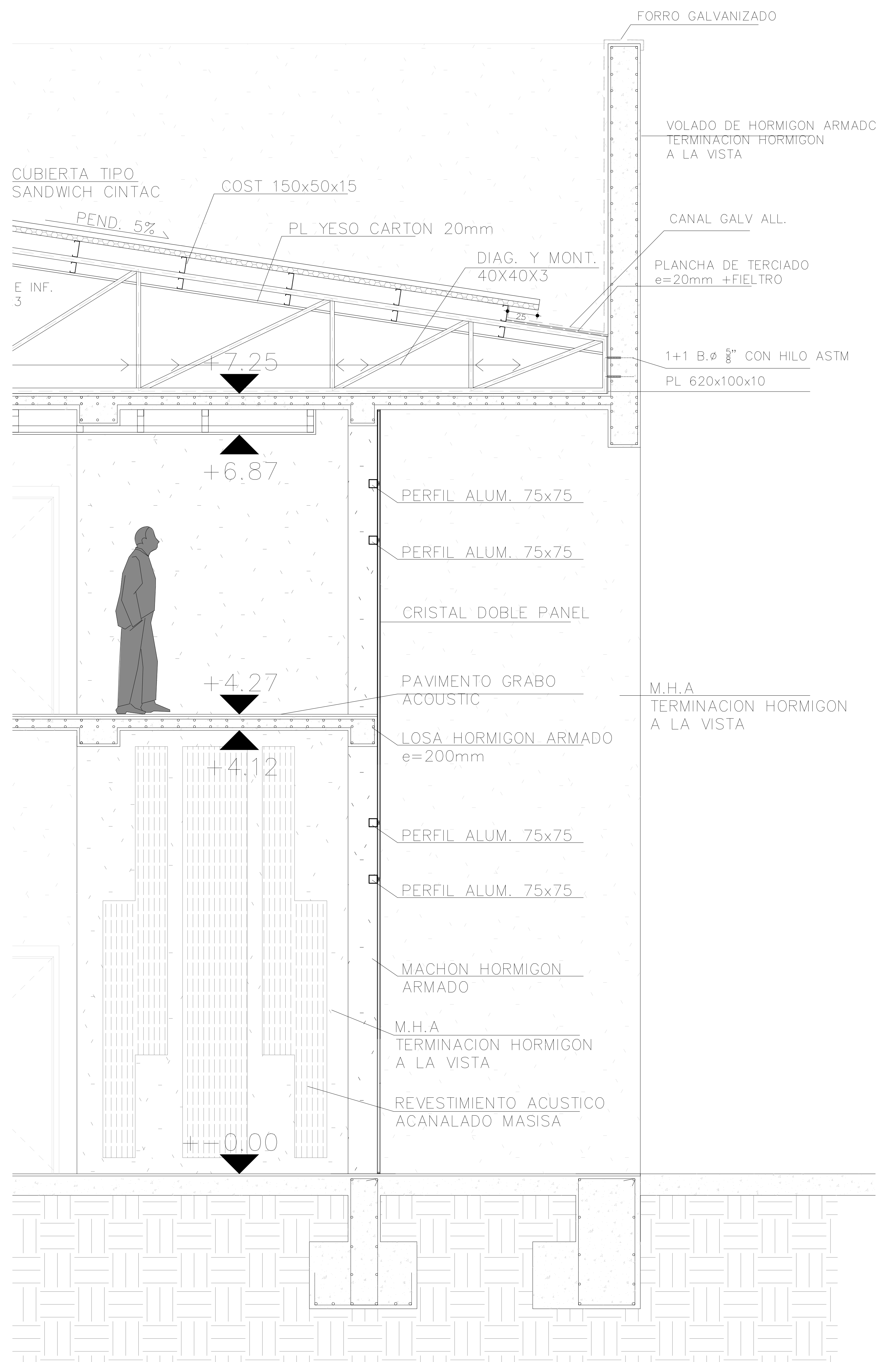
ESCANTILLON 2 CORTE B-B ELEVACION EJE I AUDITORIO ESCALA: 1/200
