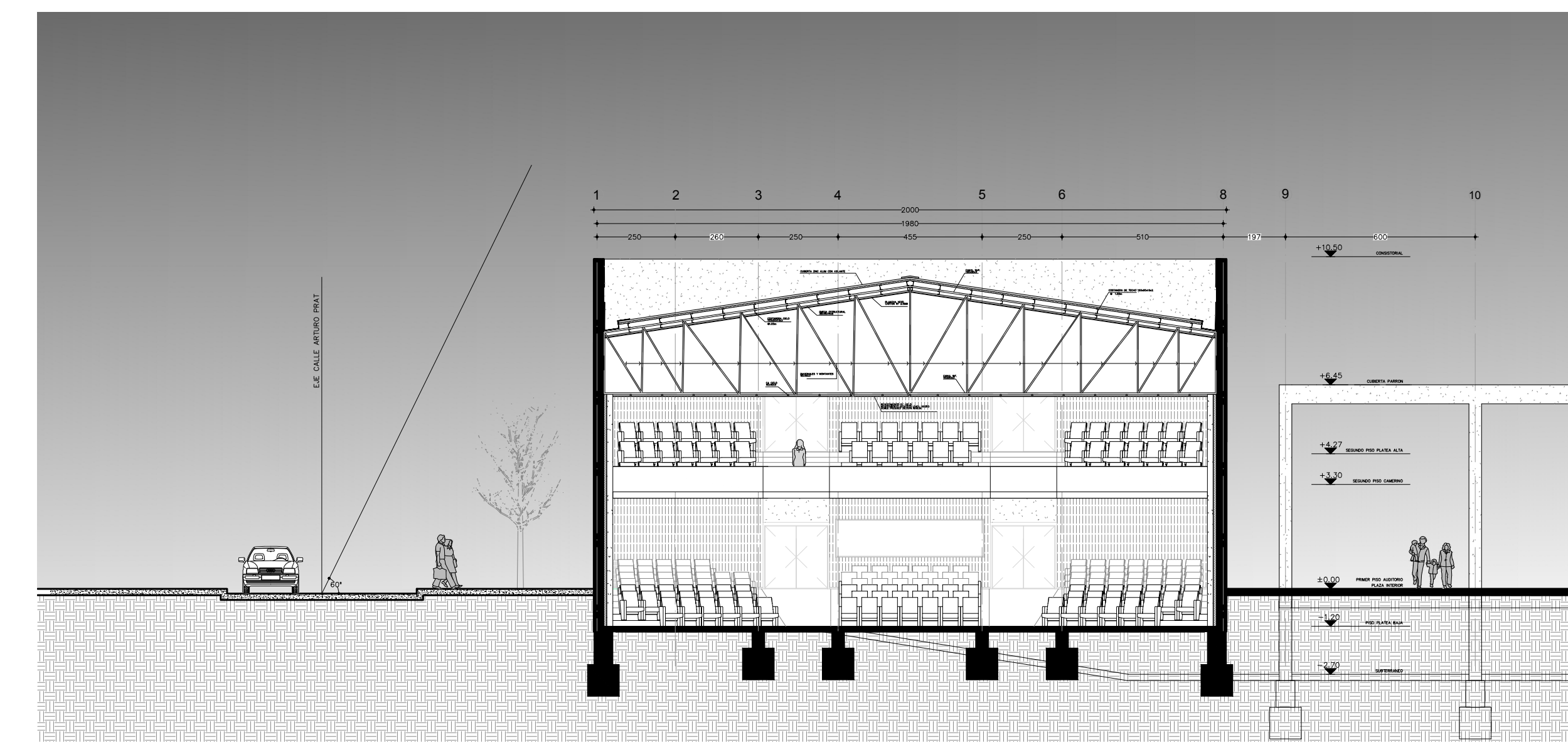
CORTE D-D ESCALA: 1/1500
