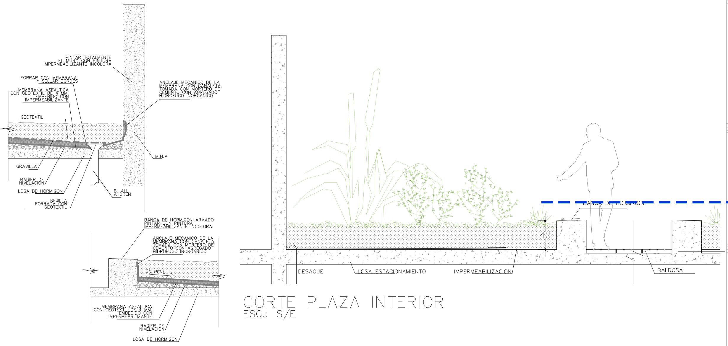
DETALLE IMPERMEABILIZACION ESC.: S/E
