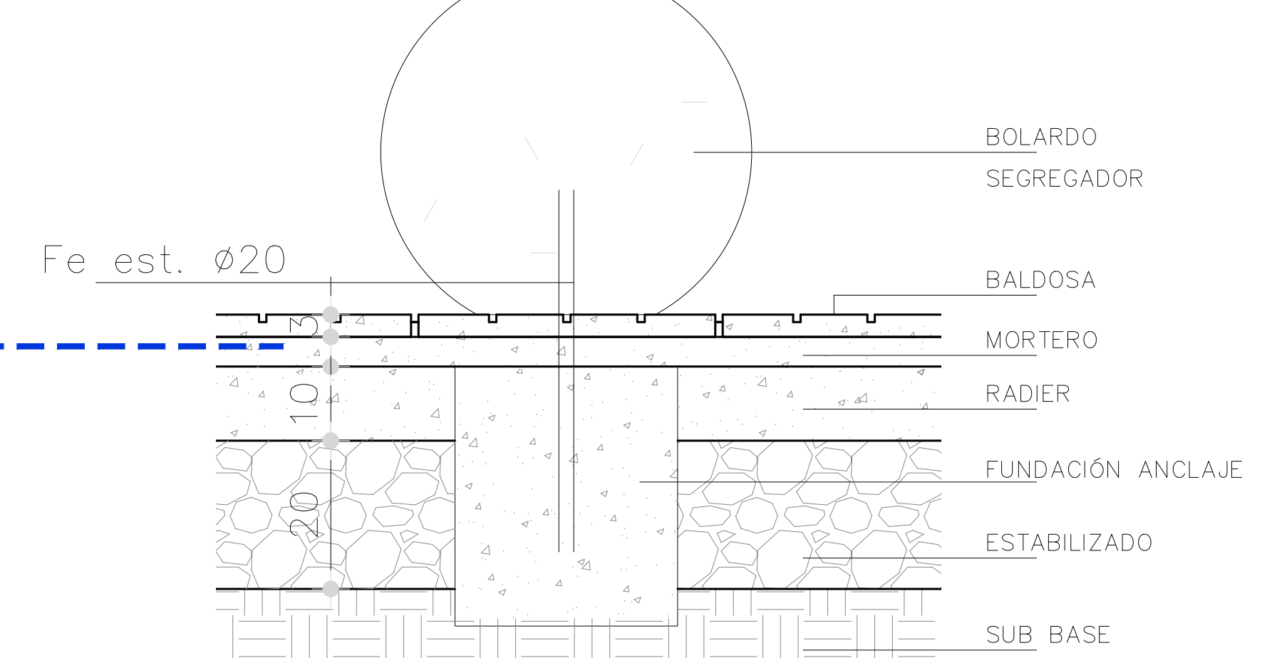
SEGREGADOR ESFERICO / BOLARDO
