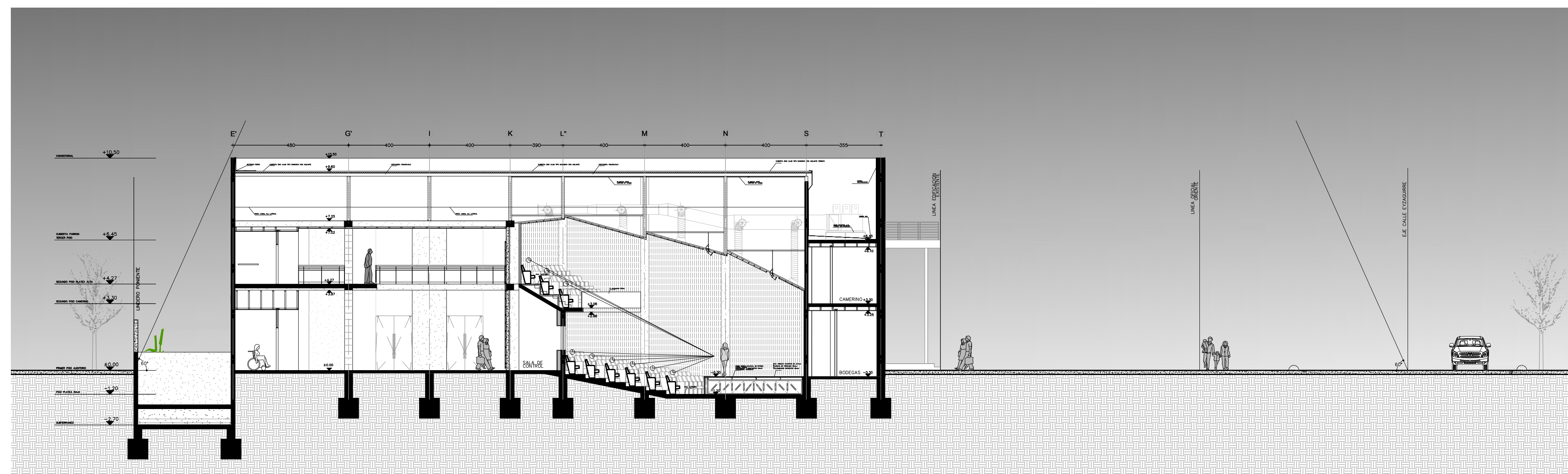
CORTE C-C ESCALA: 1/1500
