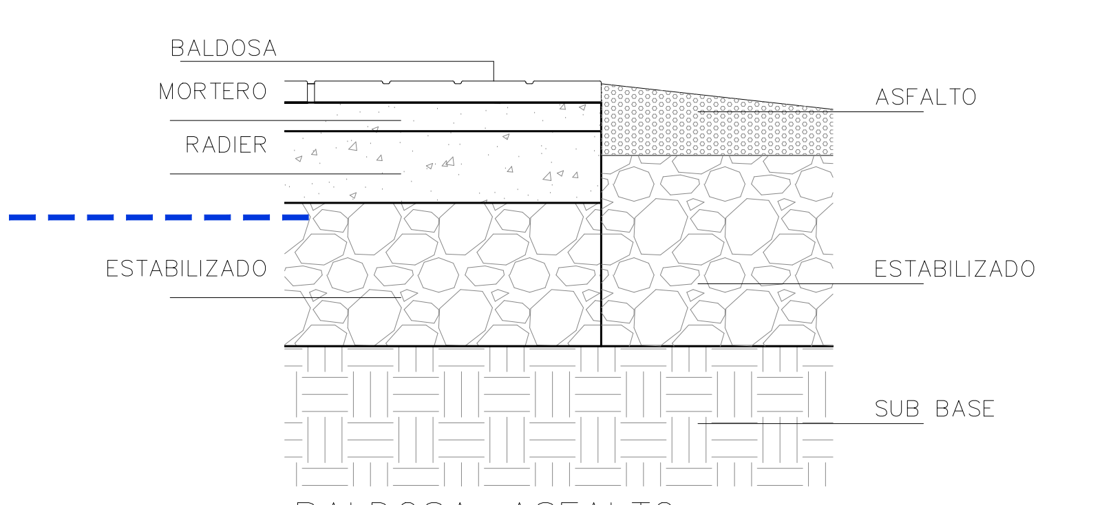
BALDOSA - ASFALTO
