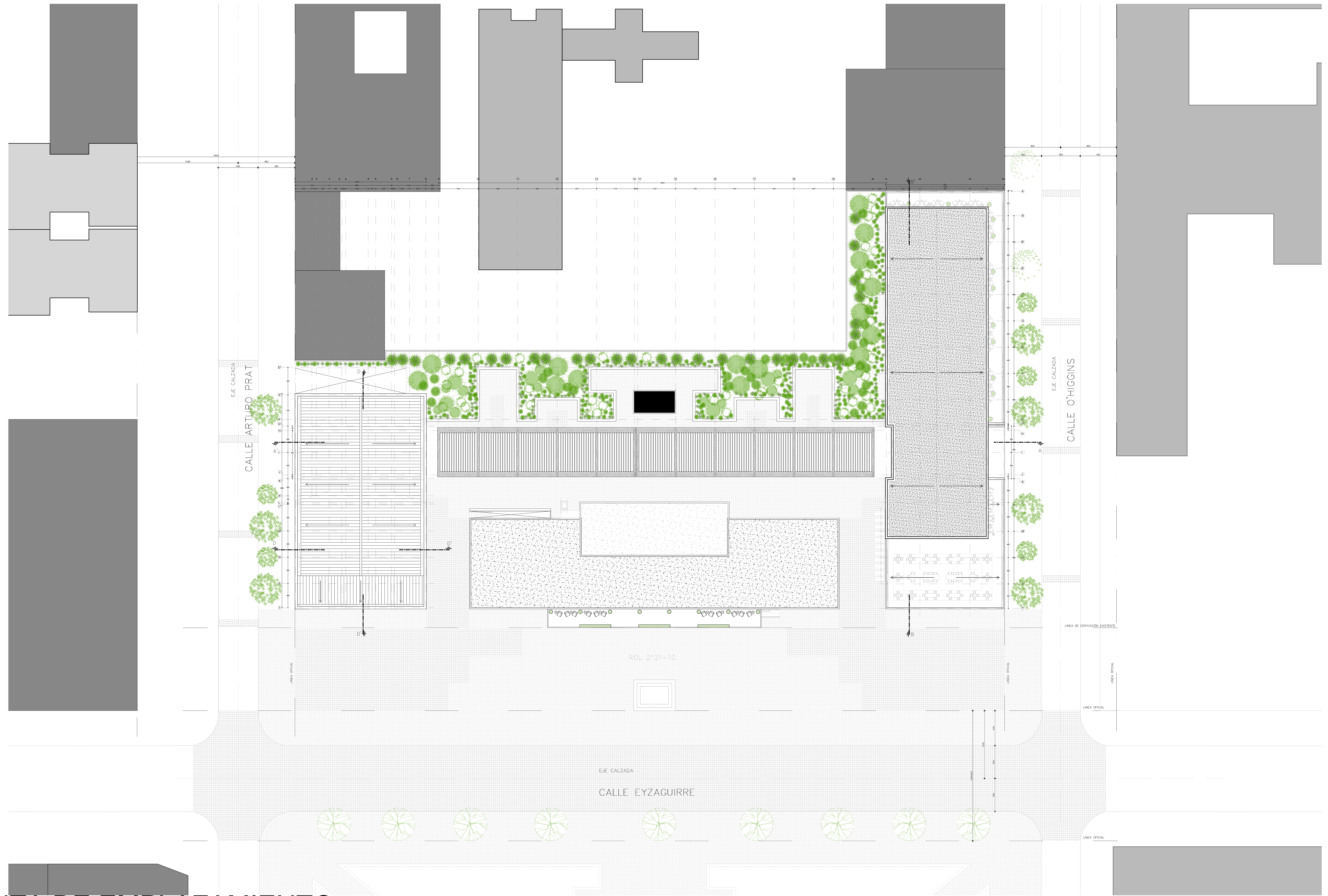
PLANTA DE EMPLAZAMIENTO ESCALA: 1/2000
