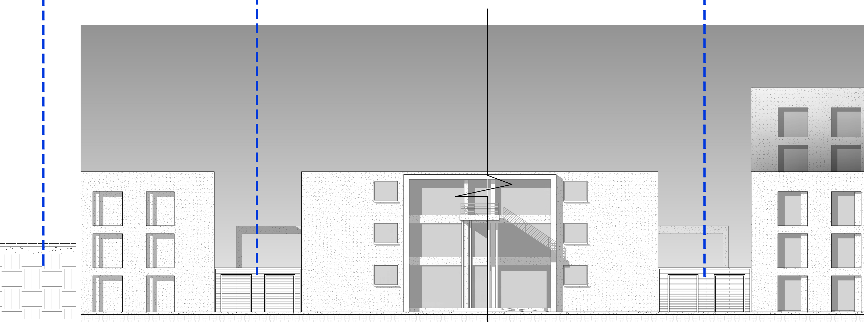
REJA PROPUESTA FACHADA ORIENTE ESC.: S/E
