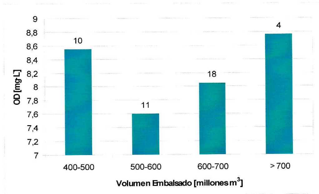
Figura 13. Promedio de OD por rango de volumen. Para la elaboración de éste gráfico se tomaron los datos de OD y volumen embalsado coincidentes en fechas entre 1993 y 2008, se separaron en los rangos respectivos y se calculó un promedio para cada uno. El número sobre las barras indica la cantidad de datos promediados
