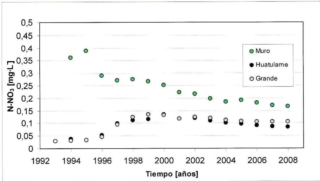
Figura 24. Comparación de la evolución de la concentración de nitrato (N-NO 3 ) entre las estaciones de monitoreo. Para la elaboración de los gráficos se realizó un promedio acumulado sobre los datos brutos y con los datos resultantes se calculó un promedio anual.
