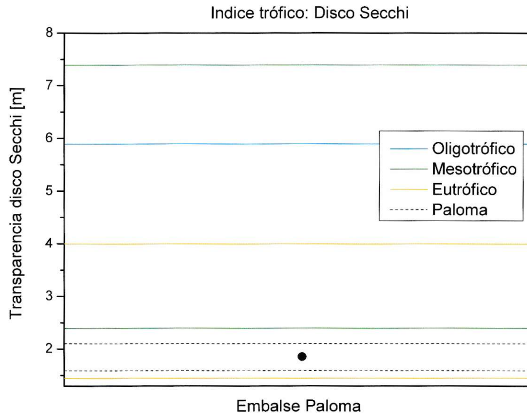
Figura 1. Estado trófico para el embalse La Paloma basado en la transparencia del disco Secchi. El ● indica la media geométrica (G) y las líneas discontinuas indican el rango G \pm ds de la transparencia.
