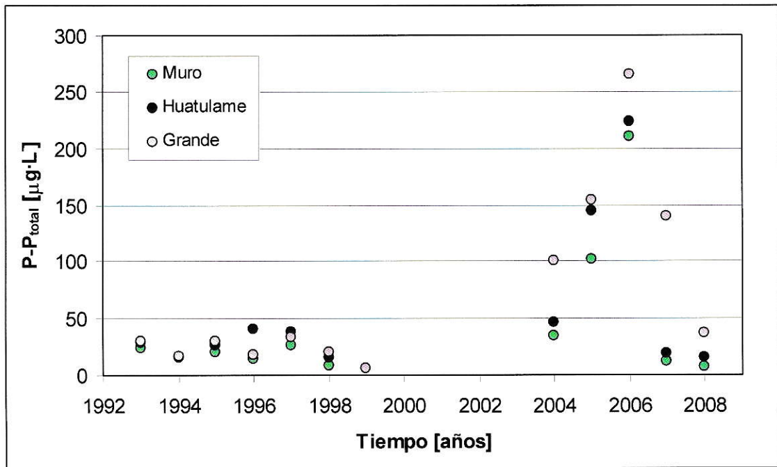
Figura 28. Comparación de la evolución de la concentración de P-P total entre las estaciones de monitoreo. Para la elaboración de los gráficos se realizó un promedio acumulado sobre los datos brutos y con los datos resultantes se calculó un promedio anual.
