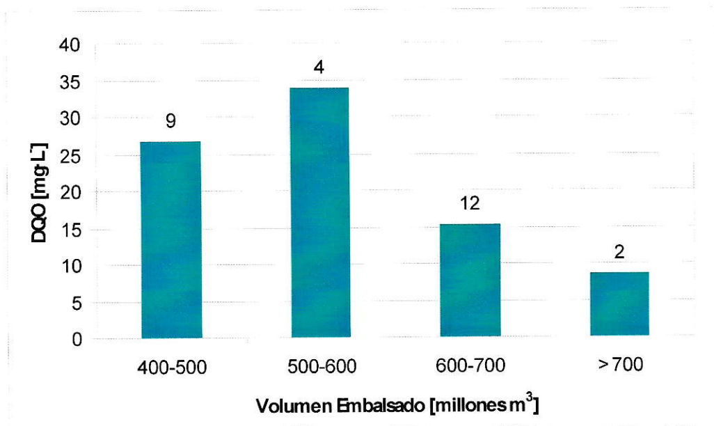
Figura 12. Promedio de DQO por rango de volumen. Para la elaboración de éste gráfico se tomaron los datos de DQO y volumen embalsado coincidentes en fechas entre 1993 y
