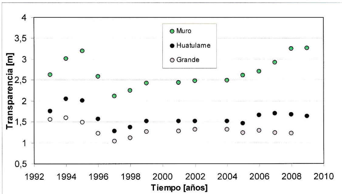
Figura 30. Comparación de la evolución de la transparencia del DS entre las estaciones de monitoreo. Para la elaboración de los gráficos se realizó un promedio acumulado sobre los datos brutos y con los datos resultantes se calculó un promedio anual.
