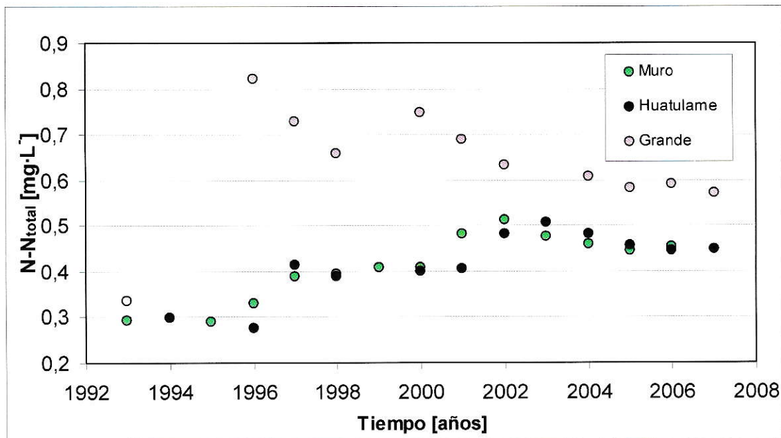
Figura 26. Comparación de la evolución de la concentración del N-N Total entre las estaciones de monitoreo. Para la elaboración de los gráficos se realizó un promedio acumulado sobre los datos brutos y con los datos resultantes se calculó un promedio anual.
