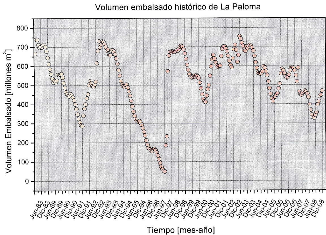
Figura 6. Datos de volumen embalsado mensual de La Paloma (1988-2008). Fuente:
