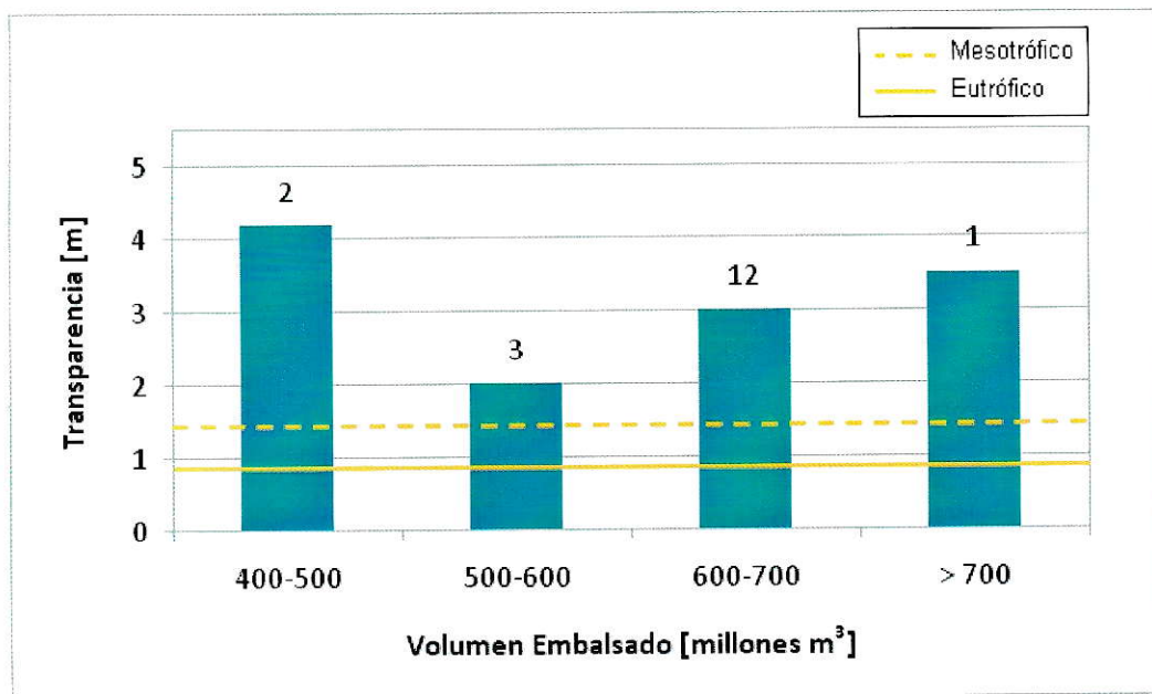
Figura 15. Promedio de transparencia del disco Secchi por rango de volumen. Para la elaboración de éste gráfico se tomaron los datos de transparencia y volumen embalsado coincidentes en fechas entre 1993 y 2008, se separaron en los rangos respectivos y se calculó un promedio para cada uno. El número sobre las barras indica la cantidad de datos promediados.
