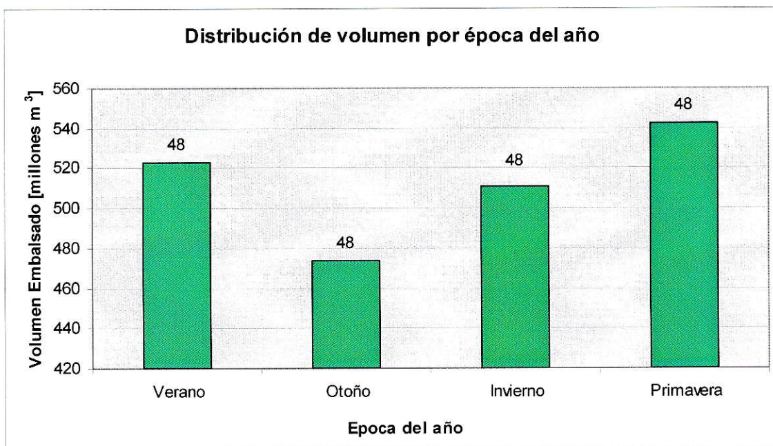
Figura 8. Distribución de volumen embalsado por época del año en el embalse La Paloma. Para la elaboración de este gráfico se tomaron datos de volumen embalsado entre 1993 y 2008, se separaron por época del año y se calculó un promedio para cada época. El número sobre las barras indica la cantidad de datos promediados.
