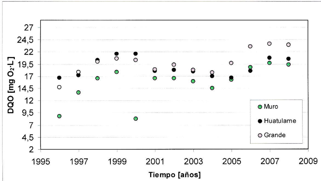
Figura 29. Comparación de la evolución de la demanda química de oxígeno (DQO) entre las estaciones de monitoreo. Para la elaboración de los gráficos se realizó un promedio acumulado sobre los datos brutos y con los datos resultantes se calculó un promedio anual.
