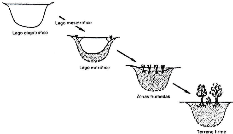
Figura 1. Eutroficación. Proceso de envejecimiento en la evolución ecológica (Settler, Ramalho y Beltran, 1996).
