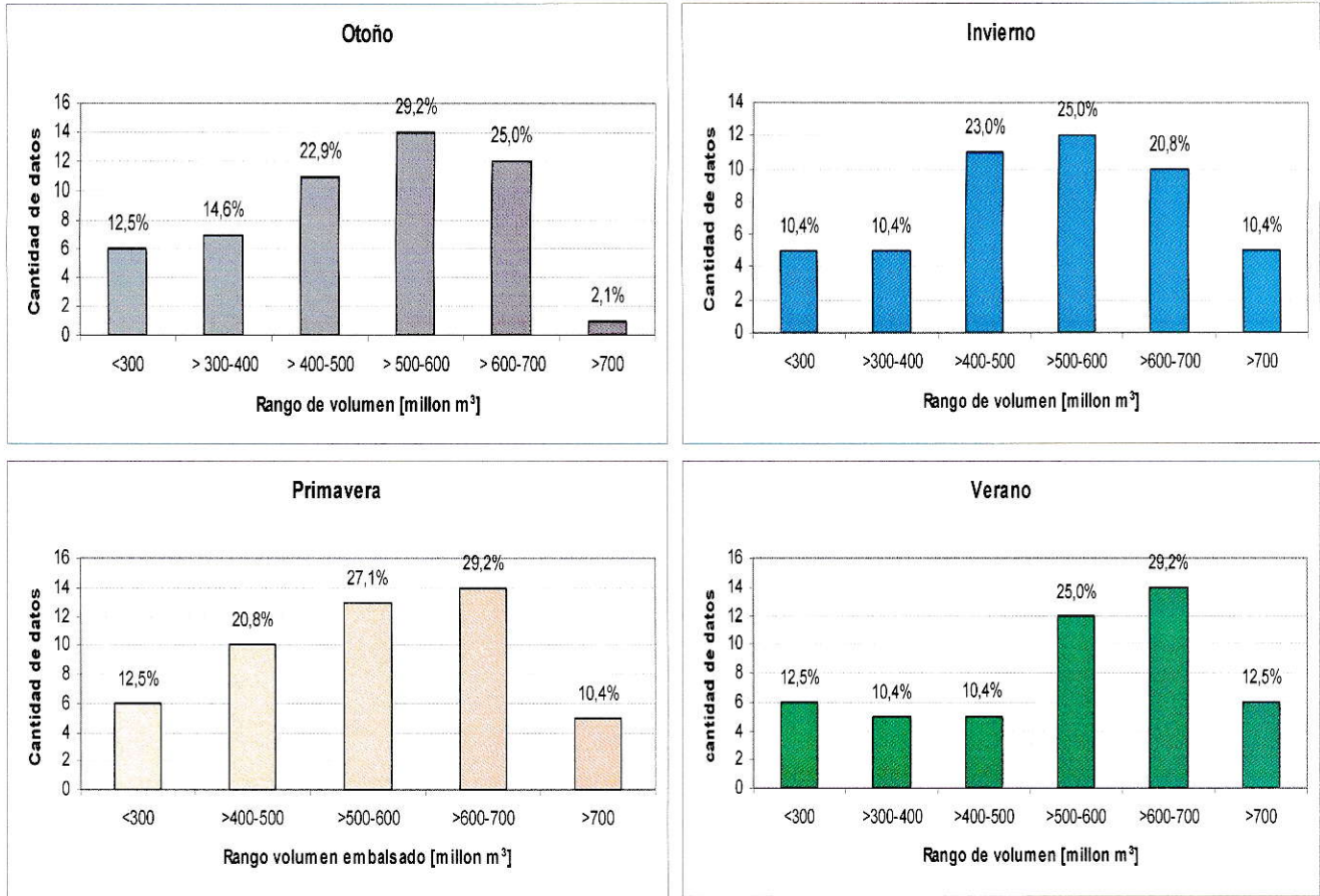
Figura 9. Porcentaje de datos de volumen embalsado por rango en cada época del año para el embalse La Paloma. Entre 1993 y 2008 cada época del año registro 48 datos. Se separaron éstos en los distintos rangos de volumen y se calculó el porcentaje de datos de cada rango.
