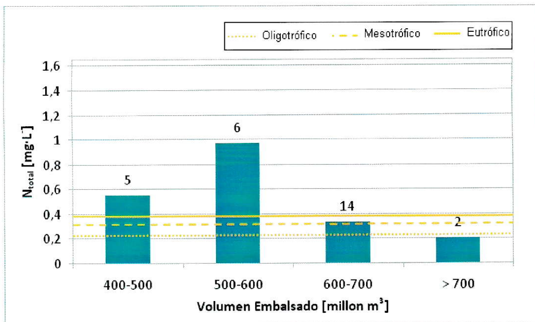
Figura 16. Promedio de la concentración de N-N total por rango de volumen. Para la elaboración de éste gráfico se tomaron los datos de N-N total y volumen embalsado coincidentes en fechas entre 1993 y 2008, se separaron en los rangos respectivos y se calculó un promedio para cada uno. El número sobre las barras indica la cantidad de datos promediados.
