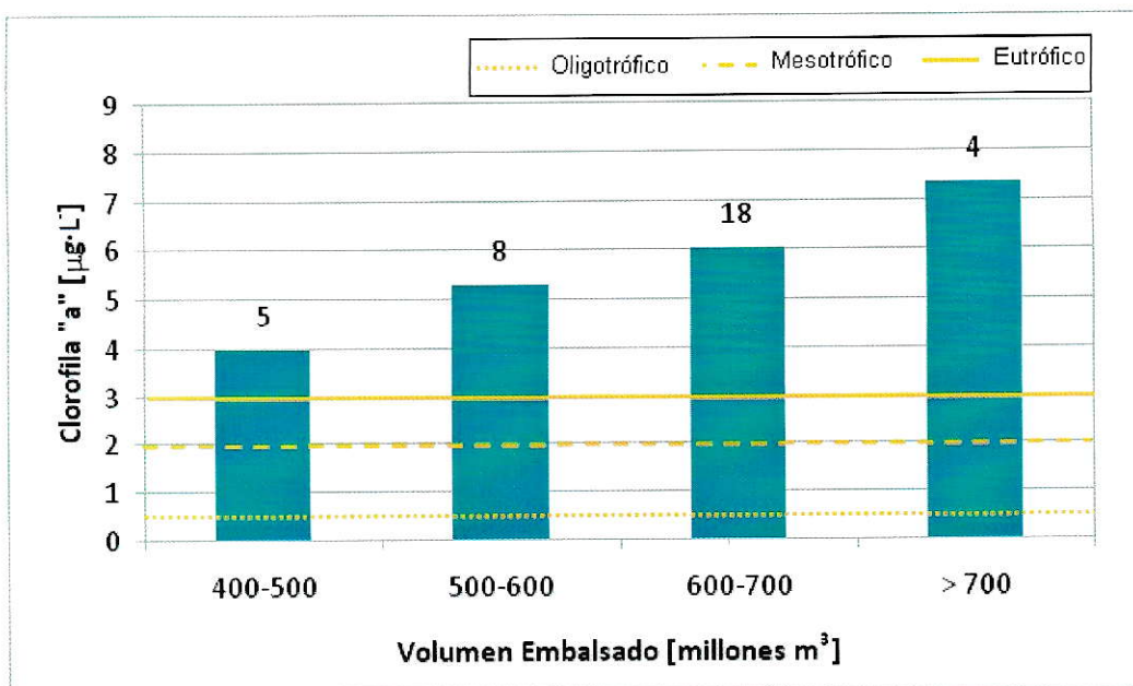
Figura 19. Promedio de la concentración de Cl “a” por rango de volumen. Para la elaboración de éste gráfico se tomaron los datos de Cl “a” y volumen embalsado coincidentes en fechas entre 1993 y 2008, se separaron en los rangos respectivos y se calculó un promedio para cada uno. El número sobre las barras indica la cantidad de datos promediados.
