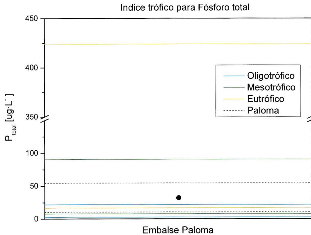
Figura 3. Estado trófico para el embalse La Paloma basado en la concentración de fósforo total. El ● indica la media geométrica (G) y las líneas discontinuas indican el rango G \pm 2ds del P_{total}
