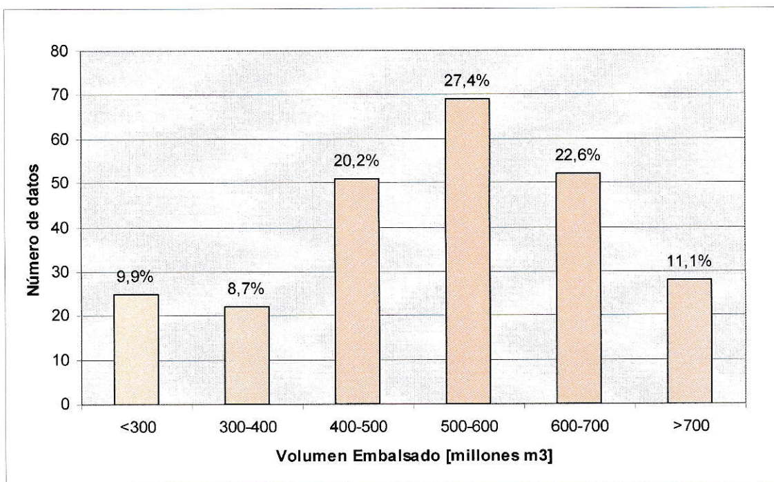
Figura 7. Distribución de rangos de volumen embalsado en el embalse La Paloma. Para la elaboración de éste gráfico se tomaron aquellos datos entre 1993 y 2008, se separaron en los respectivos rangos y se calculó el porcentaje de cada rango en el universo de datos totales.
