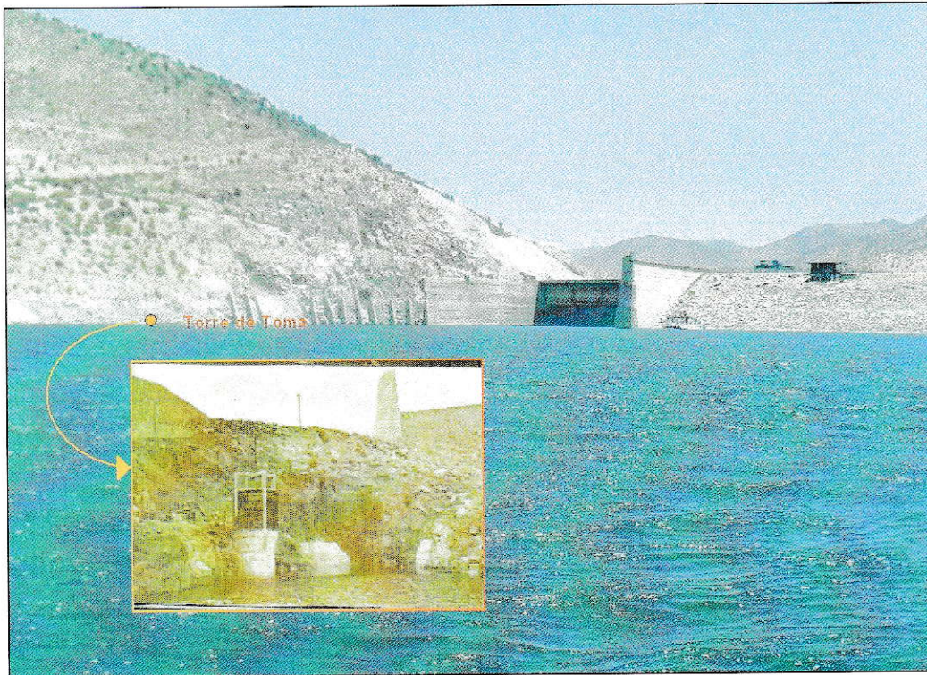
Figura 9. Torre de toma del embalse La Paloma.
