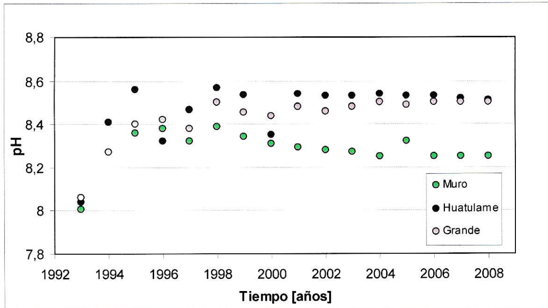
Figura 21. Comparación de la evolución del pH entre las estaciones de monitoreo. Para la elaboración de los gráficos se realizó un promedio acumulado sobre los datos brutos y con los datos resultantes se calculó un promedio anual.
