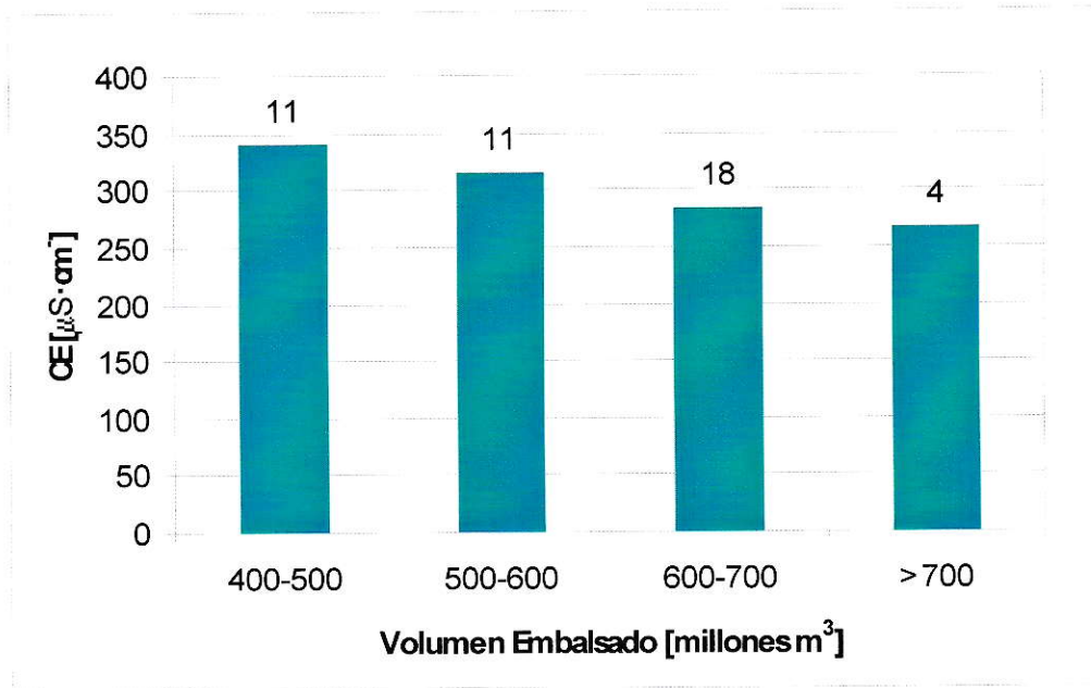
Figura 11. Promedio de CE por rango de volumen. Para la confección de éste gráfico se tomaron los datos de CE y volumen embalsado coincidentes en fechas entre 1993 y 2008, se separaron en los rangos respectivos y se calculó un promedio para cada uno. El número sobre las barras indica la cantidad de datos promediados.
