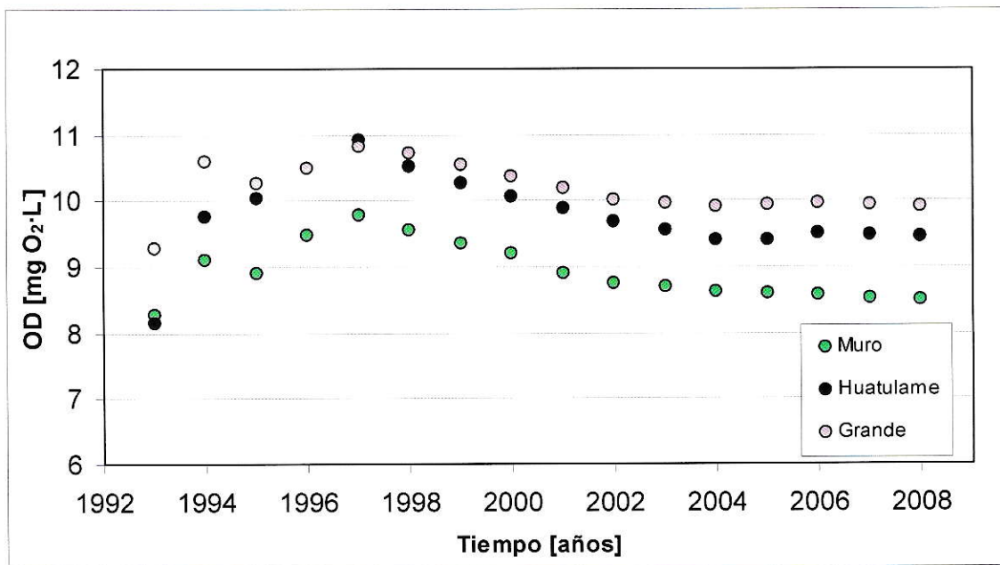
Figura 23. Comparación de la evolución del OD entre las estaciones de monitoreo. Para la elaboración de los gráficos se realizó un promedio acumulado sobre los datos brutos y con los datos resultantes se calculó un promedio anual.
