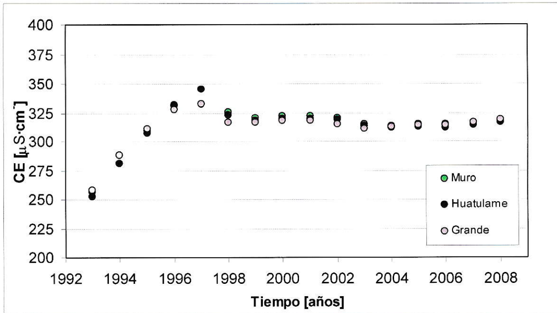
Figura 22. Comparación de la evolución de la CE entre las estaciones de monitoreo.
