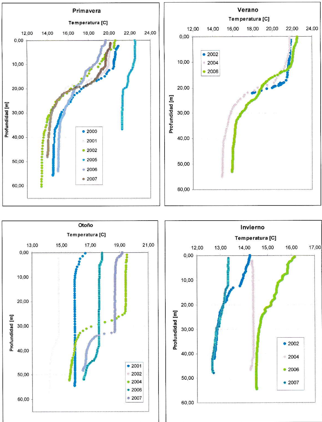
Figura 20. Perfiles de temperatura para la estación Muro desde el año 2000 al 2007.
