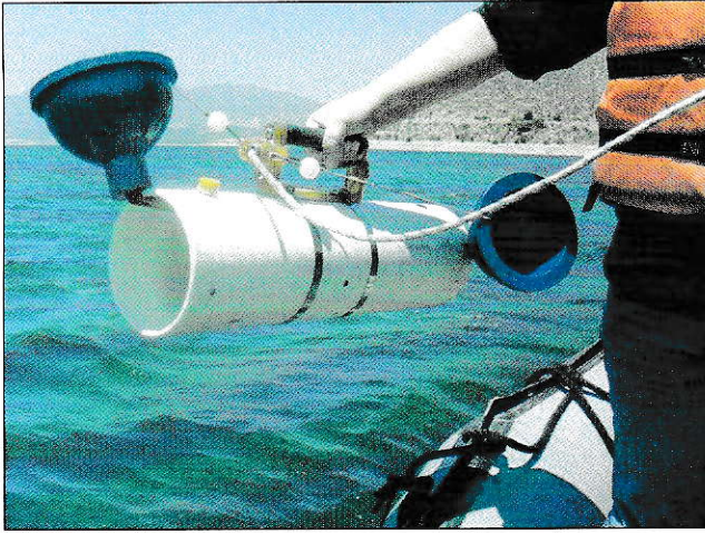
Figura 15. Botella Van Dorn para extraer para muestras a profundidad.
