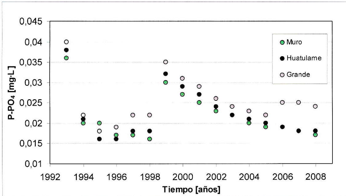
Figura 27. Comparación de la evolución de la concentración del P-PO 4 entre las estaciones de monitoreo. Para la elaboración de los gráficos se realizó un promedio acumulado sobre los datos brutos y con los datos resultantes se calculó un promedio anual.
