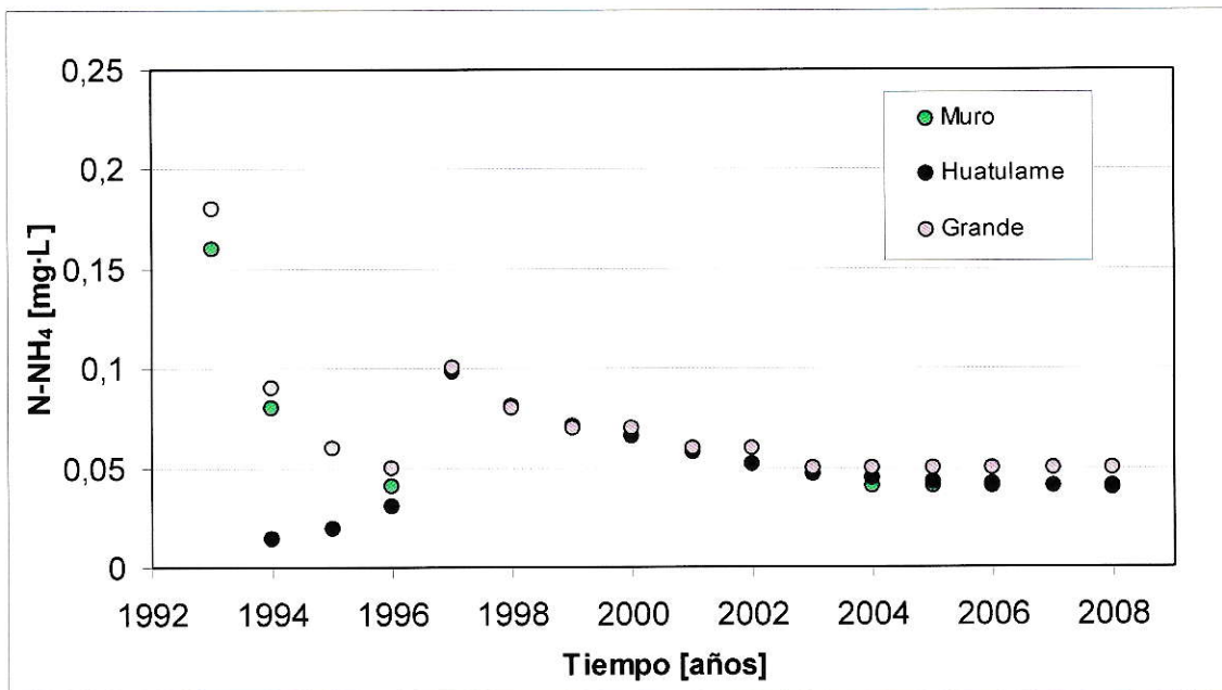
Figura 25. Comparación de la evolución de la concentración de amonio (N-NH 4 ) entre las estaciones de monitoreo. Para la elaboración de los gráficos se realizó un promedio acumulado sobre los datos brutos y con los datos resultantes se calculó un promedio anual.
