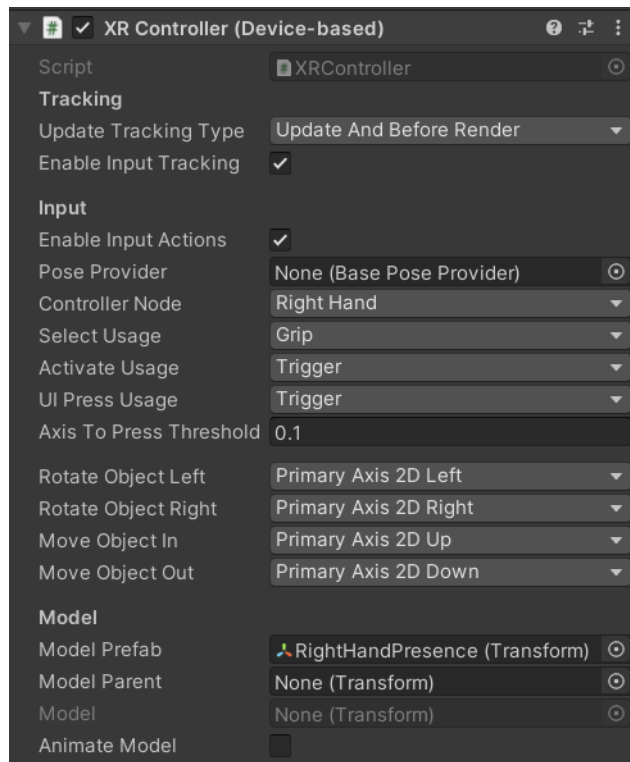
Figura 4.3: Componente XR Controller
