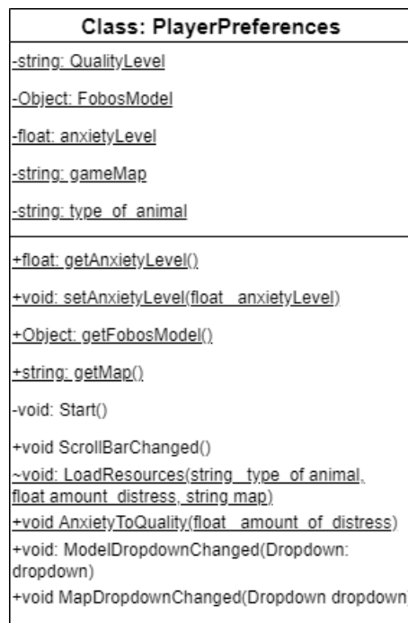
Figura 4.12: Diagrama de PlayerPreferences
