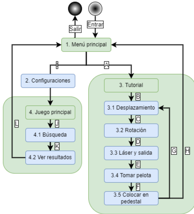
Figura 3.1: Representación gráfica de la máquina de estados.
