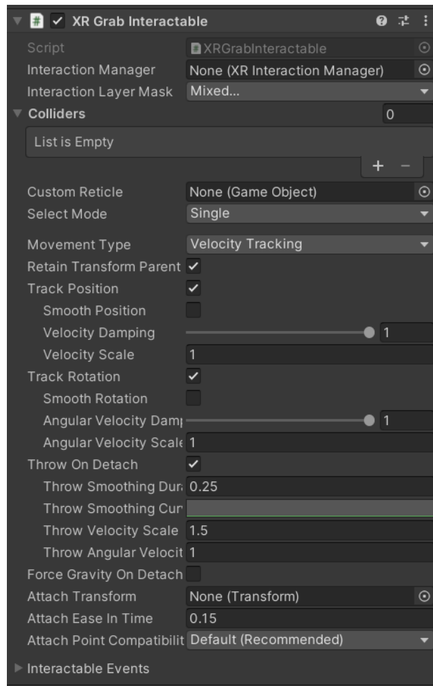
Figura 4.1: Componente Grab Interactable
