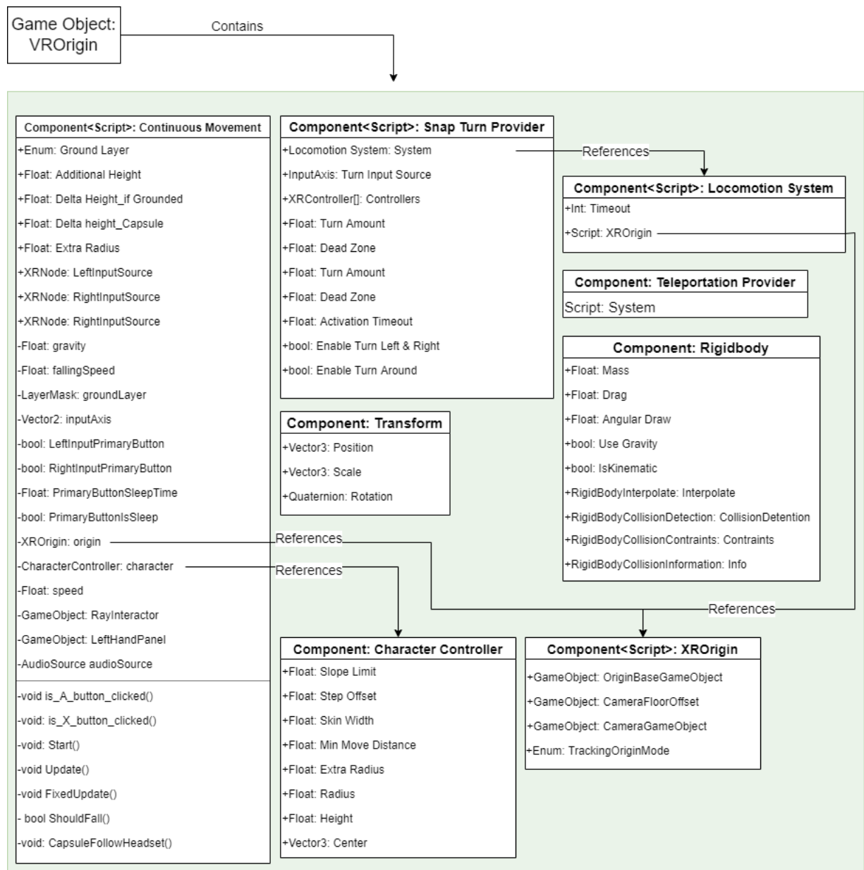
Figura 4.8: Diagrama Componentes agregados a VROrigin
